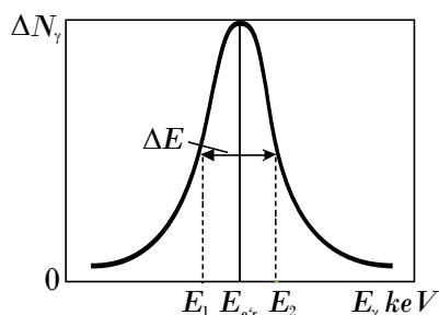
20-rasm. Yarimo'tkazgichli spektrometrning energiya bo'yicha ajrata olish qobiliyatini aniqlash.
