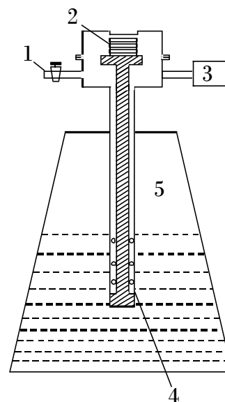
18-rasm. Yarimo‘tkazgichli detektorning umumiy ko‘rinishi: 1 – vakuum krani (VK); 2 – yarimo‘tkazgichli detektor (YaD); 3 – oldkuchaytirgich (OK); 4 – sorbent; 5 – dyuar idishi.
