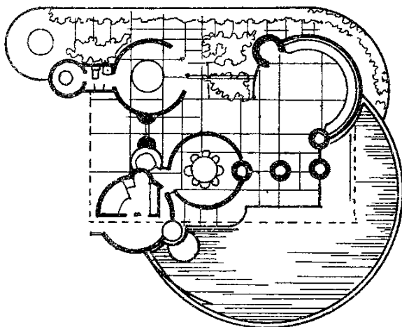
Джестер уйининг лойихаси (Ф.Райт)
