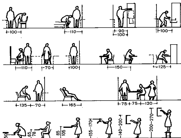
71 - расм. Турар-жой ячейкасининг фазовий ташкил
