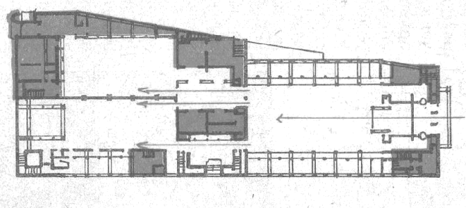
Пухта тузилган режавий структурали бино намунаси. Роттердамдаги биржа режаси.
