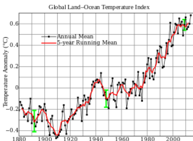
Рис. 256. Средние температуры поверхности Земли.
