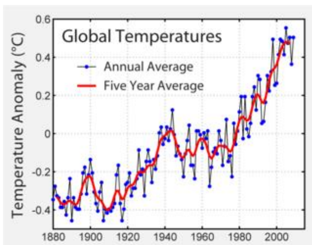
Рис.255. График температур по данным НАСА .
