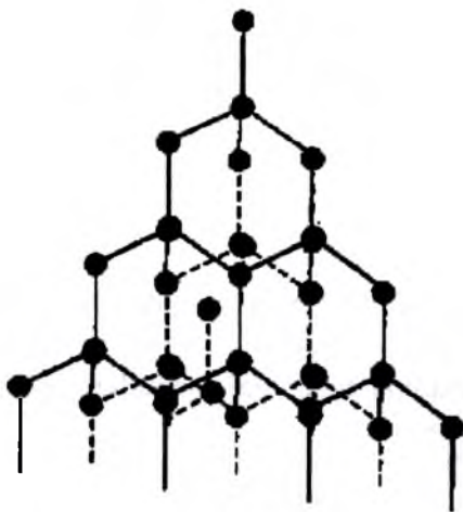
5-rasm. Olmosning kristall panjarasi.
