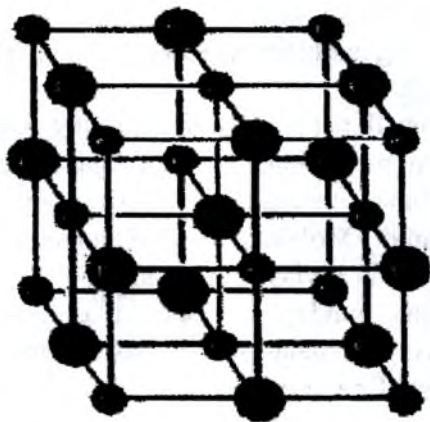
4-rasm. NaCl ning kristall panjarasi.
