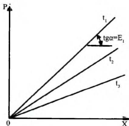
33-rasm. Absorbsiya hodisasining bosim va parsial bosim (yoki konsentratsiya)ga bog'liqligi.
