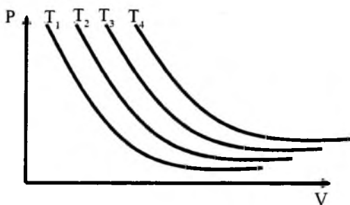
1-rasm. Ideal gazning izotermalari.
