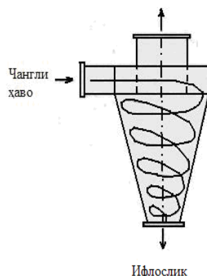
1-расм. Чанг ушлагичларнинг конструкцияси.
