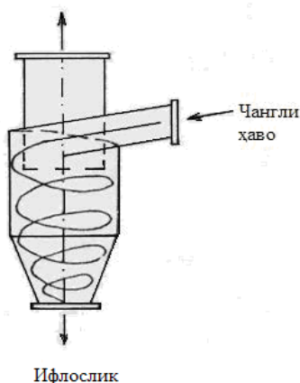
1-расм. Чанг ушлагичларнинг конструкцияси.
