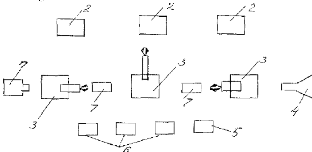
9.5-rasm. Sanoat Robotli avtomatlashtirilgan liniya struktura sxemasi.
