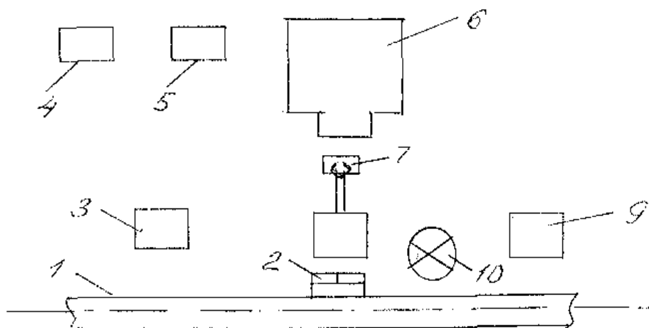
9.3-rasm. Sonli programmali boshqariladigan robototeknik bo'linmalarning struktura sxemasi.
