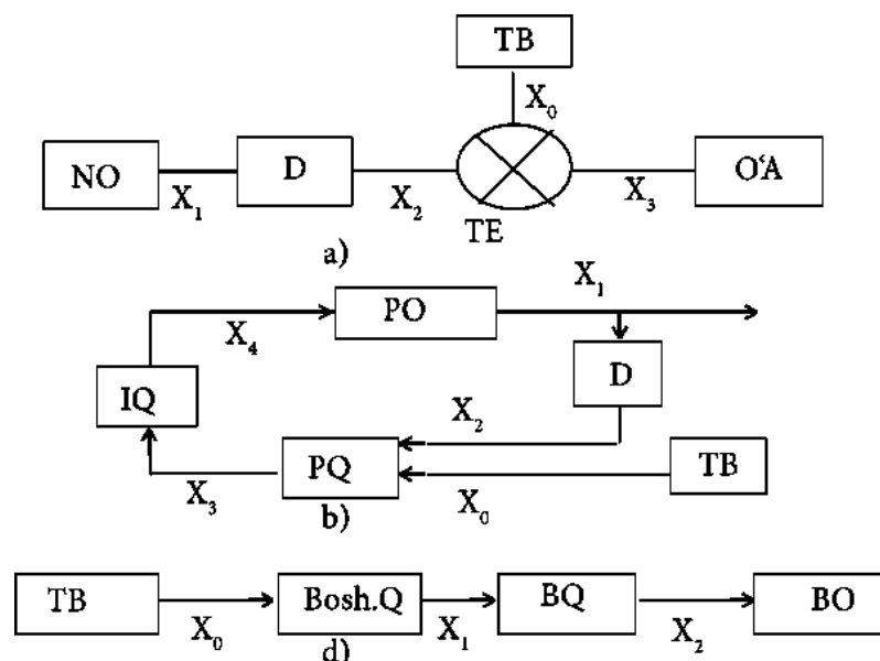
1. 1-rasm. Avtomatik sistemalarning funksional sxemalari. a) avtomatik nazorat sistemasi; b) avtomatik rostdash sistemasi; d) avtomatik boshqarish sistemasi.
