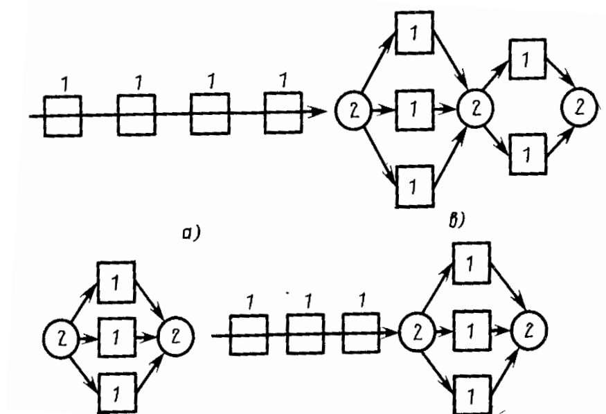
7.1-rasm: Avtomatik liniyalar strukturaviy sxemalari.
