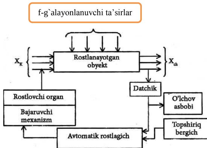
1.2-rasm. Bir konturli berk avtomatik rostdash sistemasining funksional sxemasi.
