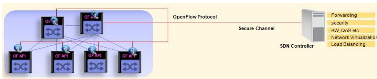
Рисунок 4. OpenFlow сетевая архитектура дата-центра
