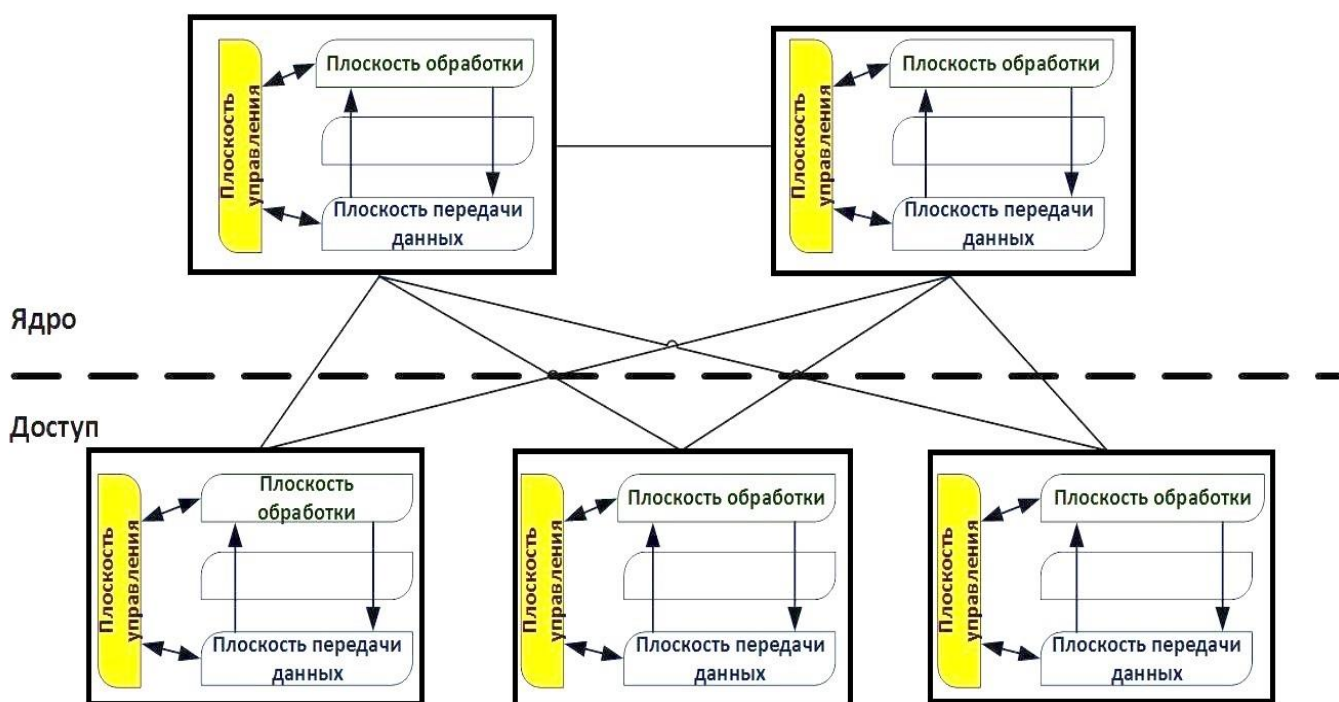
Рисунок 2. Самостоятельные плоскости обработки трафика
