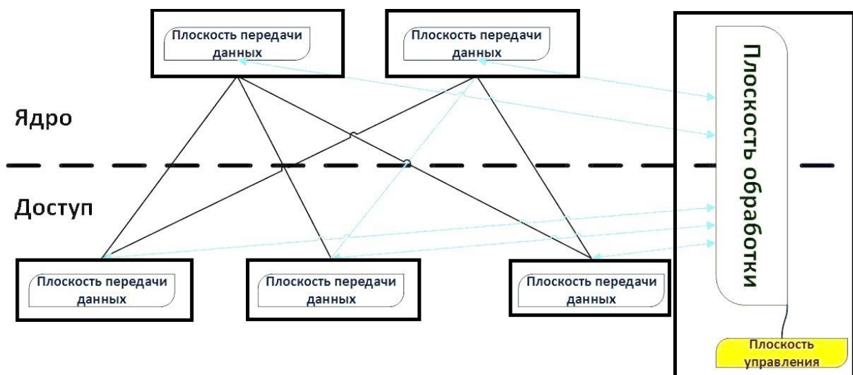
Рисунок 3. Централизованная плоскость обработки трафика
