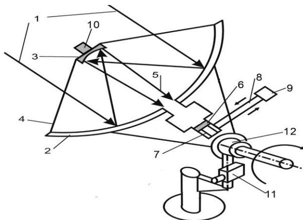
Рис.1. Общий вид гелиоэнергетической установки
