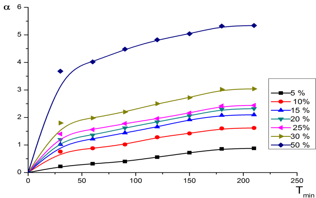
9-расм. АА:МБА чокланган сополимери бўқишининг сув миқдorigа боғлиқлиги. T=35^{\circ}\text{C} . 5,10,15,20,25,30 ва 50% сув миқдorigа, мос равишда 1,2,3,4,5,6 ва 7.
