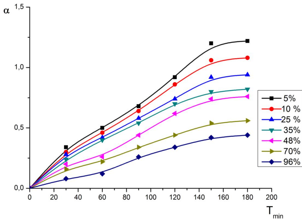
10 – расм. АА:МБА чокланган сополимери бўқишининг намуналар синтезида қўшилган этанол миқдorigа боғлиқлиги. T=25^{\circ}\text{C} .
