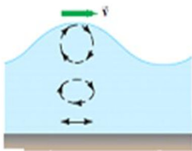
8.10-rasm. Uncha katta bo'lmagan suv to'qlini, ko'ndalang va bo'ylama to'qlinning birgalikda tarqalishiga misol bo'ladi.
