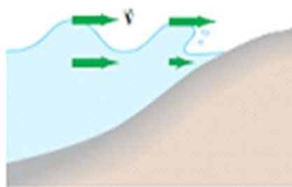
8.11-rasm. Suv to'qlinining shiddat bilan harakatlanishi. Yashil strelkalar suv molekulalarinig o'sha joydagi tezligini ko'rsatadi.
