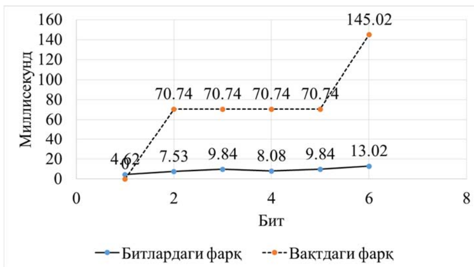
а) тезкор «пул» учун
