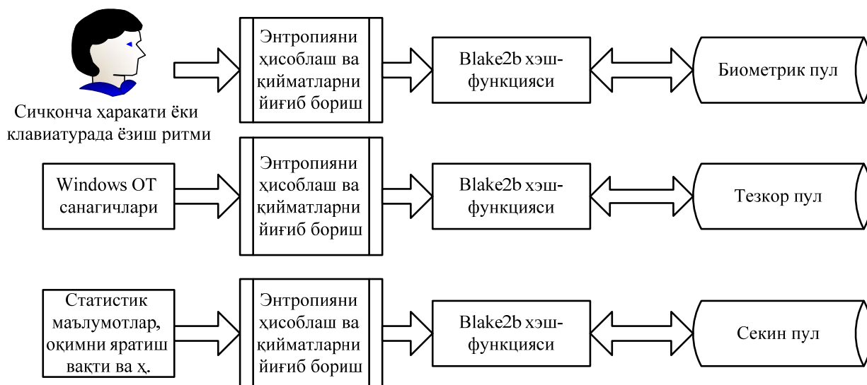
1-расм. Энтропияни ҳисоблаб тасодиғий қийматларни ажратилган «пул»ларга ёзиш
