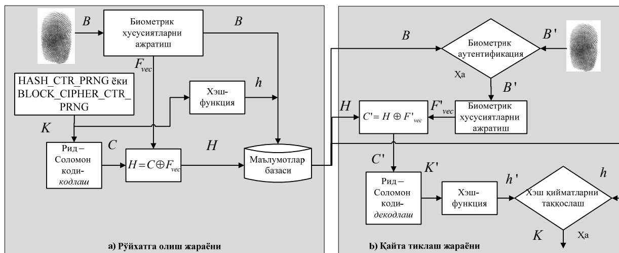
4-расм. Кристографик калитларни боғлаш усулининг функционал схемаси
