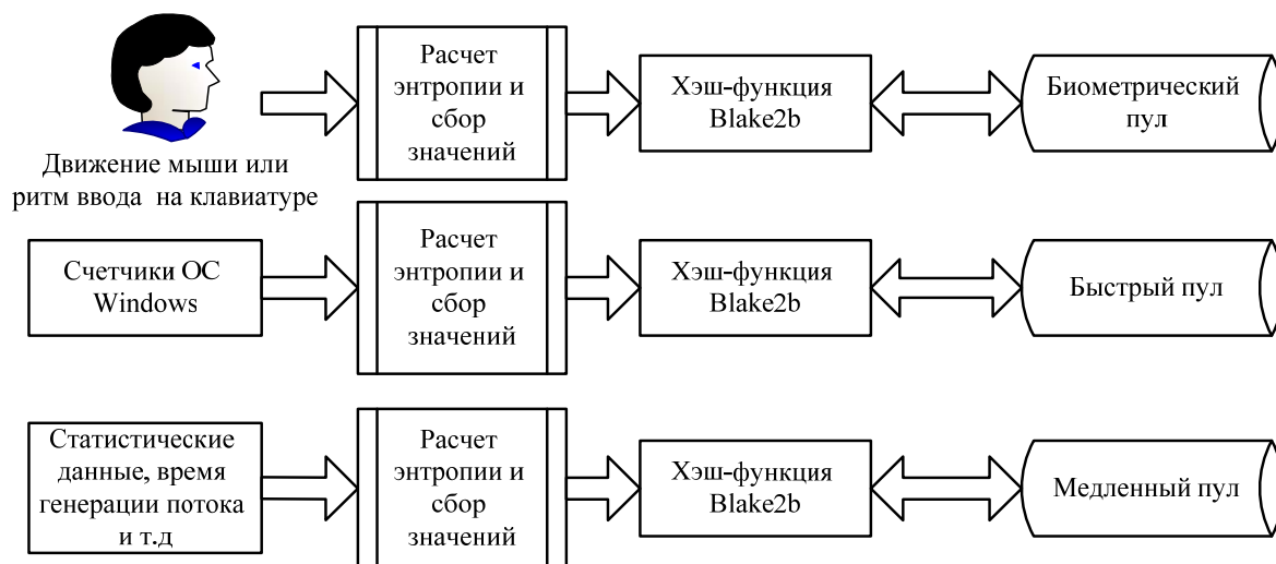
Рис. 1. Запись случайных величин с вычислением энтропии на выделенные «пулы»
