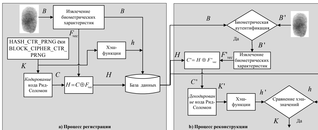
Рис. 4. Функциональная схема метода связывания криптографических ключей
