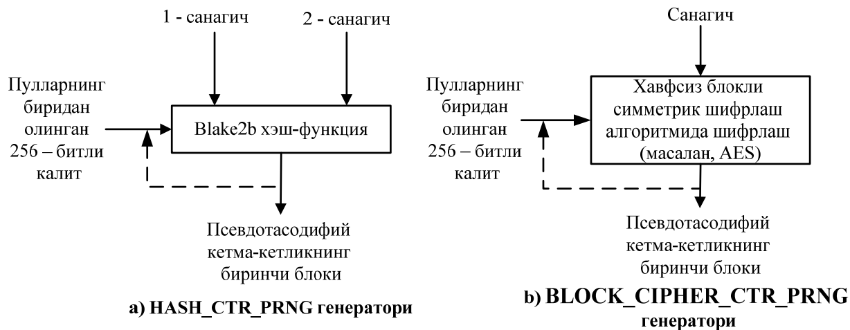
2-расм. Таклиф этилган псевдотасодиғий сонлар генераторларининг умумий кўриниши
