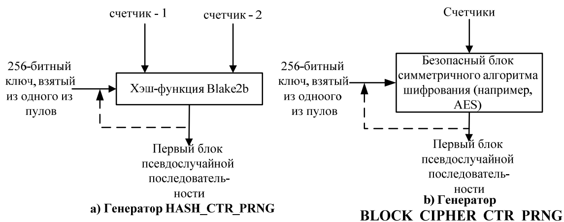
Рис. 2. Общий вид предложенного генератора псевдослучайных чисел
