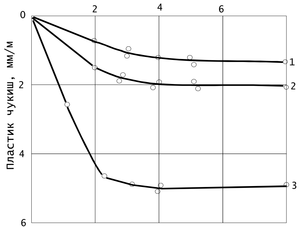
2-расм. Бетоннинг пластик чуқишининг бетон қотиш жараёнини тезлатиш усулига боғлиқлиги.
