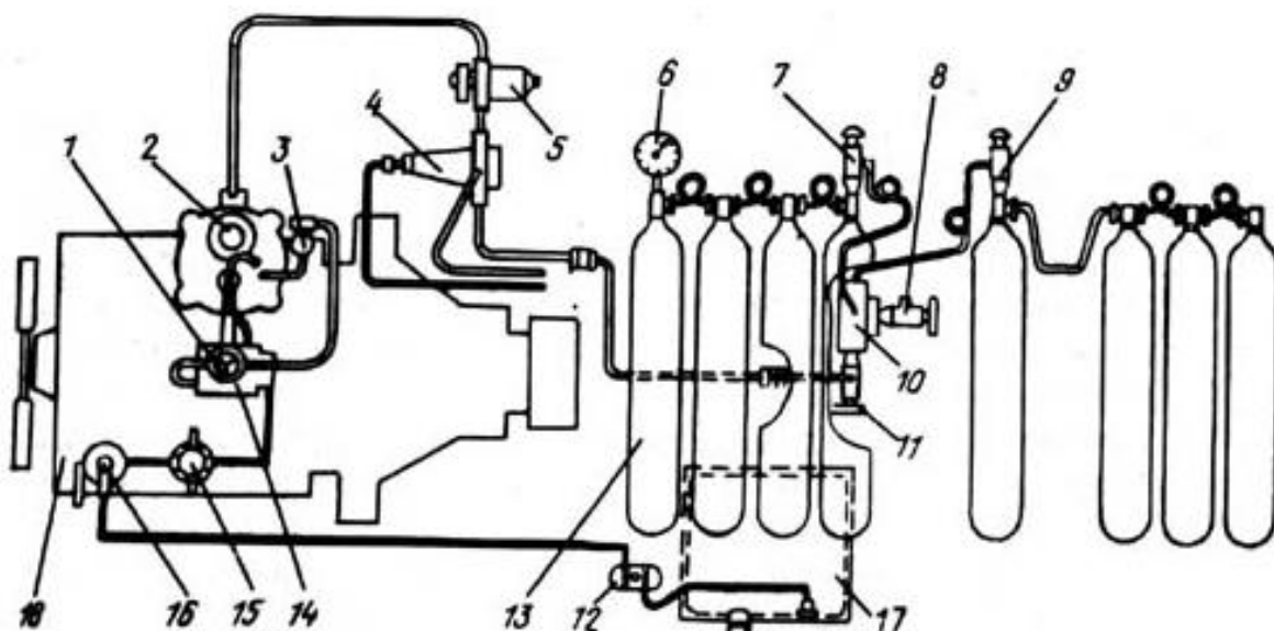
3.7-rasm. Yuqori bosimli gaz ballonda ishlovchi ZIL-43610 avtomobil dvigatelining gaz balonli ta`minot uskunasiining umumlashgan chizmasi.
