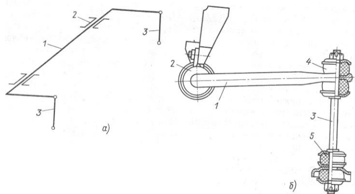
15.10-rasm. Ko'ndalang turg'unli stabilizatori: 1-P-simon shtanga, 2-rezinali vtulka, 3-ustunlar, 4 va 5-rezinali yostiqlar.
