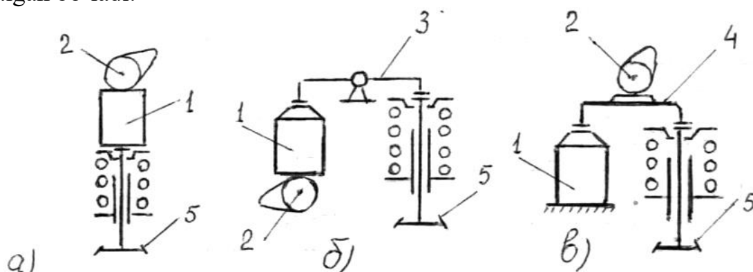
5.5-rasm. Hidrokompensatorni joylashtirish usullarining sxemalari:
