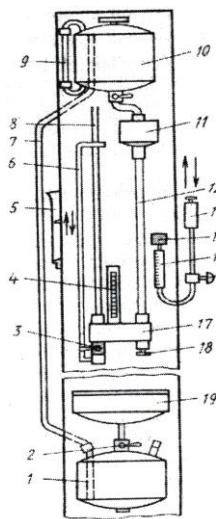
5.1-расм. Жиклёрнинг ўтказувчанлигини текширадиган НIIAT-528 русумли асбоб. Жиклёрни текшириш тартиби
