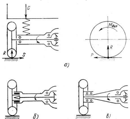
14.7-rasm. Yarim o'qlarning orqa ko'priklarda joylanish usullari
