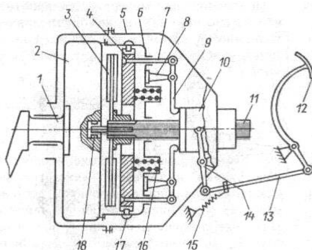
11.3- rasm. Bir diskli ilashish muftasi.
