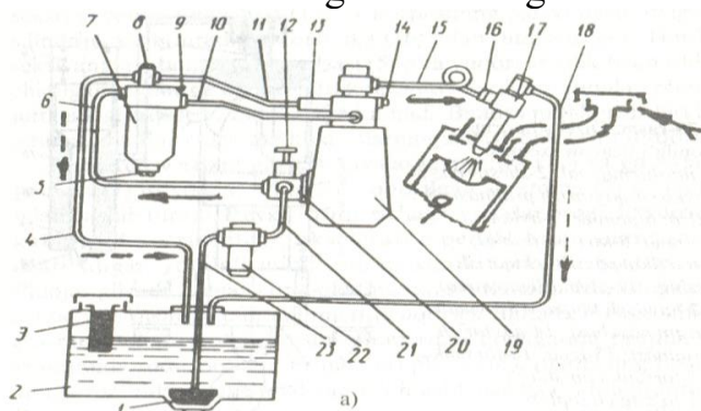
10.1-rasm. YaMZ dizelning yonilg'i bilan ta'minlash tizimi.
