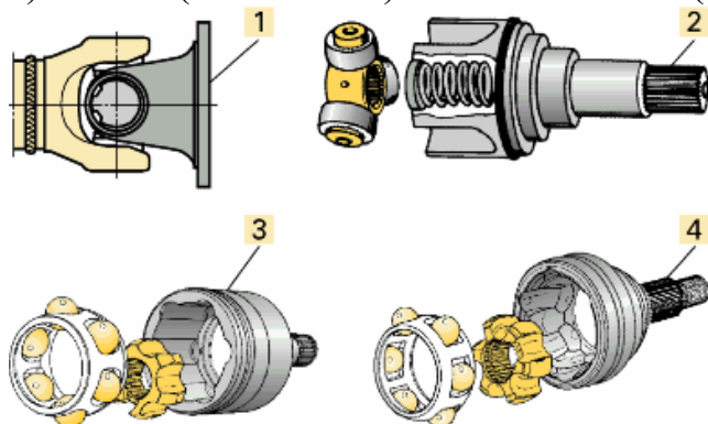
13.1-rasm. Kardanli uzatmaning konstruksiyasi
