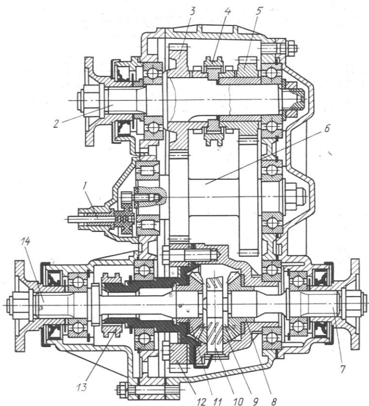
12.5-rasm. VAZ-2121 «Niva» avtomobilining taqsimlash qutisi: 1- spidometr yuritmasi; 2-etkachi val; 3-yuqori uzatma shesternyasi; 4-uzatmalarni qo'shish muftasi; 5-quyi uzatma shesternyasi; 6-oraliq val; 7-orqa ko'prikn yuritmasi vali; 8 va 11-differentsial shesternyasi; 9-differentsial satelliti; 10-satellit o'qi; 12-differentsial korpusi tishli g'ildiragi; 13-differentsial blokirovkasi muftasi; 14-old ko'prikn yuritmasi vali.
