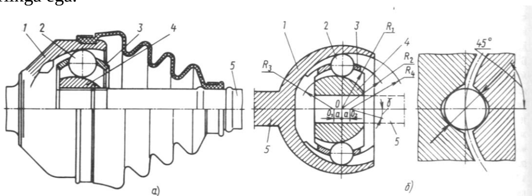
13.4-rasm. (Birfilbd turidagi) Olti sharikli kardan sharniri:
