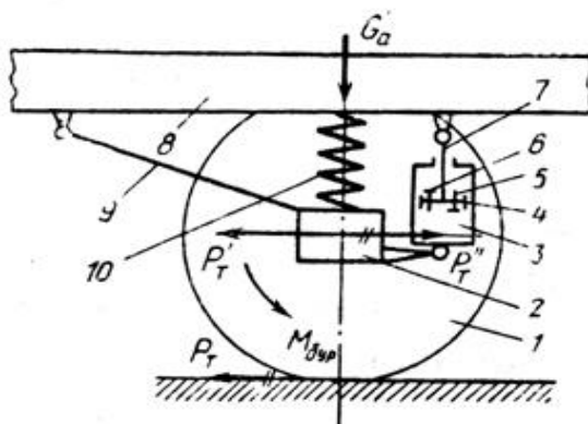
6.2-rasm. Avtomobil osmasini tasviriy chizmasi.
