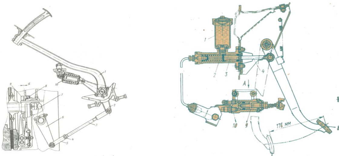
11.6-rasm ilashish muftasining boshqarish yuritmalari. a- mexaniq boshqarish yuritmasi; b-gidromexanik boshqarish yuritmasi;
