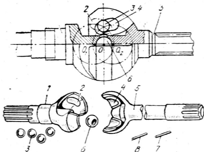
13.3 -rasm. Bir xil burchak tezlikli sharchali kardan sharniri: 1 va 5 –yarim o'qlar; 2 va 4-ariqchalar; 3- yetakchi sharchalar; 6- markaziy sharcha; 7 va 8 -shpilka;
