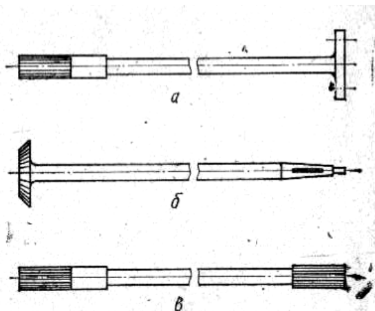
14.6-rasm. Avtomobillarning yarim o'qlari
