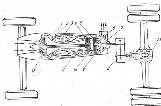
3.9-rasm. Gaz trubinali dvigatel o'rnatilgan avtomobilning oddiy sxemasi:
