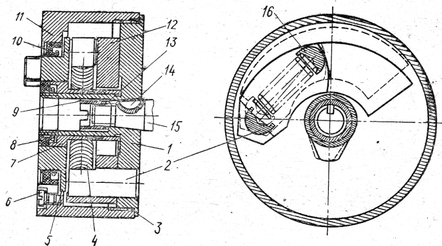
10.6-rasm. Yonilg'ini ilgariyatib purkovchi avtomatik mufta.
