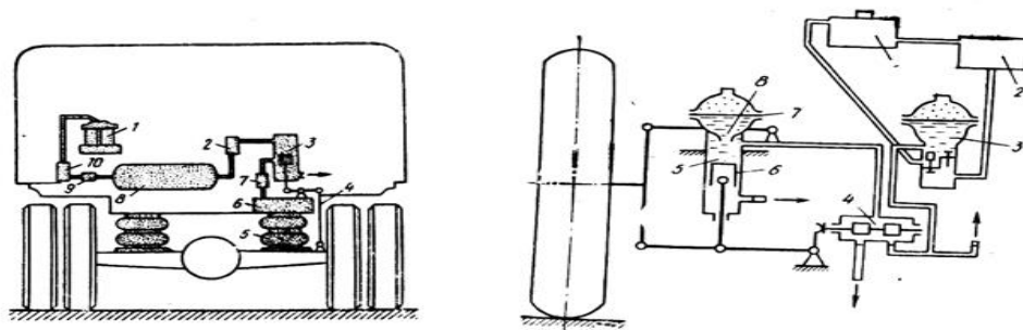
6.3-rasm. Pnevmatik va gidropnevmatik osmasining tasviriy chizmasi.
