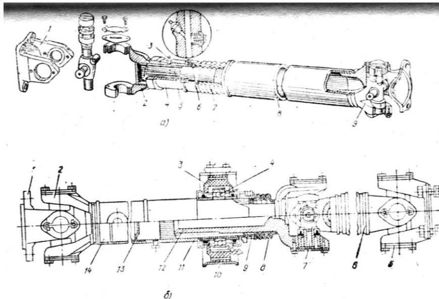
13.5-rasm. Avtomobillarning kardanli uzatmasi:
