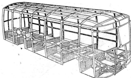
15.4-rasm. Avtobusning karkasli vagon tipidagi kuzovi.
