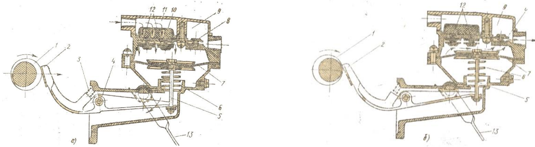
8.2-rasm. Diafragma turidagi yonilg'i nasosi.
