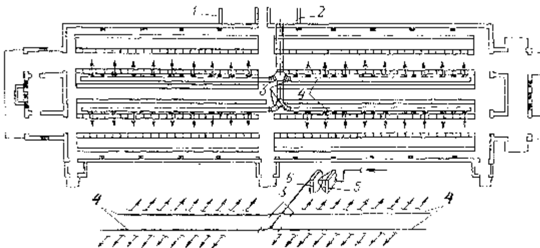
2.1-su'wret. 60 bas qaramal ushin malxanadag'ı (№ 801-70 n.l.) mexanik aydaw sisteması sxeması:
