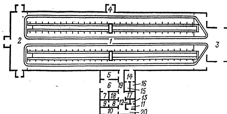
1.2-su'wret. 20 bas sıyırdı baylap bag'ıw usılına mo'lsherlengen sıyırxana jobası:
