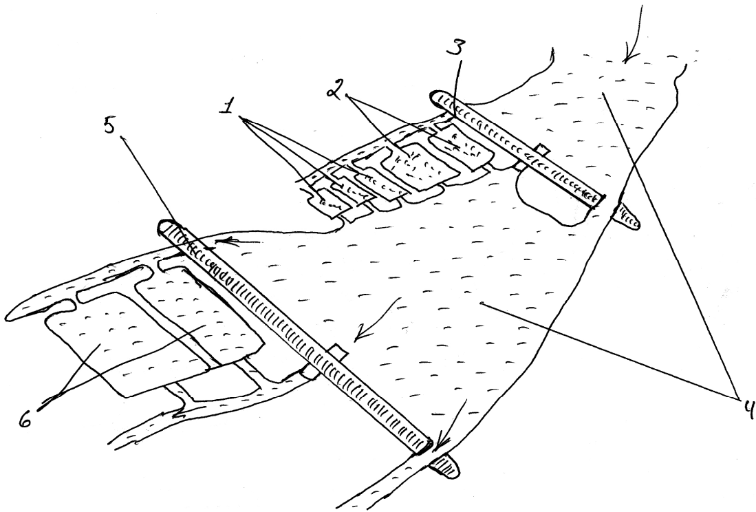
Apiwayı ha'm toliq sistemadag'ı ha'wizlerdin' du'ziliw kestesi (sxemasın) joybarlaw
