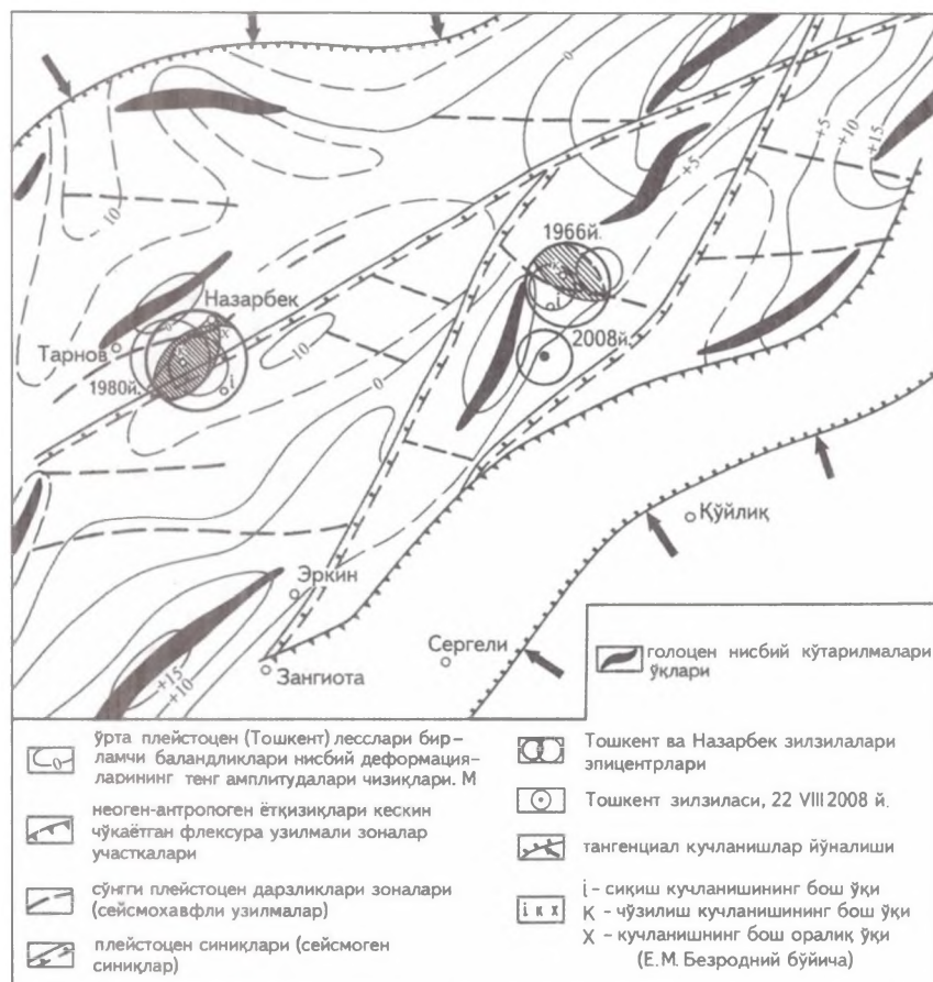
Тошкент ва унга туташ туманларнинг сейсмотектоник харитаси.
