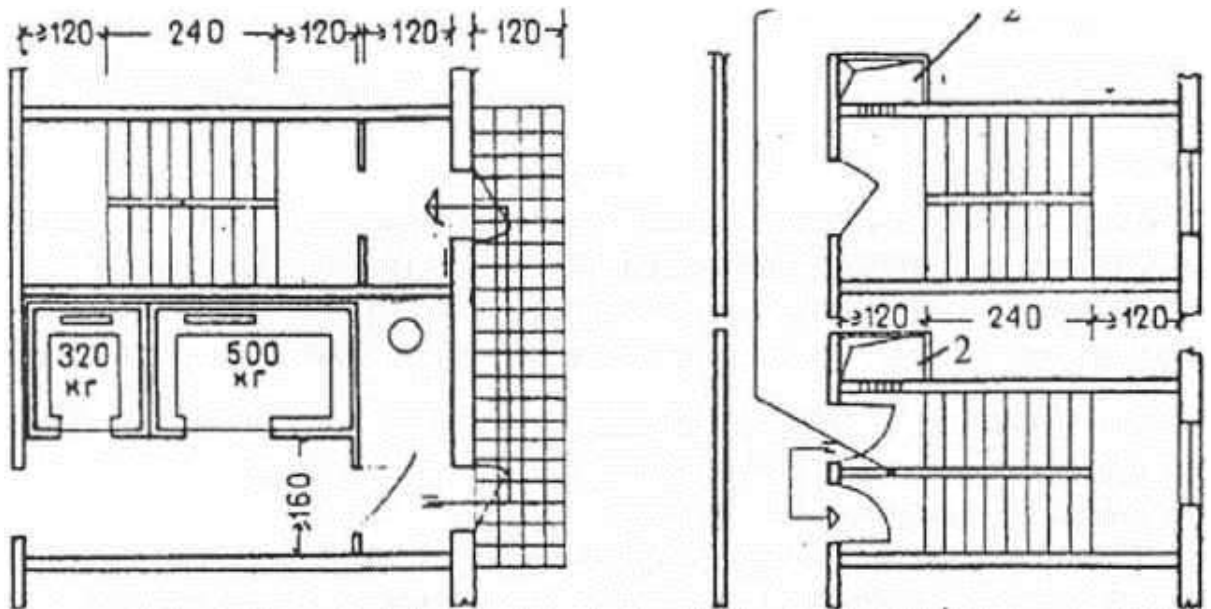
5-расм. Тутун қирмайдиган зинахоналарнинг типлари:
