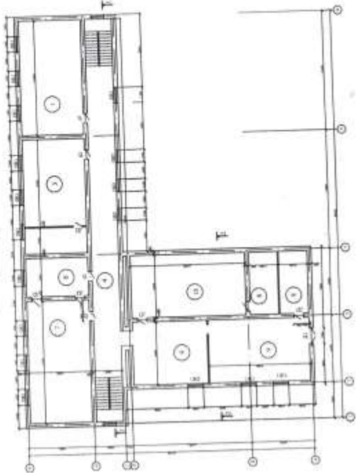
2-Қават режаси.
