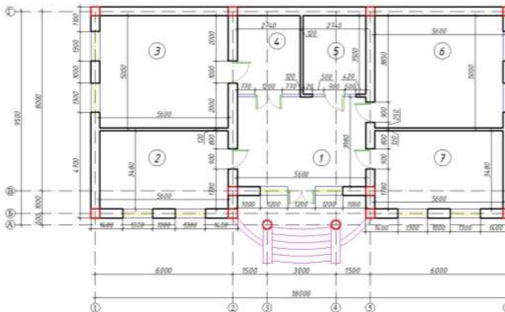
Бино режаси
