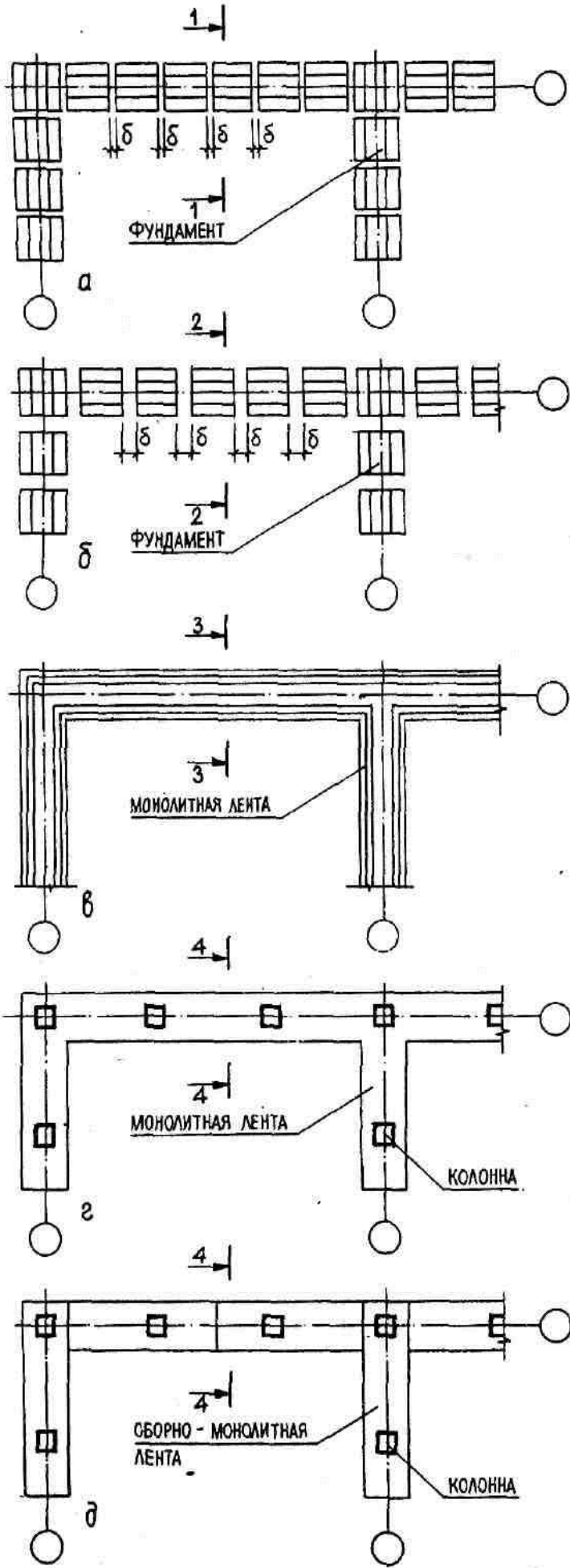
10-рasm..Лентасимон йиґма-бетон блок ва устунсимон монолит пойдевор.
