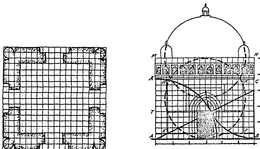
11-расм. Бухородаги Сомоний мақбарисининг меъморий лойиҳаланиш услублари. Тархи ва тарзи.
