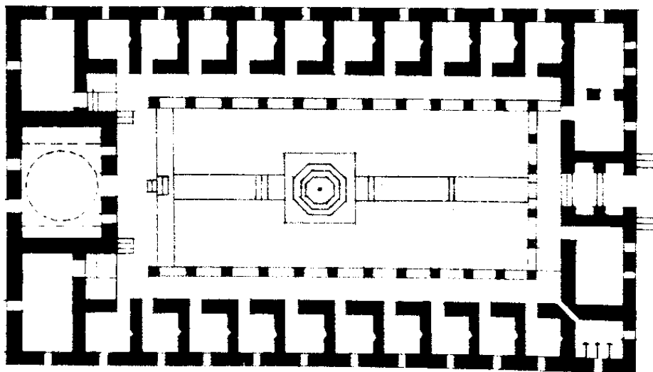
7-расм. Туркиянинг Бурса шаҳрида XV асрда Йилдин Боязид томонидан қурилган шифохонанинг тархи ва қирқими.
