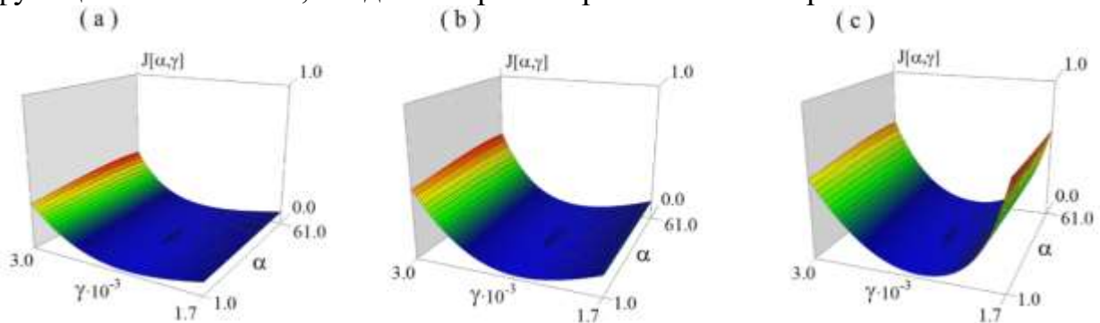
Рисунок 2. Примеры поведения функционала невязки при использовании различных интервалов временных частот, а) f_0 \in [5; 25] Гц, б) f_0 \in [5; 50] Гц, в) f_0 \in [5; 75] Гц.
