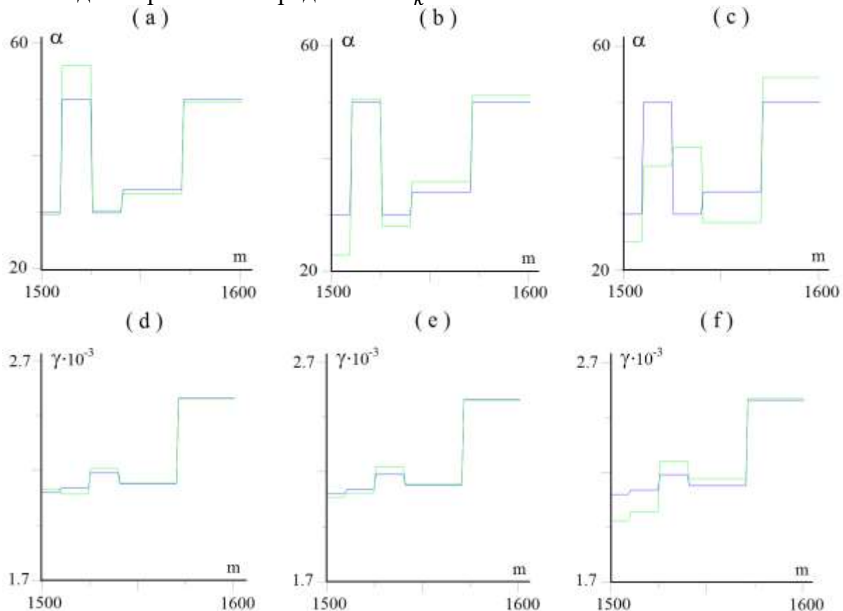
Рисунок 3. Примеры восстановления параметров а)-с) \alpha , d)-f) \gamma ; примеры восстановления с ошибкой в данных обратной задачи а), d) 3%, б), е) 5% и с), f) 10%. Точное значение указано синей линией, восстановленное – зелёной.
