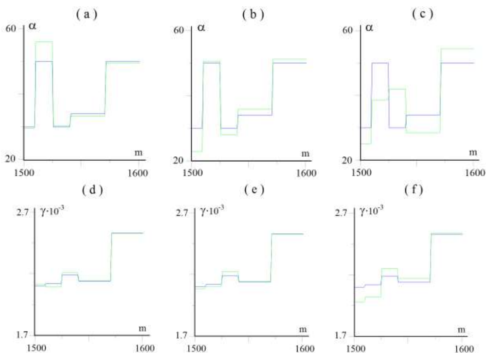
3-расм. Параметрларнинг тикланиш натижалари а)-с) \alpha , d)-f) \gamma ; тескари масала берилганларига хатолик қўшиб параметрларни тиклаш а), d) 3%, b), e) 5% ва с), f) 10%.
