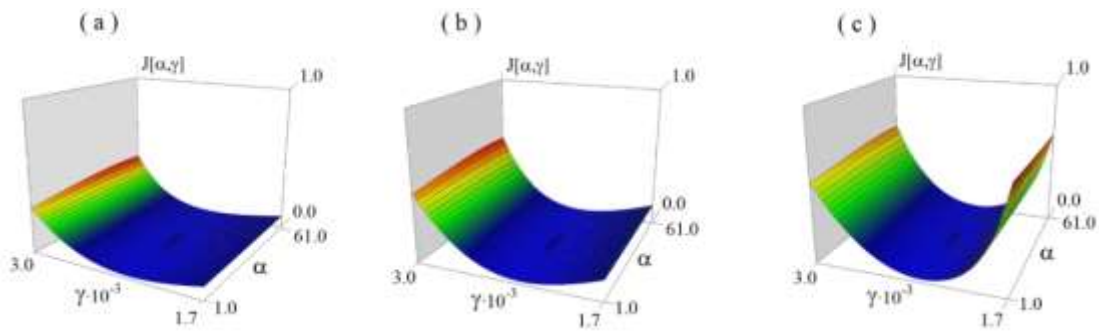
2-расм. Частотанинг турли интерваллари танланганда, қолдиқ функционали ўзгариши, а) f_0 \in [5; 25] Гц, б) f_0 \in [5; 50] Гц, в) f_0 \in [5; 75] Гц.
