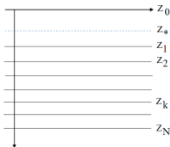
1-расм. Муҳит модели.
