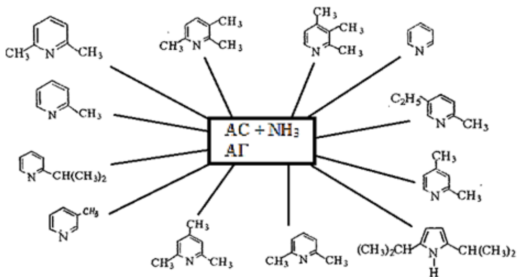
Рис.2. Общая схема синтеза пиридиновых оснований и производных пиррола на основе АС, АГ и аммиака
