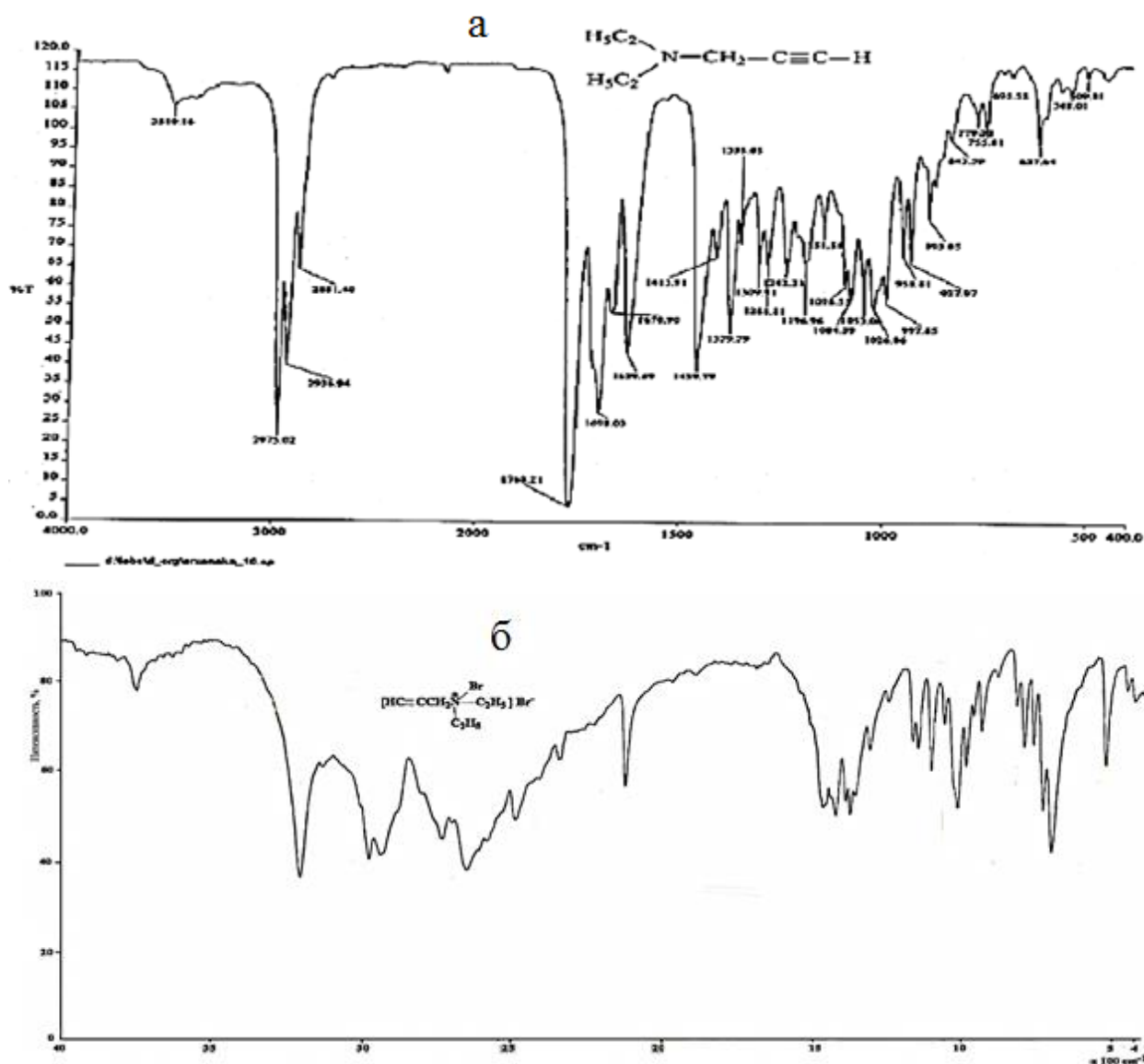
1-Расм. 1-Диэтиламинопропин-2 (а) ва унинг дибромаммонийли тузи (б) ИҚ-спектрлари.
