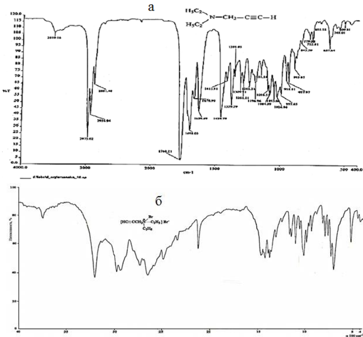
Рис.1. ИК-спектры 1-Диэтиламинопропина-2 (а) и его диброаммониевой соли (б).
