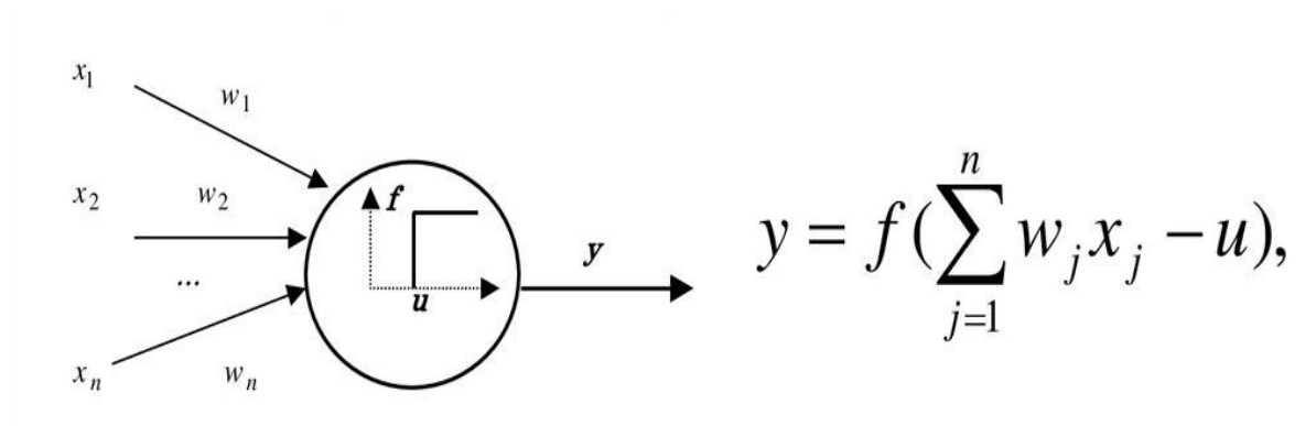
12-расм. Сунъий - математик нейрон модели:
