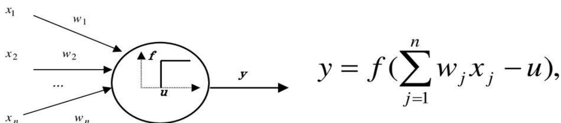
Рисунок 12. Искусственно-математическая модель нейрона:
