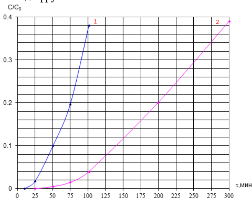
Рис.1. Динамика насыщения фруктов хлором.
