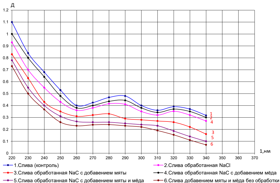
Рис.5. УФ-спектры образцов сливы.
