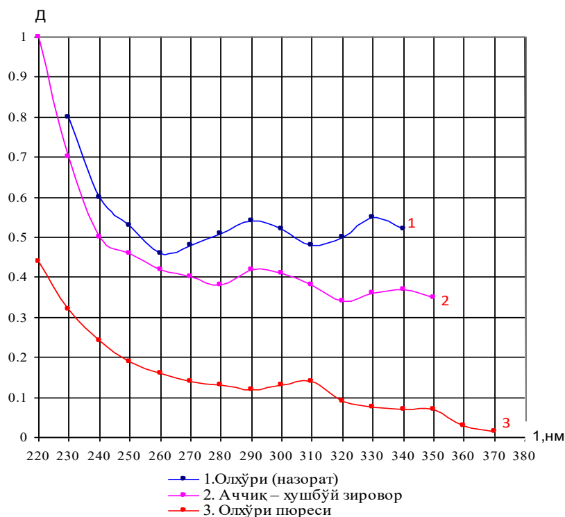
7-расм. Аччиқ-хушбўй қайлада УВ спектрли нурларнинг ютилиши.
