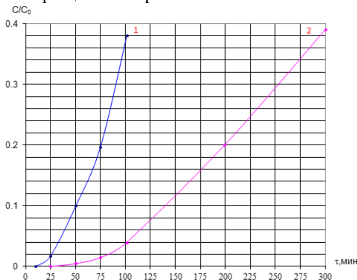
1-расм. Меваларнинг хлор билан тўйиниши динамикаси.
