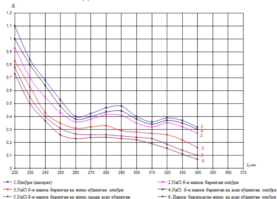
5-расм. Олхўри намуналарининг УБ спектрлари.
