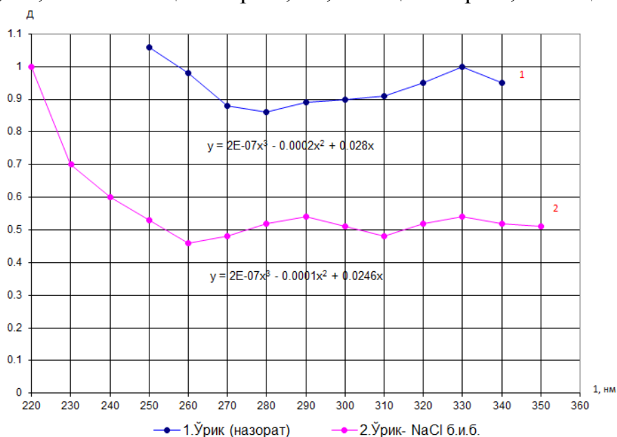
4-расм. Олхўри намуналарини УБ ютиш спектрлари.
