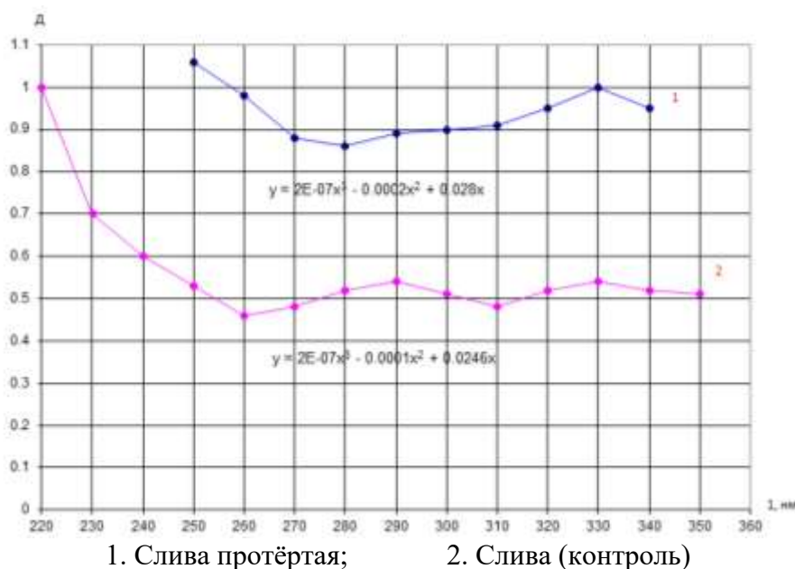
Рис.4. Спектры поглощения УФ лучей образцов сливы.
