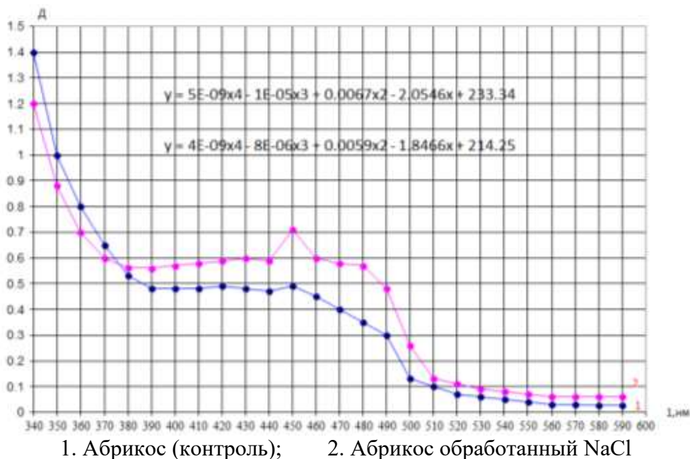
Рис.3. Спектры поглощения образцов в видимой области спиртовых экстрактов образцов плодов абрикосов до и после обработки NaCl.
