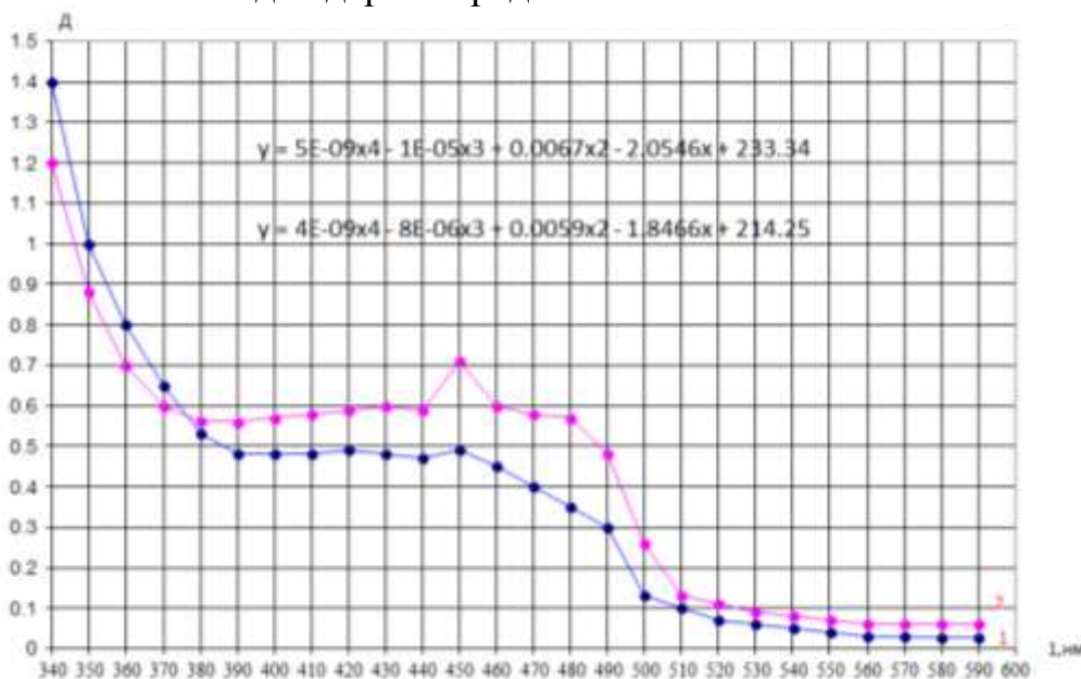
3-расм. Ўрик намунасини спиртли экстрактларининг кўриниш соҳасидаги NaCl билан ишлов беришгача ва ишлов беришдан кейинги ютилувчи спектрлари.
