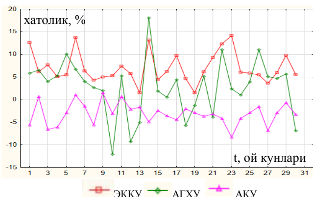
13-расм. “WBM ROMITEX” МЧЖ пахта тўқимачилик кластери корхонаси электр энергияси истеъмолининг хақиқий ва прогноз кўрсаткичлари орасидаги прогноз хатолиги графиги
