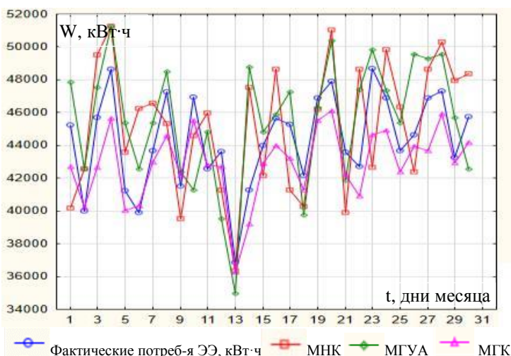
Рисунок 12. График сравнения результатов прогнозирования потребления электроэнергии хлопко-текстильно-кластерного предприятия ООО «WBM ROMITEX» с использованием MNK, MGA, MGK
