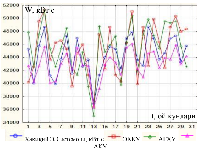
12-расм. “WBM ROMITEX” МЧЖ ПТК корхонасида ЭЭ истеъмолини прогноз қилишда қўлланилган ЭККУ, АГХУ ва АКУ натижаларини таққослаш графиги
