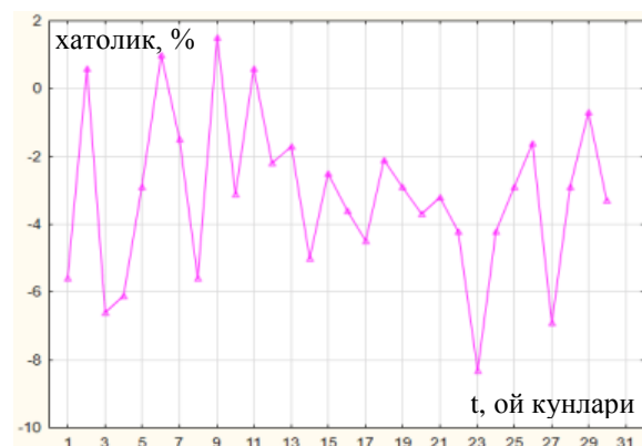
11-расм. “WBM ROMITEX” МЧЖ ПТК корхонаси ЭЭ истеъмолнинг хақиқий ва прогноз кўрсаткичлари орасидаги хатолик кўрсаткичлари графиги (2019 йил сентябр)
