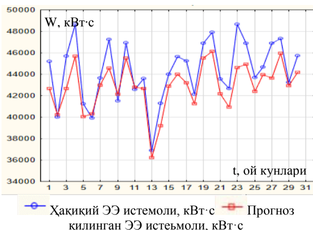
10-расм. “WBM ROMITEX” МЧЖ ПТК корхонаси ЭЭ истеъмолнинг хақиқий ва прогноз кўрсаткичлари (2019 йил сентябр)
