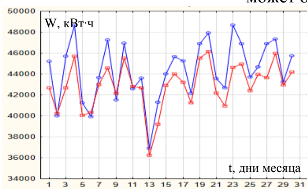
— Фактические потребления ЭЭ, кВт·ч; — Прогнозные потребления ЭЭ, кВт·ч.
