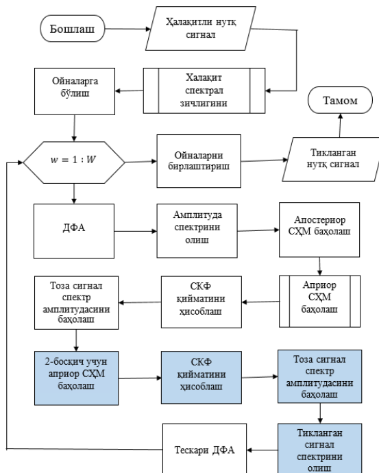
7-расм. Халақитни камайтириш икки босқичли алгоритми блок схемаси
