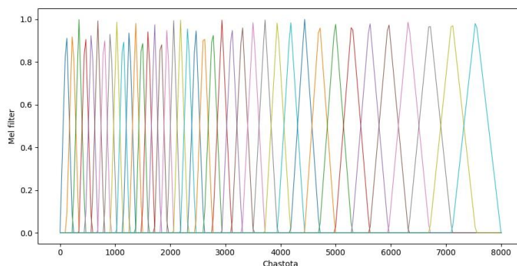
3-расм. Q=24 мел-фильтрларнинг АЧХси
