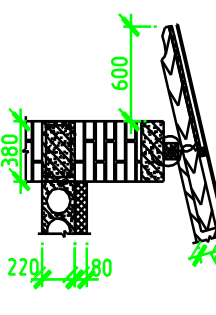
Luqun "2" M 1:20
