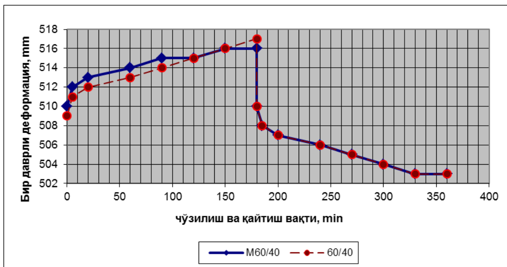
4-расм. M60/40 (60%и модификацияланган нитрон, 40%и пахта тола) ва 60/40 (60%и нитрон, 40%и пахта тола) намуна ипларнинг бир даврли деформацияси.
