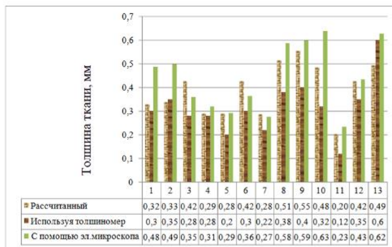
Рисунок 5. Сравнительная диаграмма толщина ткани, определенных 3 различными способами
