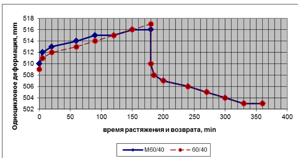
Рисунок 4. Одноцикловая деформация образцов пряжи M60/40 (60% модифицированной нитрон, 40% хлопковой волокна) и 60/40 (60% нитрон, 40% хлопковой волокна).
