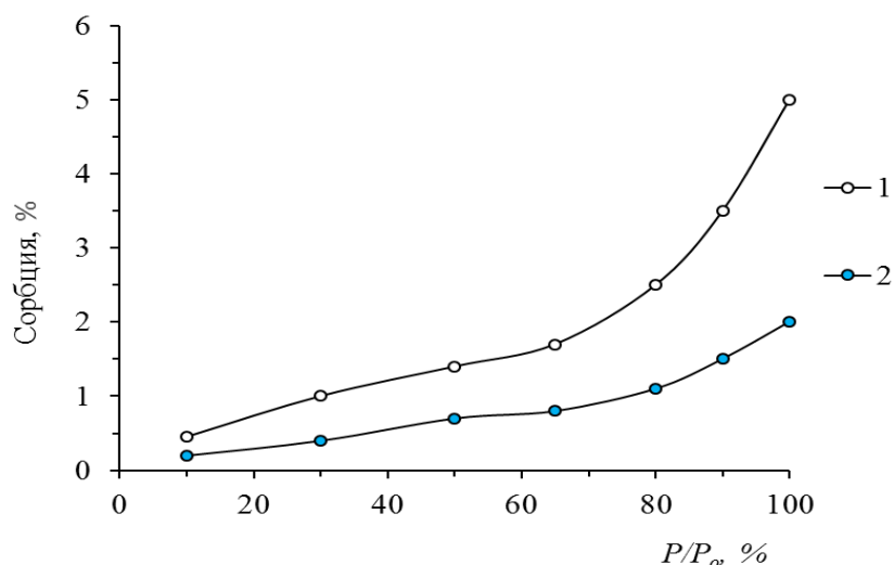
7-расм. Фиброин микротолали нотўқима материалларнинг сув бугларини сорбциялаши: 1 –микротолали, \beta \approx 0,5 ; 2 –микротолали, \beta \approx 0,8 .
