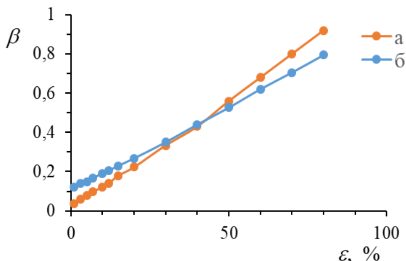
6-расм. Ориентация факторини ( \beta ) нисбий узайишга ( \epsilon ) боғлиқлиги: а – ФБ микротолали материал; б – ФБ нанотолали материал.
