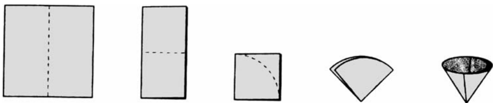
Рис. 12. Приготовление фильтра
