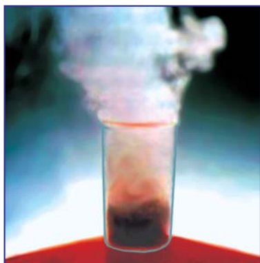
Рис. 19. Разложение \text{H}_2\text{O}_2 в присутствии \text{MnO}_2
