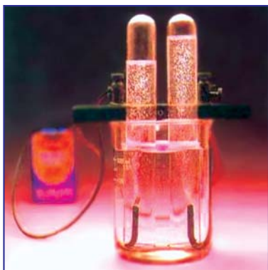
Рис. 18. При электролизе воды образуется один объем кислорода и два объема водорода.
