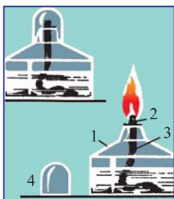
Рис. 4. Спиртовая лампа
