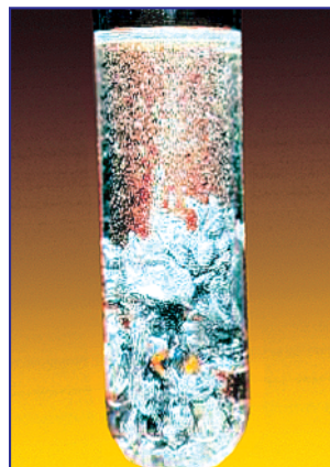
Рис. 25. Вытеснение водорода цинком из соляной кислоты
