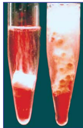
Рис. 50. Воздействие соляной кислоты на мел
