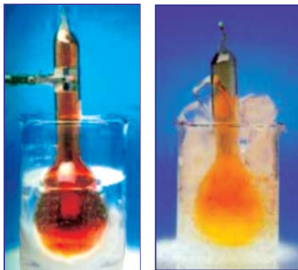
Рис. 39. NO 2 в газообразном и охлажденном виде
