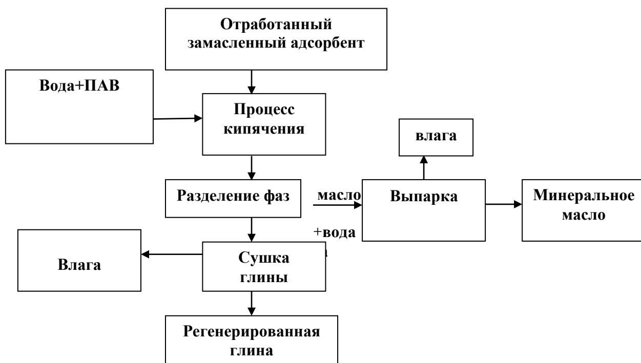
Рис. 1. Схема извлечения минеральных масел из отработанных глинистых адсорбентов
