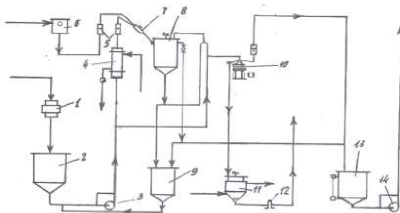
Рис. 3 Технологическая схема разделения минерального масла и парафина из отработанных глинистых адсорбентов с использованием центробежного аппарата
