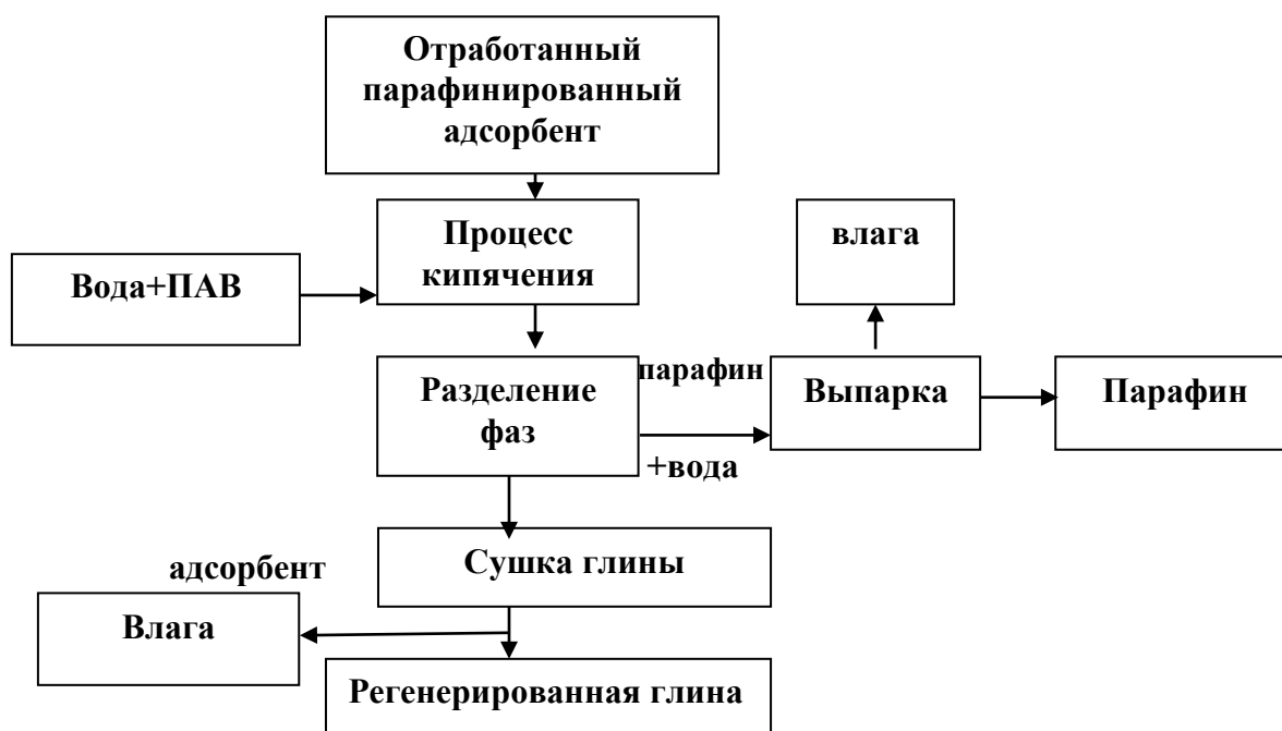
Рис. 2. Схема извлечения парафина из отработанных глинистых адсорбентов
