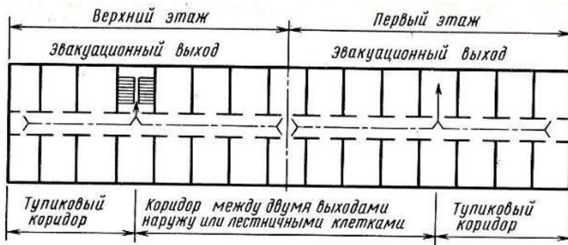
Чизма 17. Эвакуация йўллари таркибий қисмлари
