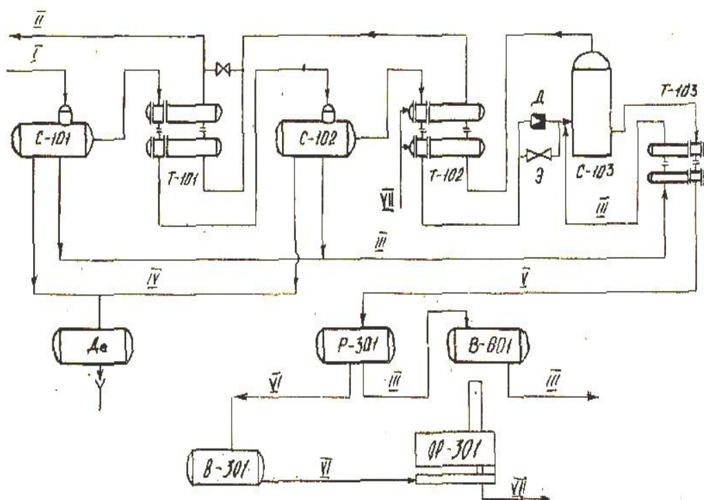
Рис.2.2. Принципиальная технологическая схема НТС УКПГ месторождения Шуртан:
