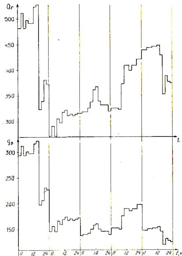
Рис.2.3. Динамика загрузки УКПГ месторождения Шуртан по зависимости от времени минимально возможного количества капельной влаги, поступающей в низкотемпературный сепаратор С-103
