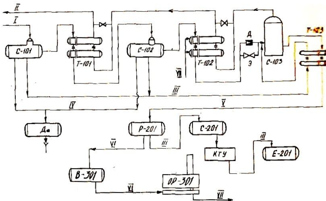
Рис.2.1. Принципиальная технологическая схема НТС УКПГ месторождения Зеварды:
