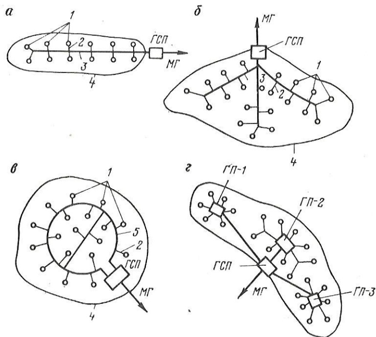
Рис. 1.1. Схемы промышленного сбора газа и конденсата:
