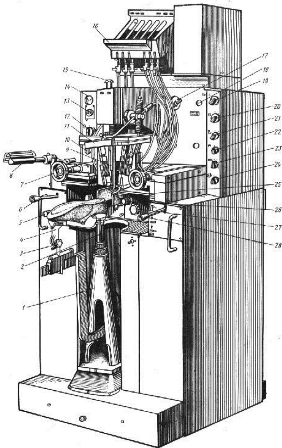
67-rasm.02146/R2 yarim avtomati.
