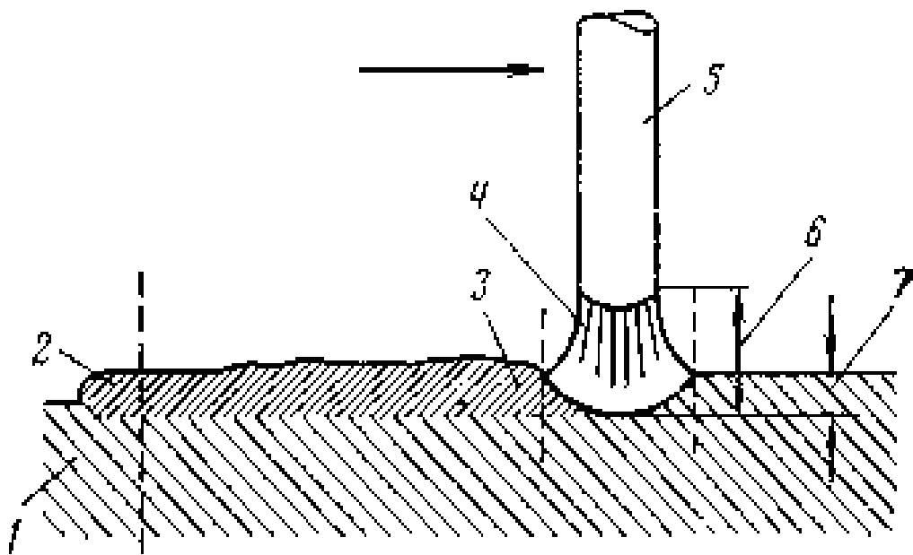
32-rasm. Suyultirib qoplash jarayoni sxemasi.
