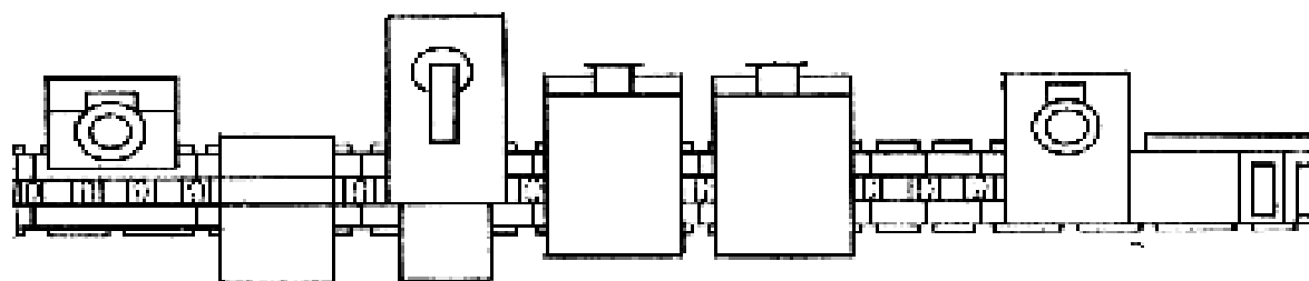
69--rasm. PLK-3-0 yarimavtomatik qatori.
