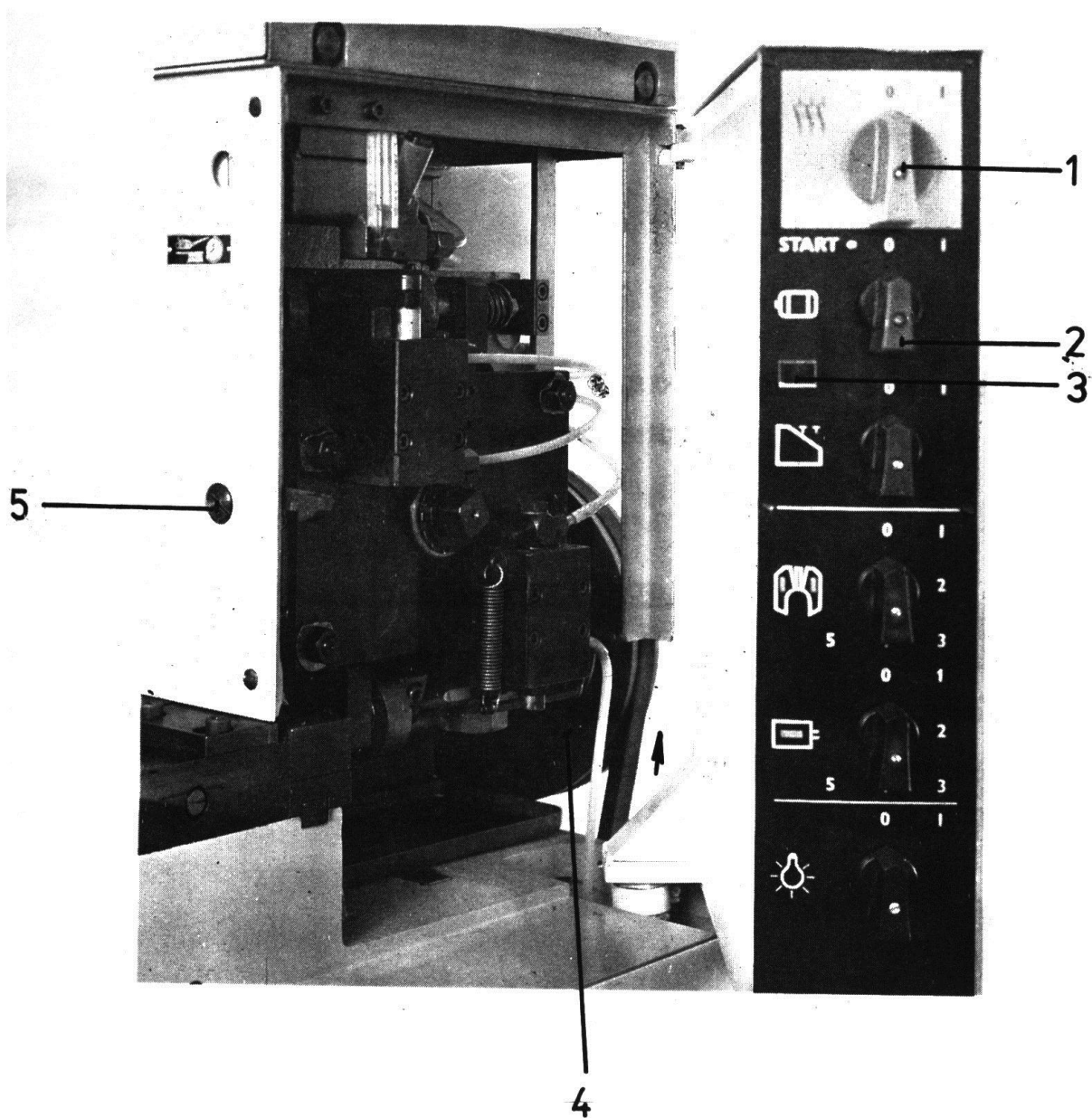
66–rasm. a) Mashinani boshqarish pulti.
