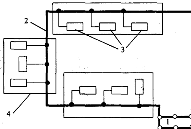
Рис. 20.4. Схема выносного заземления: 1 – заземлители; 2 – заземляющие проводники; 3 – заземляемое оборудование; 4 – производственные здания
