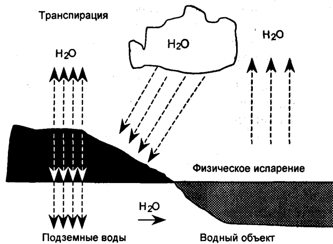
Рис. 1.3. Круговорот воды [21]
