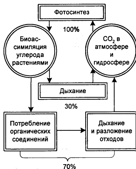
Рис. 1.2. Круговорот углерода [21]
