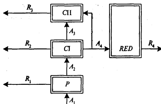
Рис. 6.1. Схема потоков энергии через четырехуровневую экосистему: P – продуценты, C1 – консументы 1 порядка, CII – консументы второго порядка, RED – редуценты, A_k и R_k - входящие и исходящие потоки энергии для k -го трофического уровня соответственно ( k = 1, 2, \dots )
