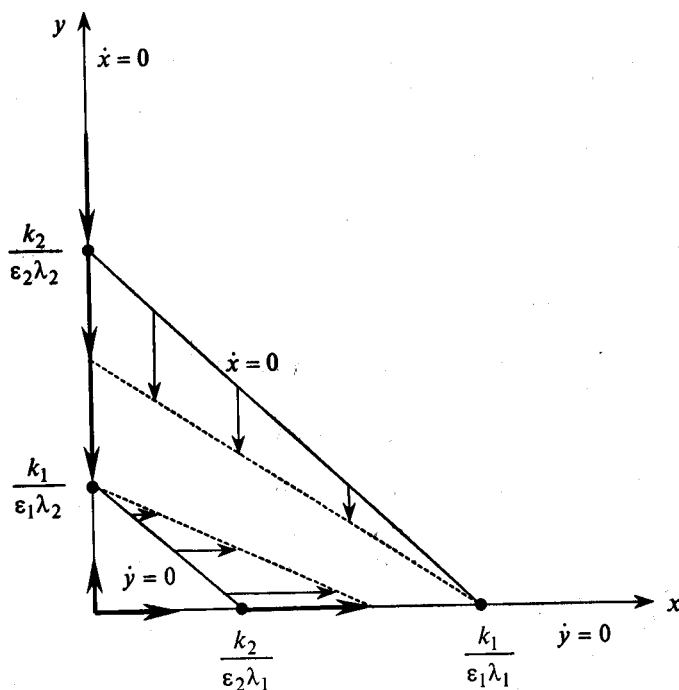
Рис. 9.2. Фазовый портрет динамической системы (9.10)
