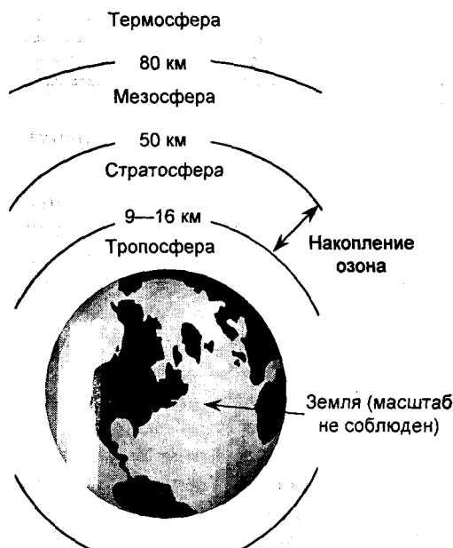
Рис. 4.3. Строение атмосферы
