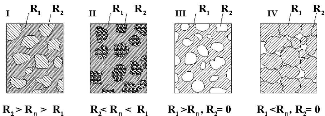
8.4 – расм. Бетон микротузилишининг асосий турлари. I - зич; II - зич ғовак тўлдирувчили; III - ковакли; IV - донадор; R_0 - бетон тузилишининг ўртача мустаҳкамлиги; R_1 ва R_2 - бетон таркибини ташкил этувчиларнинг мустаҳкамлиги.
