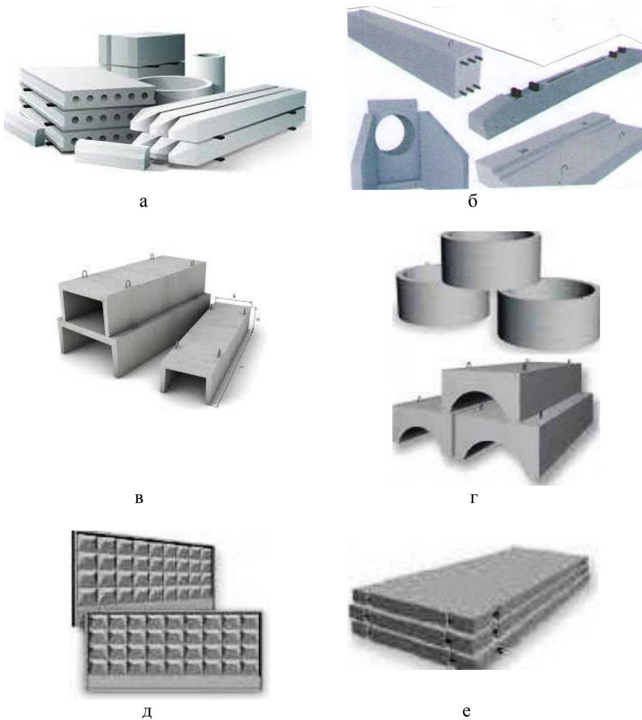
9.7 – расм. Муҳандислик бино ва иншоотлар конструкциялари. а-турли мақсадлар учун мўлжалланган буюмлар; б-йўл ва кўприк конструкциялари; в-лоток-ариқлар; г-сув ўтказиш буюмлари; д-тўсиқ девор панеллари; е-йўл ва канал плиталари.
