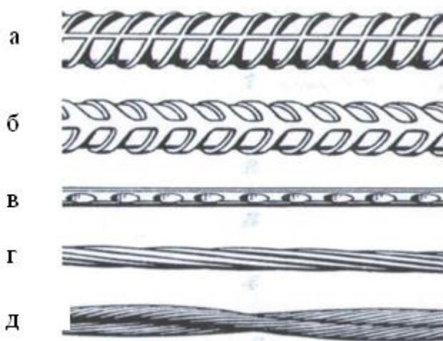
9.2 – расм. Пўлат арматура турлари. а-даврий профилли (резбасимон); б-худди шундай (арчасимон); в, г-юқори мустаҳкам симли; д-арқон арматуралар
