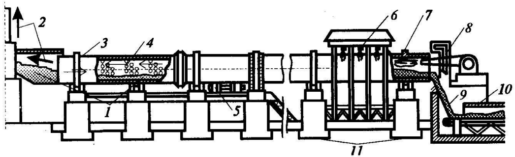
7.4 – расм. Айланма хумдон схемаси. 1 – хом ашё аралашмаси; 2 – иссиқ газлар; 3 – айланма хумдон; 4 – иссиқ алмашишини барқарорловчи мослама; 5 – ҳаракатлантирувчи қурилма; 6 – хумдонни сув билан совутиш қисми; 7 – аланга оқими; 8 – ёқилги юборувчи пуркагич; 9 – клинкер; 10 – совуткич; 11 – таянчлар.
