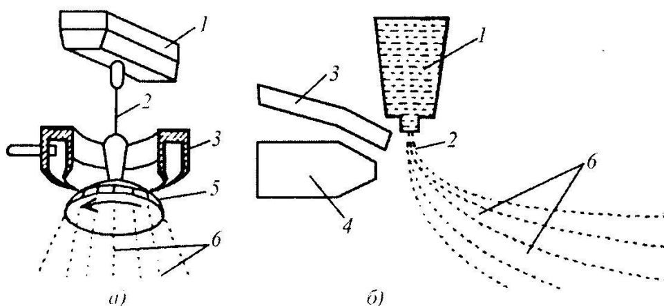
5.9 – расм. Шиша толасини марказдан қочма (а) ва пуфлаш (б) усулларида тайёрлаш схемалари. 1-шиша эритмали ванна; 2-эритма оқими; 3-иситгич; 4-сиқилган ҳаво узатувчи мослама; 5-марказий айланувчи мослама; 6-шиша толалари.
