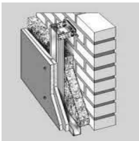
11.6 - расм. Гипскартон қопламали иссиқ сақловчи ташиқи девор конструкцияси
