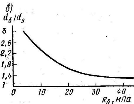
8.14 – расм. Бетон мустаҳкамлигини аниқлаш учун “таърировкалаш” графиги.
