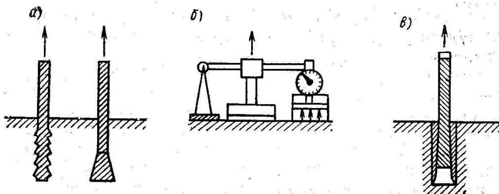
8.15 – расм. Бетоннинг мустаҳкамлигини маҳаллий бузиш орқали аниқлаш усуллари. а - олдиндан ўрнатилган металл стерженни суғуриб олиш; б - бетон юзасига елимланган шайбани узиб олиш; в - бетон танасига ўрнатилган тўмтоқ учли стерженни суғуриб олиш.
