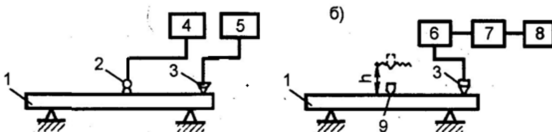
8.17 – расм. Бетонни титратиш усулида синаш схема-лари. а-резонанс усули; б-тебранишларнинг сўниши усули. 1-бетон намуна; 2-тебранишларни ҳосил қилгич, 3-тебранишларни қабул қилгич, 4-ўлчовчи генератор, 5-резонанс тебранишлар генератори, 6-тебранишларни йиғувчи қурилма, 7-стандарт частотали генератор, 8-электрон частота ўлчагич, 9-ургич.
