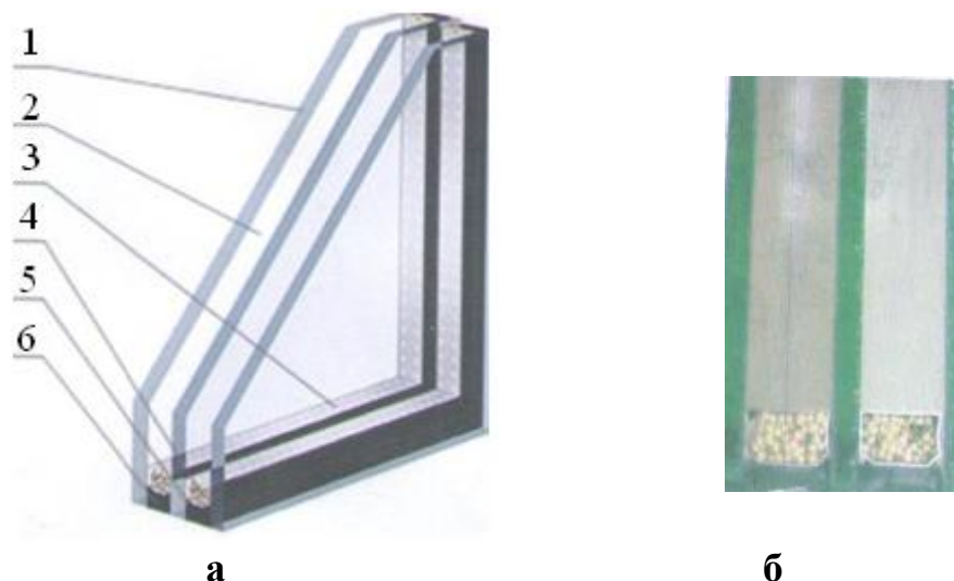
5.8 – расм. Замонавий шишапакет. а-икки камерали шишапакетнинг конструкцияси; б-шишапакетнинг қирқими. 1–треплекс ойна; 2–ҳаво бўшлиғи; 3-рама; 4-гигроскопик материал; 5-пластик елим; 6-бириктирувчи герметик.
