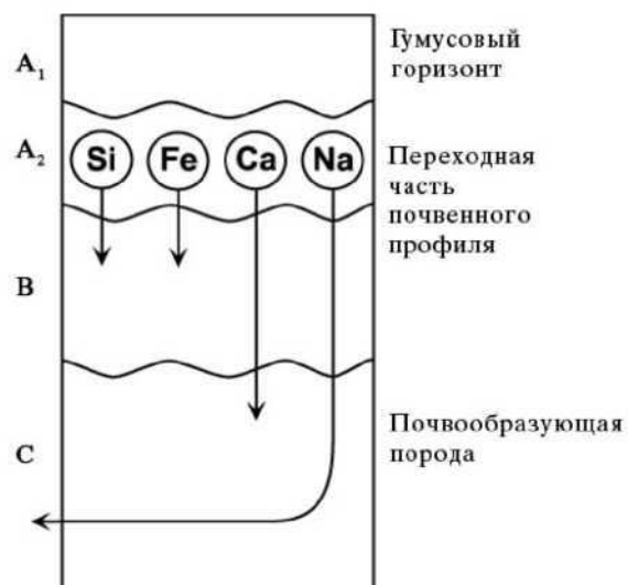
Рис. 7.1. Почвенный профиль автоморфных почв: A - перегнойно-аккумулятивный горизонт ( A 1 - минеральный гумусово-аккумулятивный, A 2 - элювиальный), B - горизонт вымывания (иллювиальный), C - материнская порода
