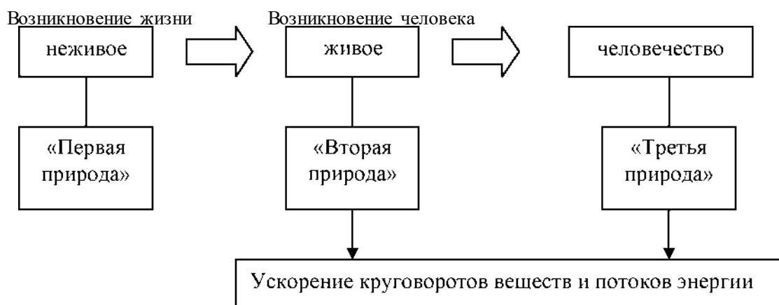
Рис. 5.5. Модель эволюции биосферы (по И.М. Швец, Н.А. Добротина «Биосфера и человечество», 2004)
