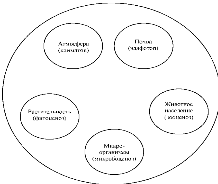
Рис. 4.1. Структура биогеоценоза и схема взаимодействия между компонентами
