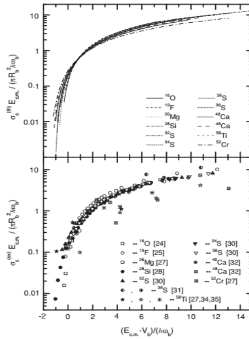
Рис. 8. Зависимость рассчитанных (верхняя часть) и экспериментальных (нижняя часть) значений \sigma_{cap} E_{cm} / (\pi R_b^2 \hbar \omega_b) \sigma_c E_{cm} / (\pi R_b^2 \hbar \omega_b) от (E_{cm} - V_b) / (\hbar \omega_b) (E_{cm} - V_b) / (\hbar \omega_b) для реакций с ^{208}\text{Pb} -мишенью и указанными налетающими ядрами, где V_b = V(R=R_b, J=0) V_b = V(R = R_b, J = 0) .
