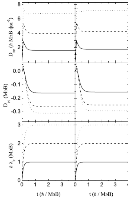
Рис. 1. Рассчитанные зависимости от времени микроскопических коэффициентов диффузии и трения для перевернутого (левая часть) и гармонического (правая часть) осцилляторов ( \mu=50m_0 и \hbar\omega =1\text{МэВ} ) при T=1\text{МэВ}
