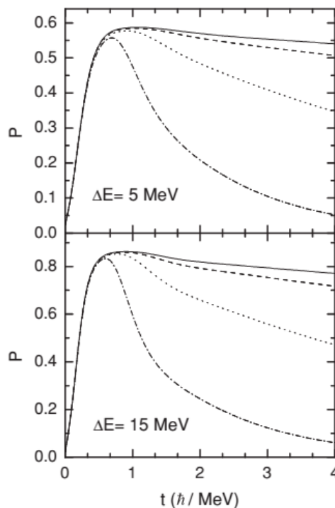
Рис. 4. Вероятность захвата P от времени t при энергиях столкновения \Delta E = E_{cm} - V(R=R_b, J) = 5 МэВ и 15 МэВ в реакции ^{48}\text{Ca} + ^{208}\text{Pb} . Энергия отсчитана от кулоновского барьера при J=0 (сплошная кривая), 30 (штриховая), 60 (пунктирная) и 90 (штрихпунктирная)
