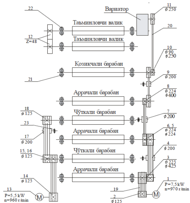
2 расм. ЧХ-3М2 “Меҳнат” пахта тозалаш машинасининг кинематик схемаси.
