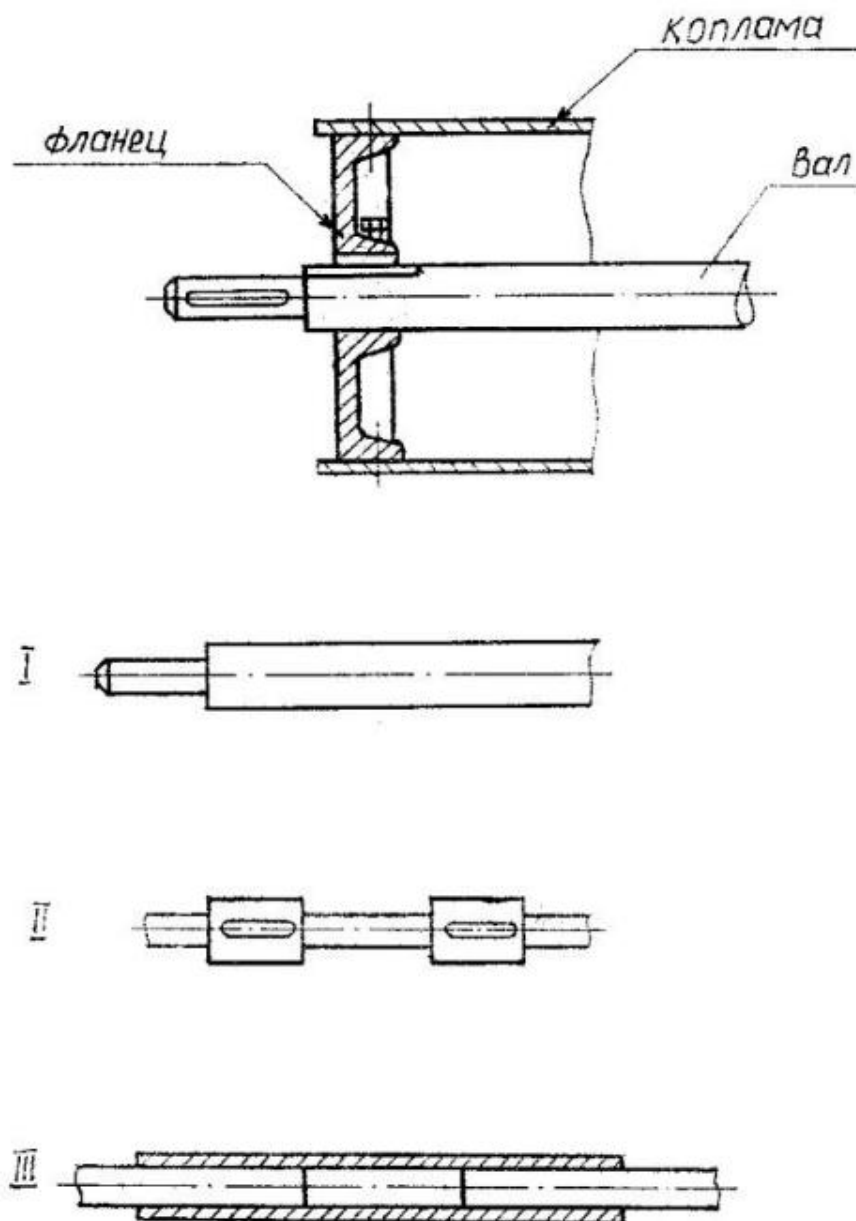
18-расм. Барабан ва валнинг кўриниши.
