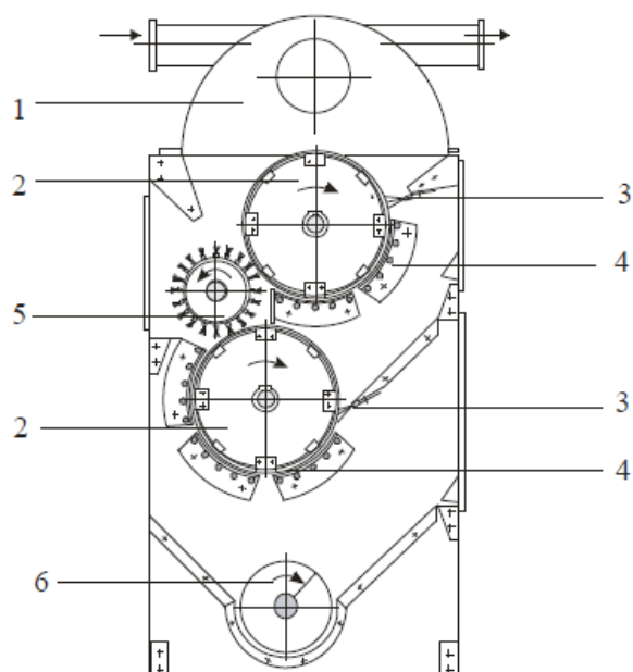
12 - расм. PX-1 пахтани регенерациялаш машинасининг схемаси 1- пневмотаъминлагич, 2- аррачали барабан, 3- илдирувчи чўтка, 4- колосникли панжара, 5- чўткали ажратувчи барабан, 6- винтли конвейер.
