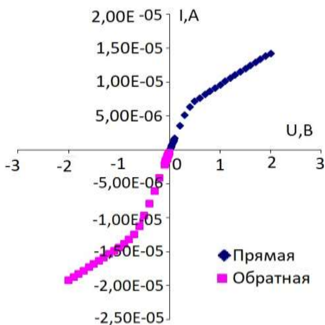
6-расм. Si<B,Mn> намунасидаги қоронғи холатдаги ВАХ (КДБ-3)
