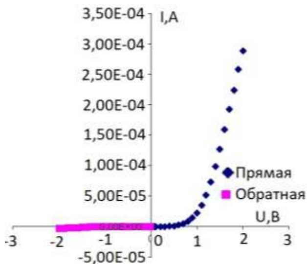
Рис.5. Темновая ВАХ образца Si<B,S>(исх. КДБ-1)
