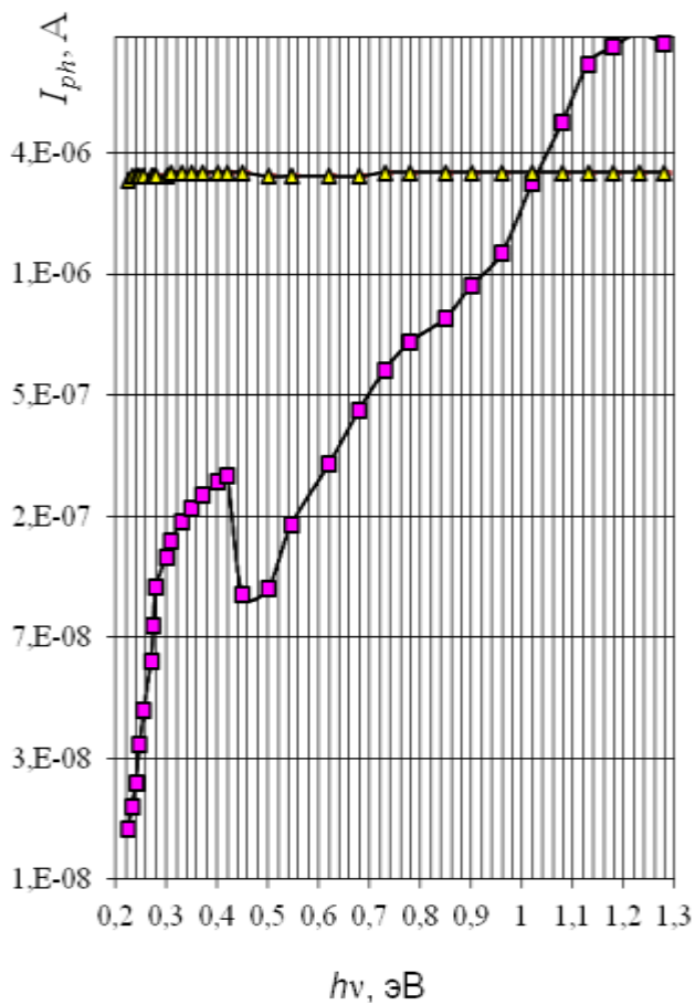
8-расм. Si<Mn,S> намунасида қоронғи ва ёруғлик ҳолатидаги Фўнинг спектрал боғлиқлиги
