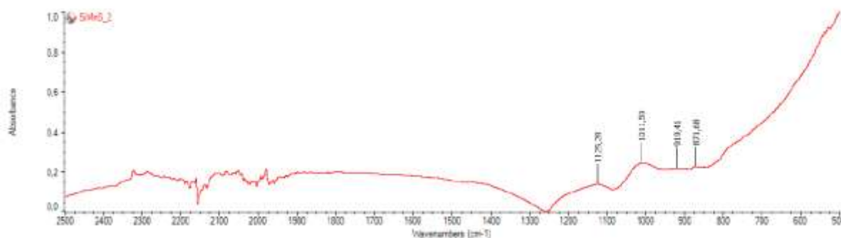
Рис. 7. ИК-колебательный спектр образца \text{Si}\langle\text{Mn,S}\rangle , полученный на FT IR Nicolet iS50 в диапазоне 2500 \div 500 \text{ см}^{-1} при T=300 \text{ K} с наиболее интенсивными модами 1125,28 \text{ см}^{-1} , 1011,50 \text{ см}^{-1} , 919,41 \text{ см}^{-1} и 871,68 \text{ см}^{-1} .
