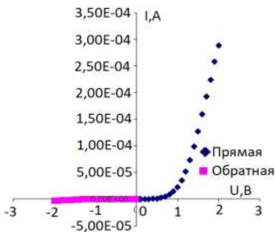
5-расм. Si<S> намунасидаги қоронғи ҳолатдаги ВАХ (КДБ-1)
