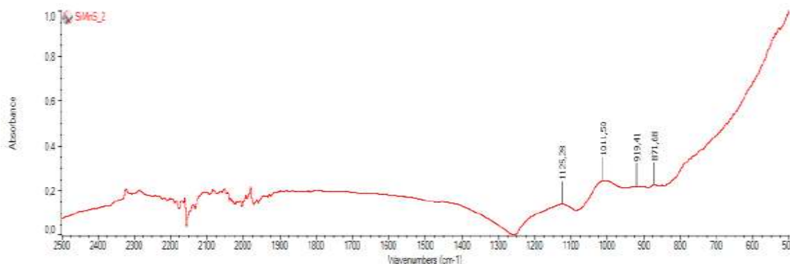
7-расм. FT IR Nicolet iS50Si қурилма ёрдамида <Mn,S> намунасида 2500÷500 оралиғида T=300K да олинган интенсив модалар 1125,28 см -1 , 1011,50см -1 , 919,41 см -1 ва 871,68 см -1 га тенг ИҚ-тебранма спектри
