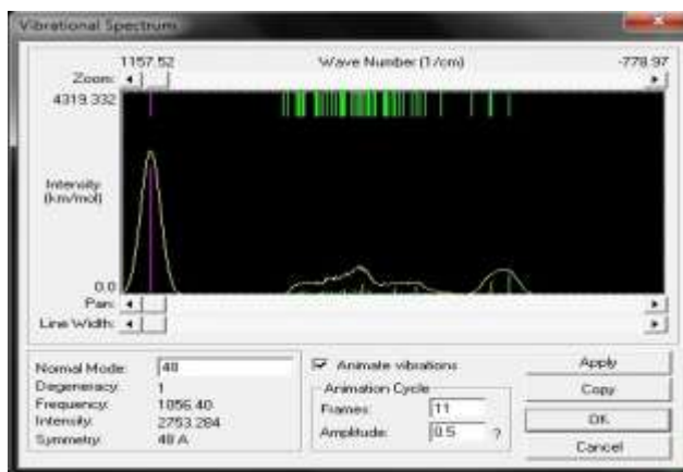
Рис.3. ИК-спектр ячейки \text{Si}_2\text{Mn}_2\text{S} модами колебаний
