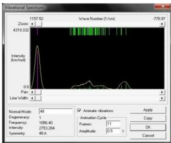
3-расм. \text{Si}_2\text{Mn}_2\text{S} ячейкасининг ИҚ –спектри тебранма модалари
