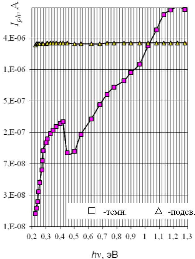
Рис. 8. Спектральная зависимость ФП в образце \text{Si}\langle\text{MnS}\rangle в темновых условиях и при постоянной подсветке
