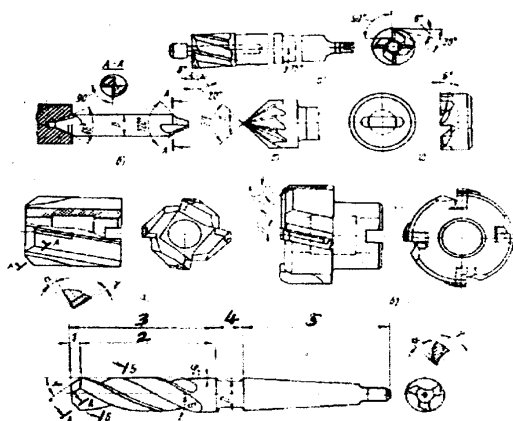
8 - расм. Зенкерлар
