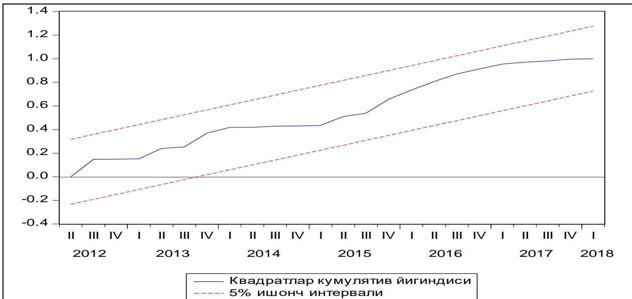
3-расм. CUSUM тести натижаси.
