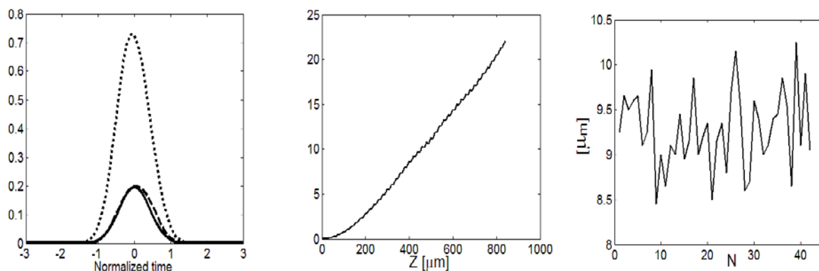
Рис. 7. Результаты алгоритма модельной закалки для 100 фс импульса второй гармоники с эффективностью 20% (в центре) для кристалла ниобата лития при длине волны 1550 нм основного излучения: слева – временной профиль основного излучения (точечный), планируемый (пунктирный) и полученный профиль второй гармоники (сплошной); справа – изменение размеров доменов в зависимости от их числа
