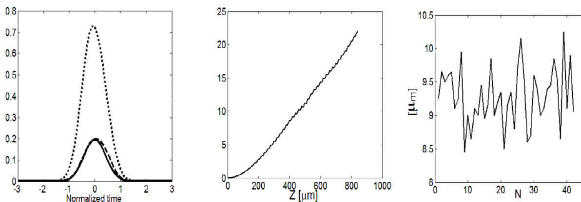
7-расм. Иккинчи гармоника импульсининг 100 фс модель тобланиш алгоритмини 20% эффективлик билан (марказда) литий ниобат кристалли учун асосий ёруғланишнинг 1550 нм. тўлқин узунлигида олинган натижалари: (чапдан) асосий ёруғланишнинг профили (нуқтали), режалаштирилган (пунктир) ва иккинчи гармоникани олинган профили (узлуксиз); (ўнгда) доменларни сонига қараб ўлчамларининг ўзгариши.
