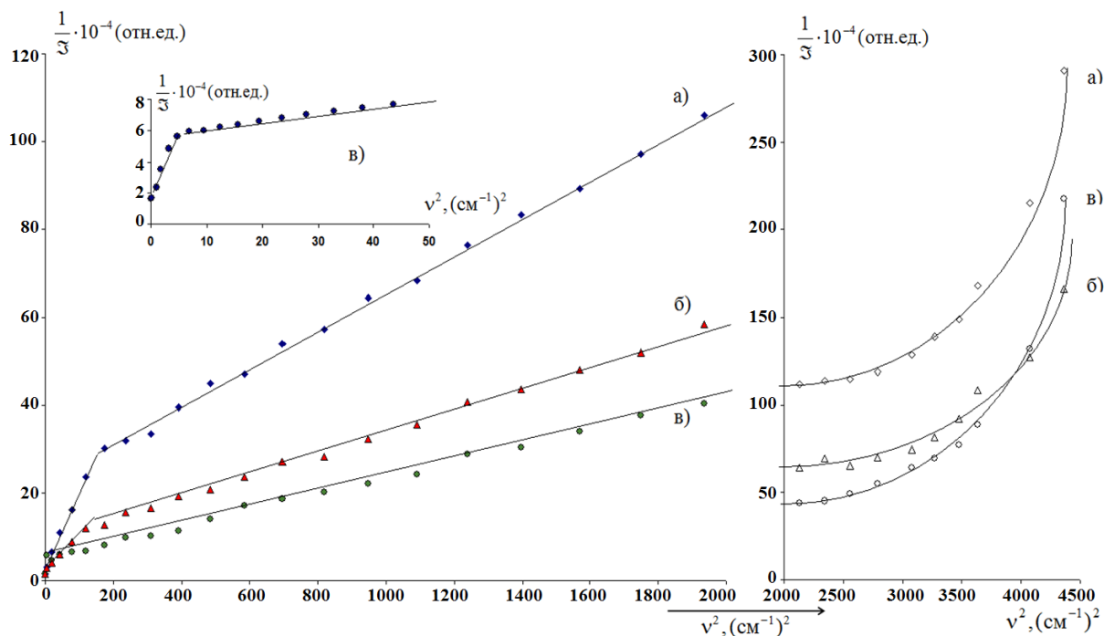
Рис. 1. Обратная спектральная плотность контура линии ДКМРС в молекуле бензола как функция квадрата частоты при температурах 293 К (а); 423 К (б); 553 К (в)
