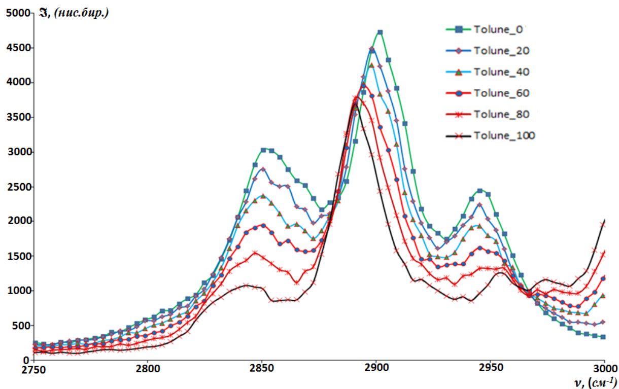
4 - расм. Толуолнинг этанол билан эритмасидаги ёруғликнинг комбинацион сочилиш спектрлари.
