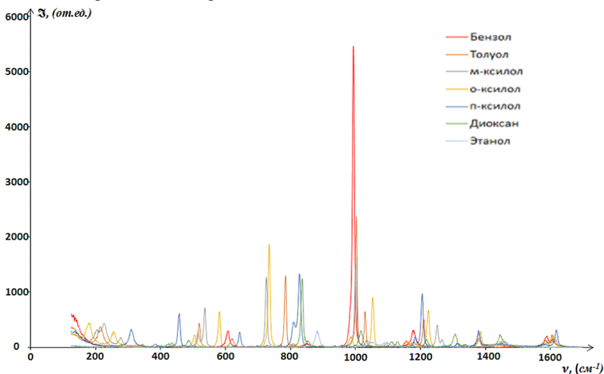
Рис. 3. Общий вид КРС в области 50\text{--}1600\text{ см}^{-1} для чистых исследованных жидкостей
