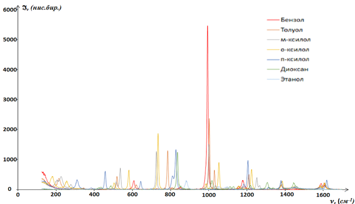
3-расм. Ўрганилган тоза суюқликларда ёруғликнинг комбинацион сочилиш спектрининг 50-1600 \text{см}^{-1} соҳа учун умумий кўриниши.
