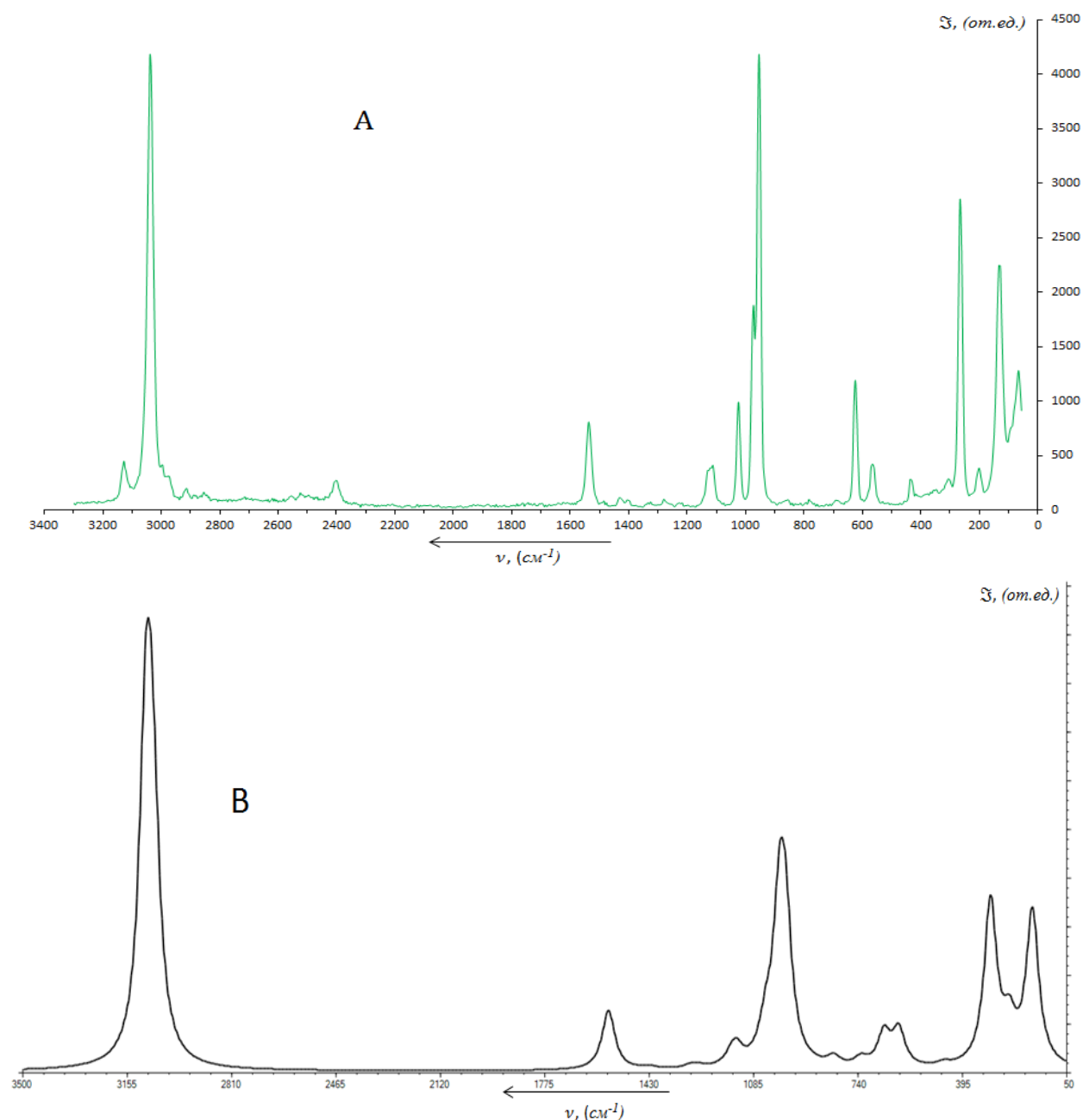
Расм.5. Бромбензол молекулалари учун ёруғликнинг комбинацион сочилиш спектрлари чизиғи интенсивлигининг частотага боғлиқлиги. А – тажриба, В –квант-кимёвий ҳисоблашлар.
