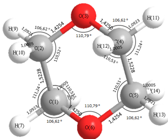
Рис. 6. Длина связи и углы между связями атомов молекулы диоксана
