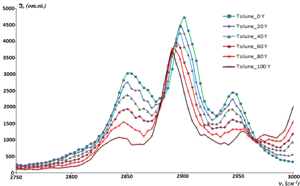
Рис. 4. Полосы КРС толуола в растворе с этанолом
