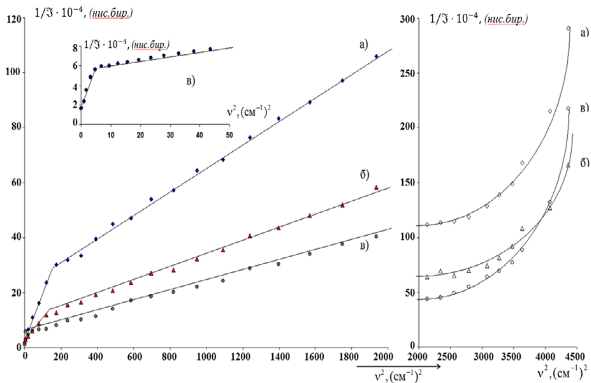
1-расм. Ёруғлик молекуляр сочилишининг ноқутбланган компонентаси контури спектрал зичлигининг частота квадратиға температуравий боғлиқлик графиги: а) 293 K; б) 423 K; в) 553 K.
