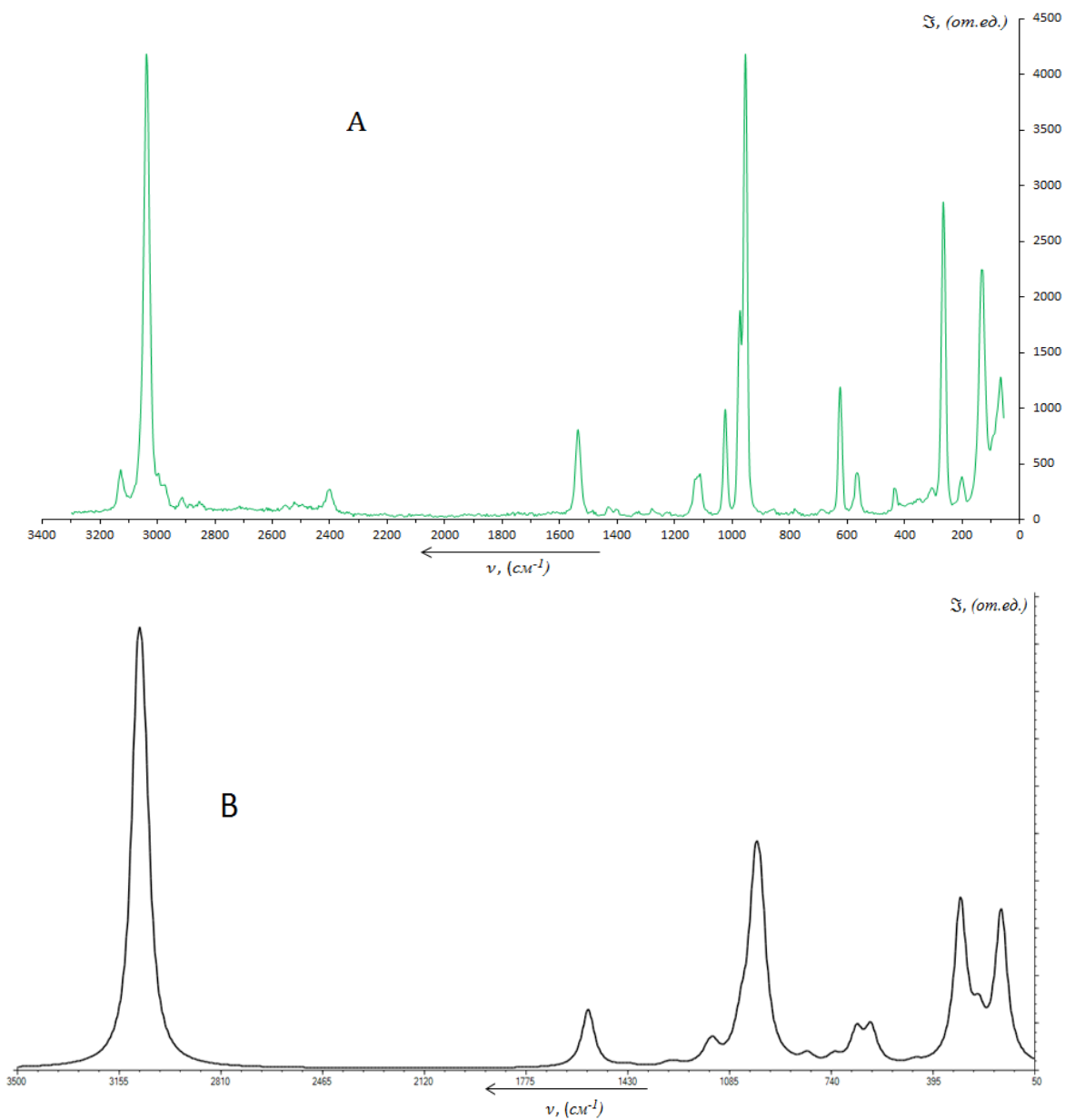
Рис. 5. Зависимость спектральной интенсивности контура линии КРС от частоты для молекул бромбензола: А – эксперимент, В – квантово-химический расчёт
