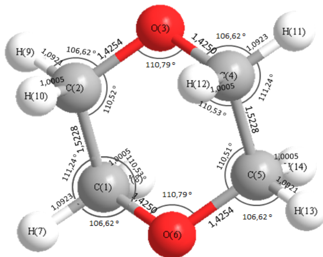
6-расм. Диоксан молекуласининг атомлар боғлари узунлиги ва улар орасидаги бурчаклар.
