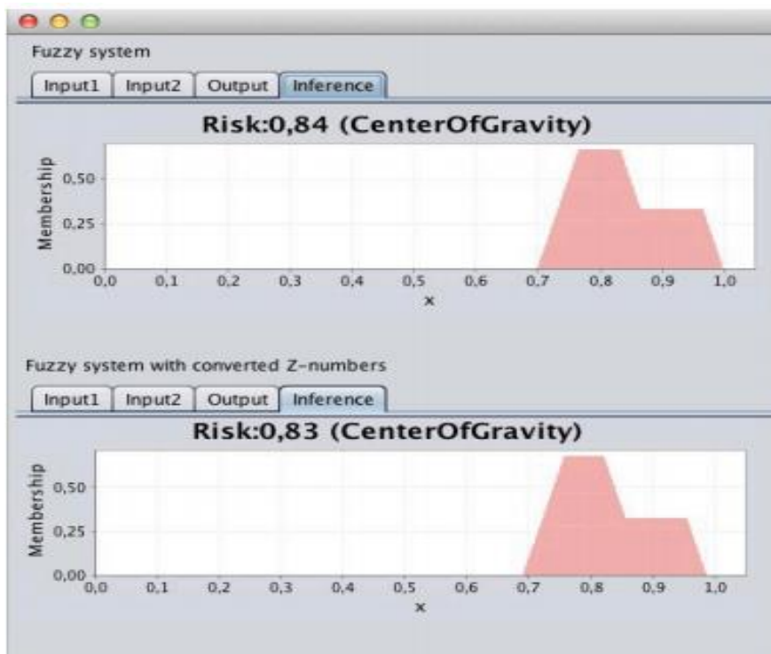
Рис. 7. Результаты, полученные на основе базы знаний
