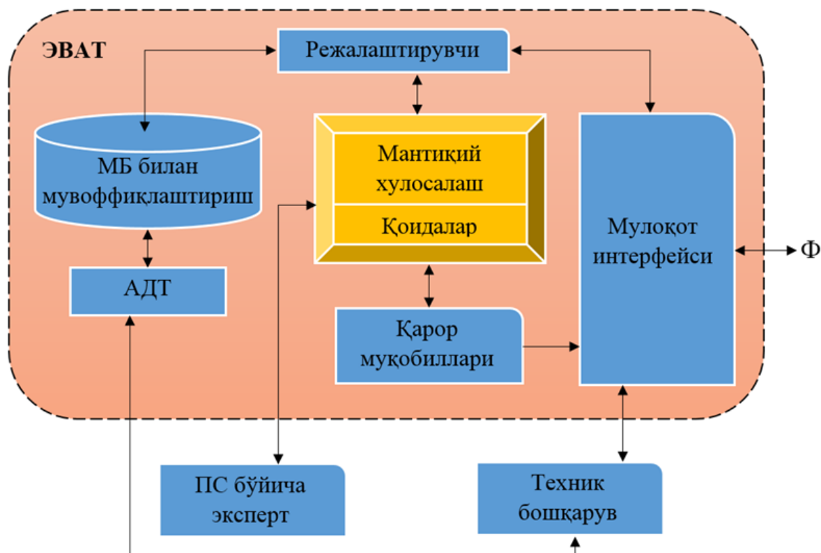
8-расм. ЭВАТ тузилмаси
