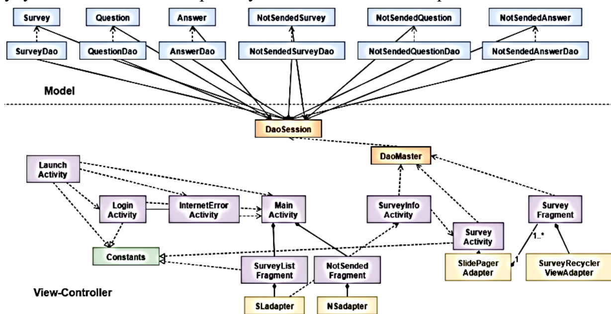
5-Расм. MVC архитектурасида синфлар боғланиш схемаси
