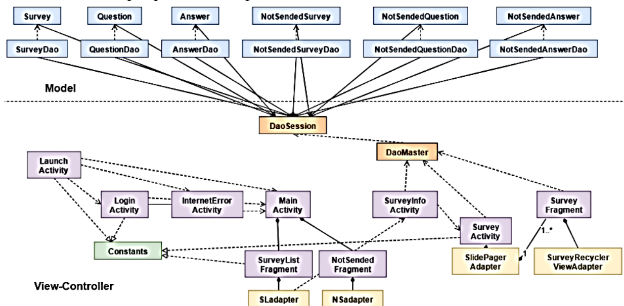
Рис. 5. Схема взаимосвязей между классами в архитектуре MVC
