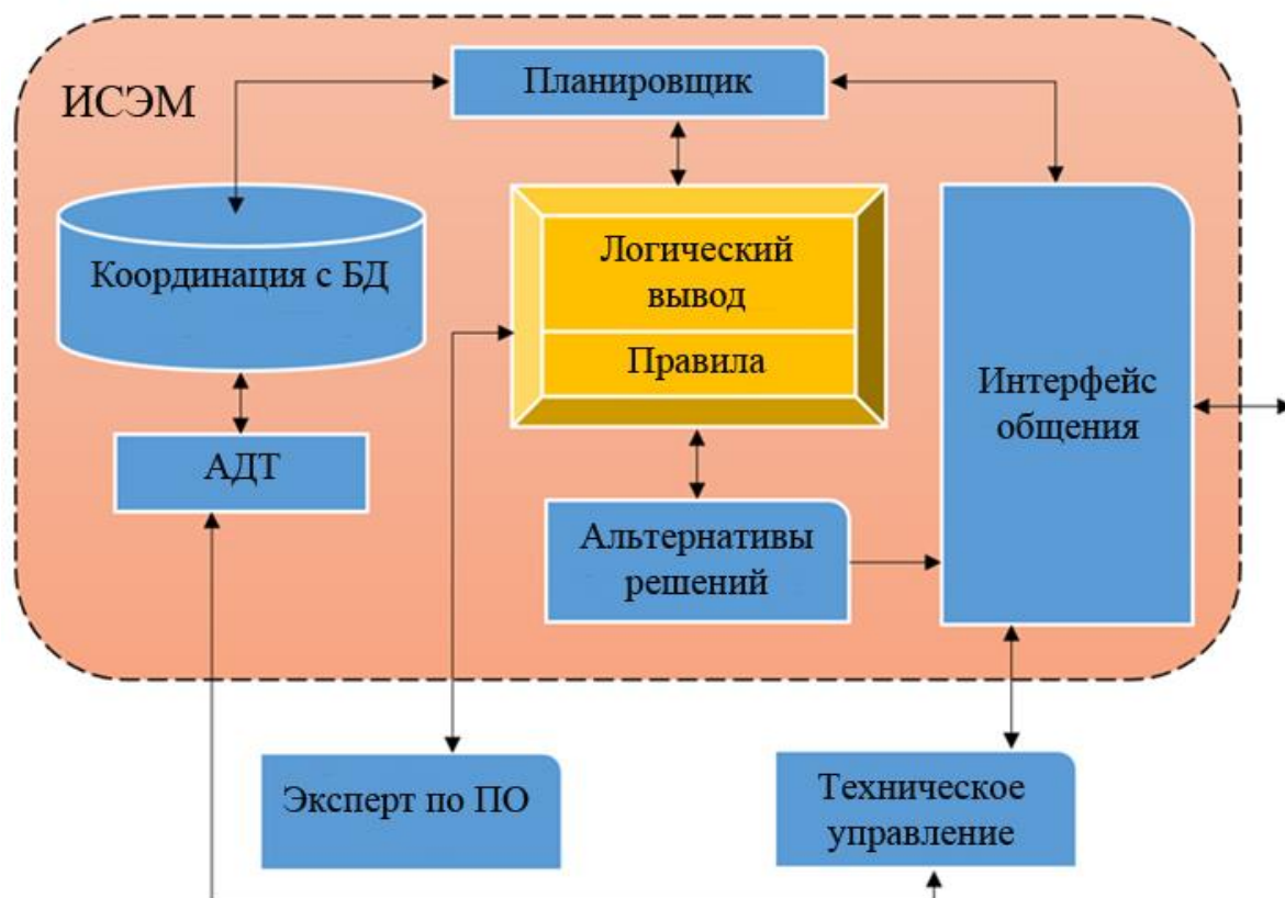
Рис. 8. Структура ИСЭМ
