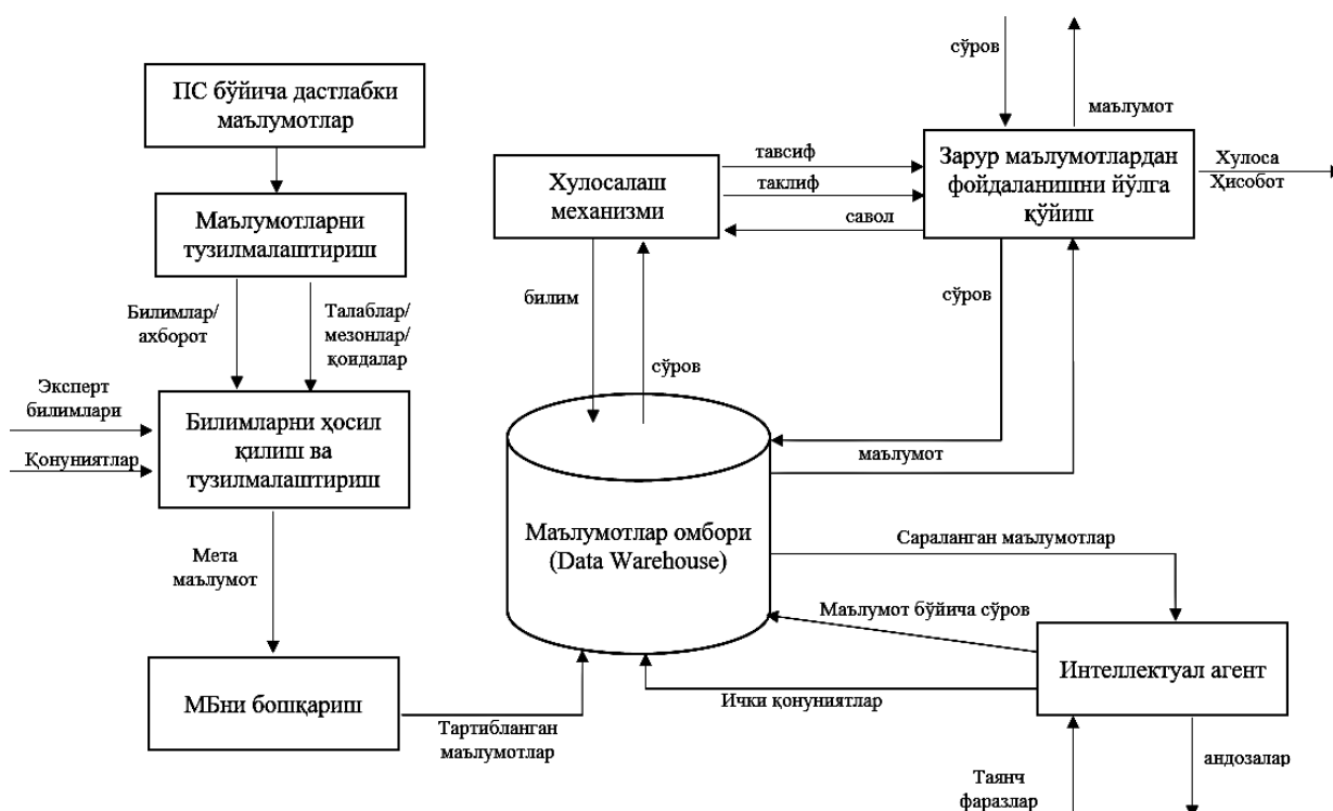
3-расм. Предмет соҳа бўйича билимларни тақдим қилишнинг умумлашган тузилмаси
