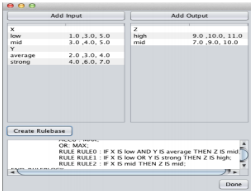
Рис. 6. Вид программы создание базы продукционных знаний
