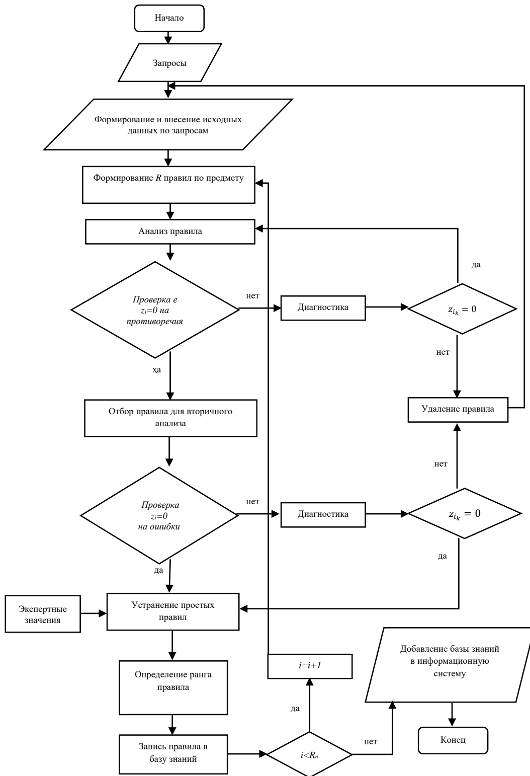
Рис. 4. Алгоритм формирования базы знаний информационных систем, ориентированных на повышение эффективности альтернативности решений в информационных системах
