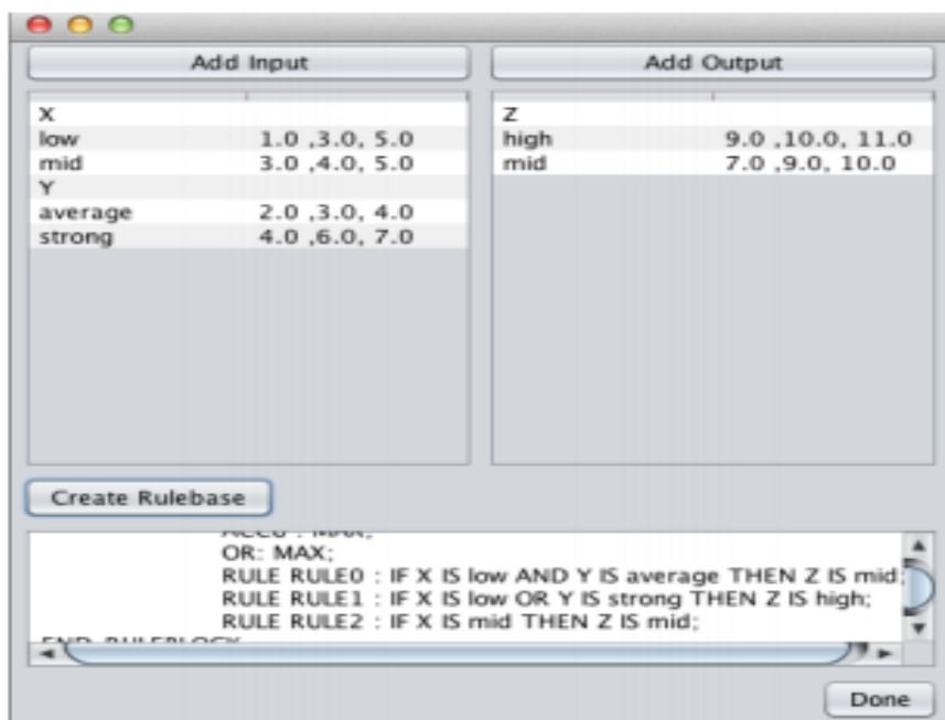
6-расм. Продукцион билимлар базасини яратиш дастурининг кўриниши
