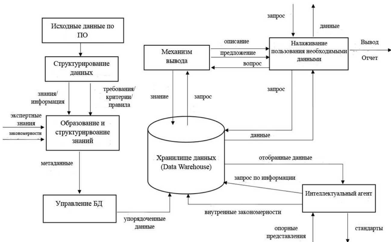
Рис. 3. Обобщенная структура представления знаний в предметной области
