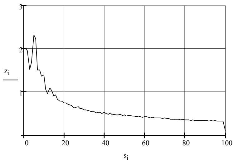
5.11.-rasm. Bulstoer funksiyasi uchun natijalar
