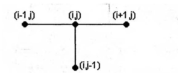
6.5-rasm. Ikki qatlamli ayrimaning oshkormas sxemasi.
