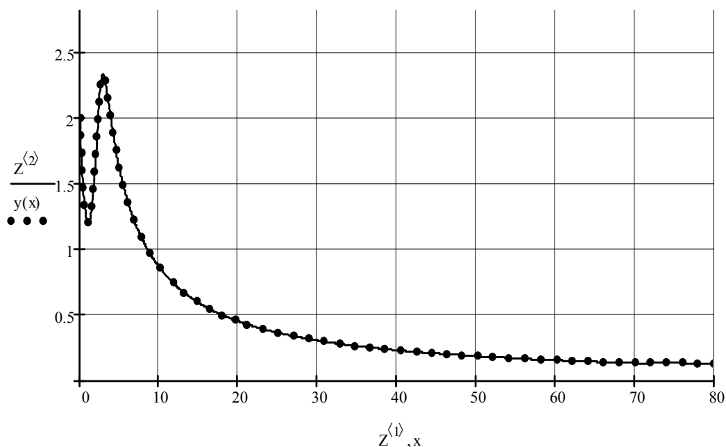
5.15-rasm. Odesolve va rkfixed funksiyalari uchun yechimlar grafiklari
