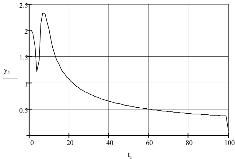
5.10-rasm. Rkadapt funksiyasi uchun natijalar
