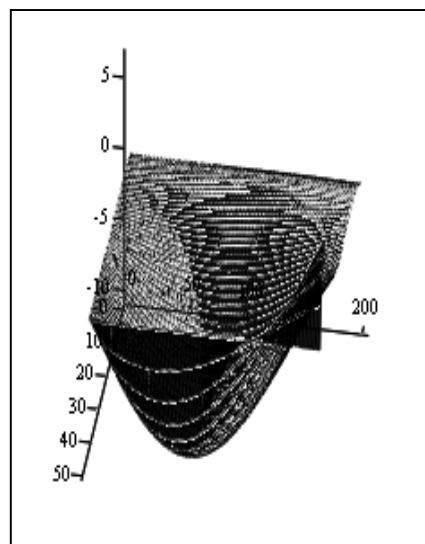
6.4-rasm. Masalaning grafik yechimi.
