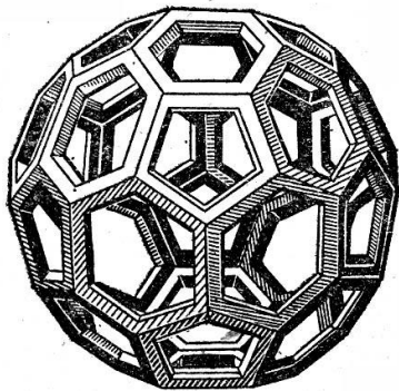
Қуръа (икосаэдр) ва кесик қуръа (кесик икосаэдр) расмлари (Леонардо да Винчи чизган расмлар).
