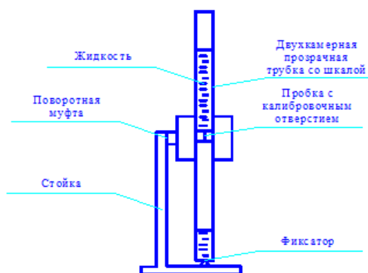
2.7-расм. Гидравлик толчкомер
