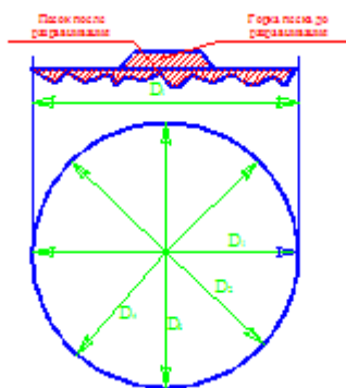
2.9-расм. Кумли дог усулида қолама тишлаши сифатини аниқлаш.
