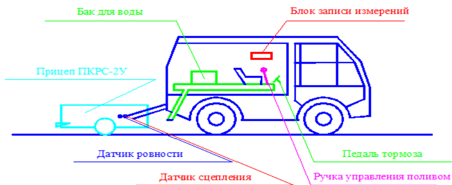
2.8-расм. Динамометрик аравача ПКРС-2У
