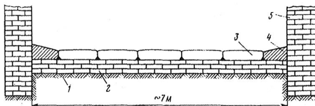
1.1-расм. Дастлабки қаттиқ қопламали йўлнинг кундаланг кесими.
