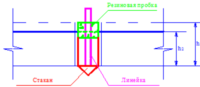
2.12-расм. Износмер
