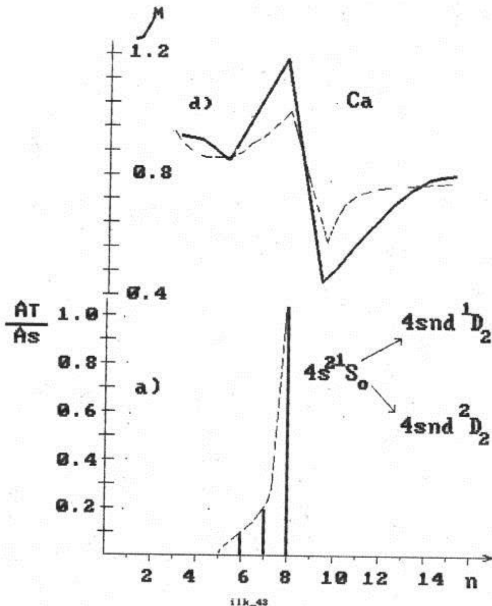
Рис..5.12 Атом Ca. а) Зависимость отношения амплитуд резонансов A_T / A_S от n . Для n = 5-8 данные нашей работы, для n = 12-14 работы [32]
