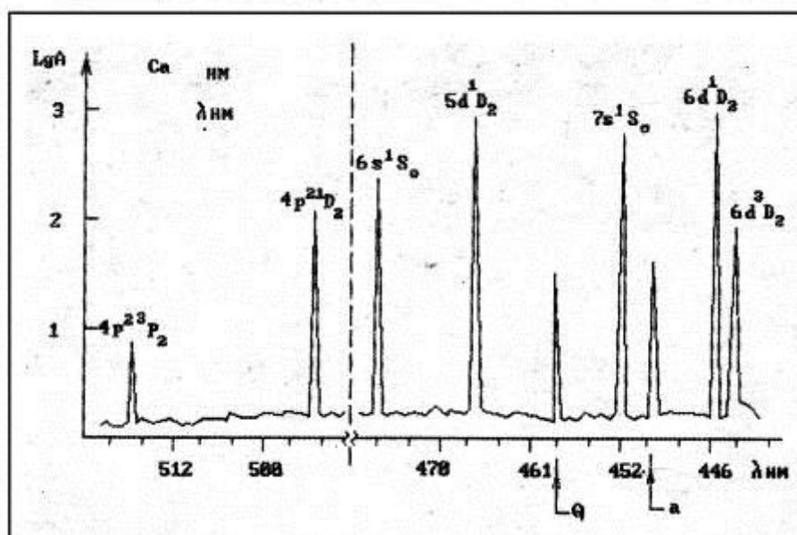
Рис.5.1. Участок спектра атома Ca, полученный методом многофотонной ионизационной спектроскопии. О, - однофотонный квадрупольный переход 4s^2 \ ^1S_0 - 4s3d^2D_2 , а - однофотонный переход 4s4p \ ^1P_1 - 4s8s^1S_0 .
