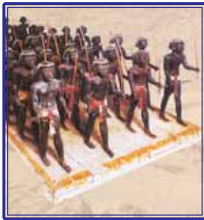
A'yyemgi Mi'si'r a'skerlerinin' gu'laldan jasalg'an ha'ykelleri
