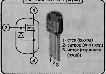
КР1014КТ1А (В)
