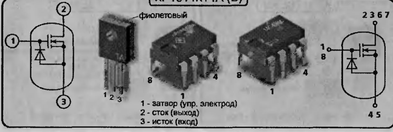
КР1014КТ1А (В)
