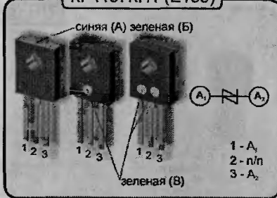
КР1014КТ1А (В)
