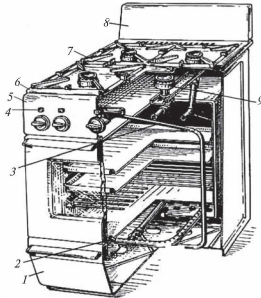
7-rasm. 4-konforkali GP ko'rinishi.
