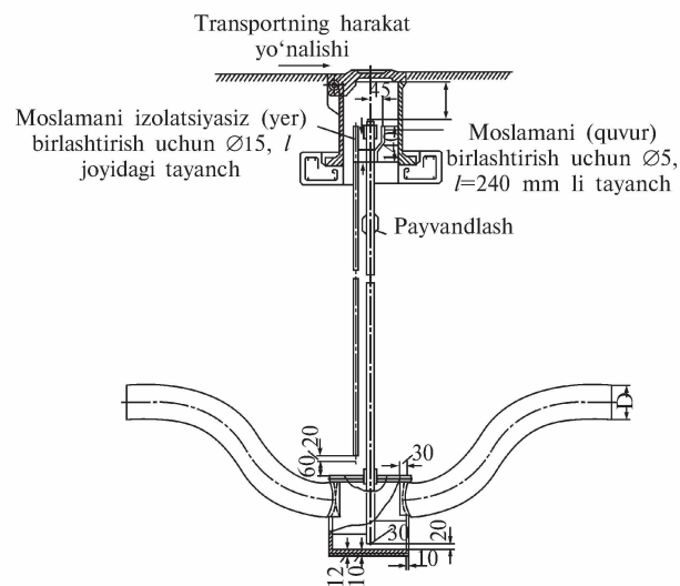
3-rasm. Elektr o'lchov uchun kondensat yig'uvchi uskuna.
