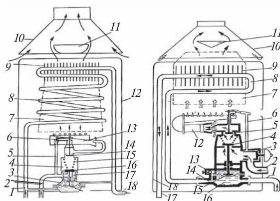
8-rasm. GSI-18 ko'rinishli suv isitgichning prinsipial sxemasi: 1—suvning kirishi; 2—gazning kirishi; 3—blokli kran; 4—suv va gazni blokirovka qiluvchi klapan; 5—xavfsizlikni ta'minlovchi klapan; 6—gazni alangalatish; 7—yonuv o'chog'i; 8—spiral ko'rinishli quvur (змеевик); 9—buramali kalorifer; 10—tutun gazi chiquvchi joy; 11—tutun gazini qaytarishdan saqlagich; 12—gorelka; 13—sharikli yondirgichni so'ndirgich; 14—Venturi quvuri; 15—membranali kamera; 17—suvning chiqishi; 18—kojux.
