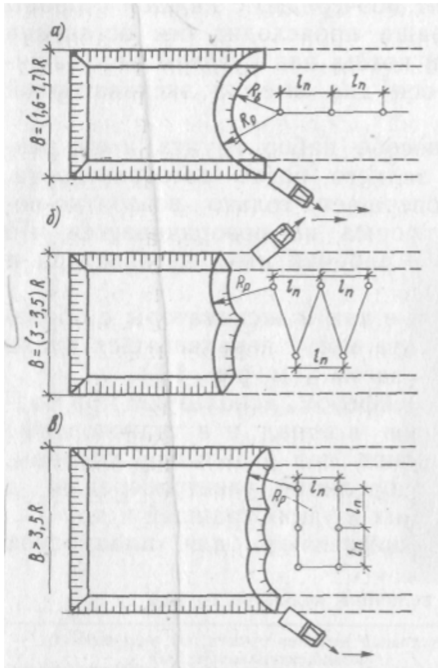
Рис. 6. Схема проходки экскаватора обратная лопата при разработке котлована: а — вдоль котлована; б — зигзагом; в — поперек котлована.
