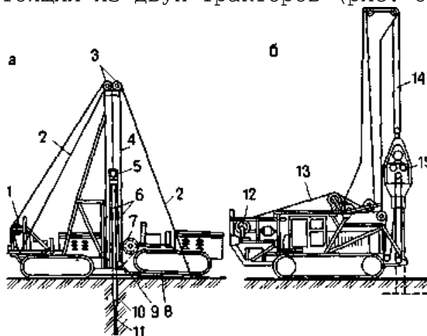
Рис. 5. Установки для статического вдавливания (а) и вибровдавливания (б) свай : 1 – лебедка с тяговым канатом для опускания опорной плиты и подъема наголовника; 2 – растяжки стрелы; 3 – блоки для тягового каната; 4 – рама стрелы; 5 – наголовник сваи с блоками для рабочего каната; 6 – рабочий канат; 7 – лебедка, создающая нагрузку; 8 – опорная плита; 9 – отводной блок рабочего каната; 10 – свая; 11 – лидерная скважина; 12 – двухбарабанная лебедка, создающая нагрузку; 13 – рабочий канат с блоками; 14 – канат с блоками для подъема вибропогружателя; 15 – вибропогружатель
