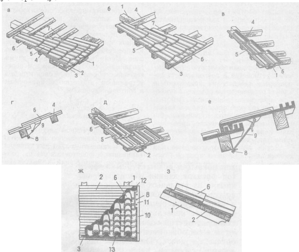
Рис. 3. Устройство кровель из черепицы :
