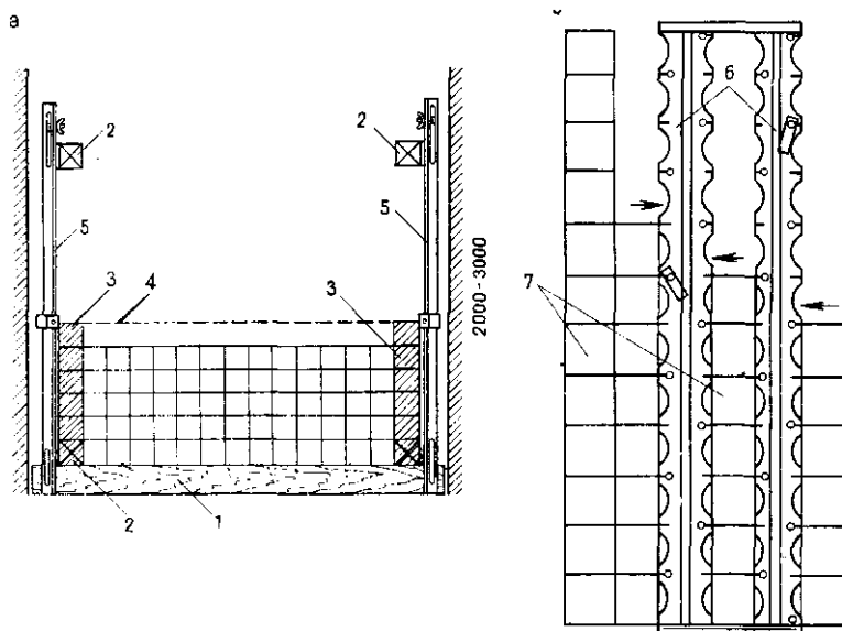
Рис. 2.3 - Устройство облицовки стен из керамической плитки на растворе: а - технологическая схема выполнения облицовки; б - схема укладки плиток с помощью шаблона; 1 - горизонтальный брус; 2 - марки; 3 - маячные ряды; 4 - шнур-причалка; 5 - порядовки; 6 - шаблон; 7 - облицовочные плитки.
