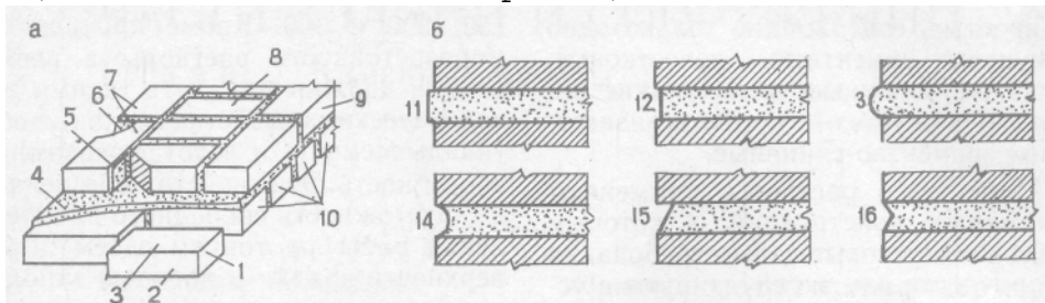
Рис. 1. Элементы каменной кладки (а) и виды расшивки (б) : 1 – тычок; 2 – ложка; 3 – постель; 4 – горизонтальный шов; 5 – поперечный шов; 7 – наружная ложка верста; 8 – забутка; 9 – внутренняя ложка верста; 10 – внутренняя тычковая верста; 11 – прямоугольная расшивка шва; 12 – то же, заглубленная; 13 – выпуклая; 14 – вогнутая; 15 – односрезная; 16 – двухсрезная.
