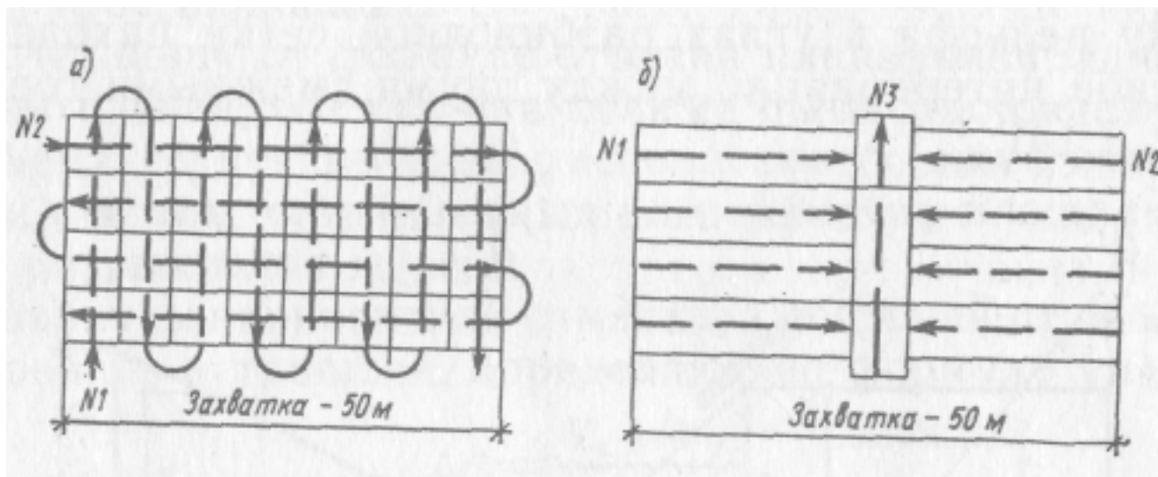
Рис. 6. Схемы движения бульдозеров: а – продольно-поперечный; б – поперечно челночный; № 1, № 2. № 3 – бульдозеры.
