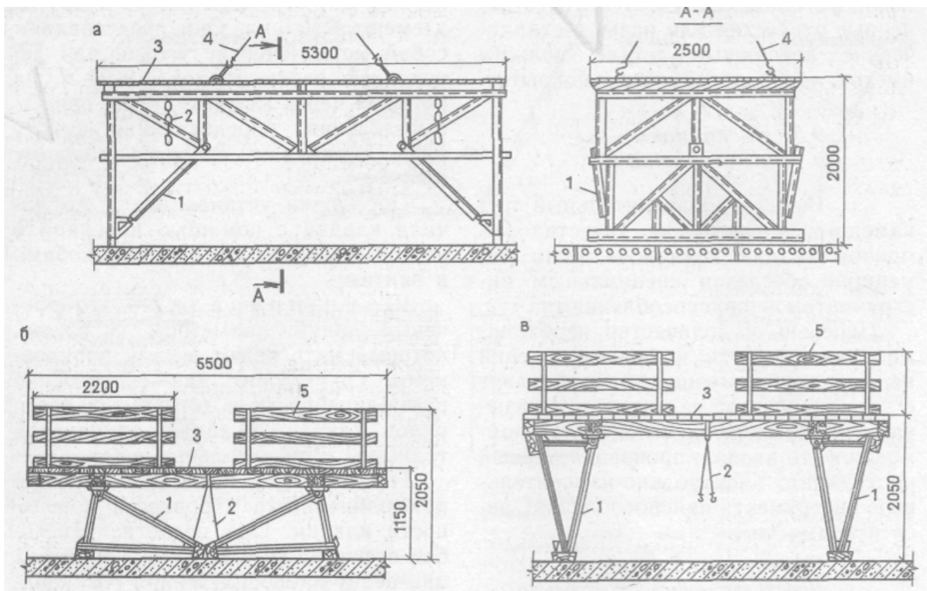
Рис. 4. Подмости для выполнения каменных работ : а – инвентарные блочные; б – шарнирно-панельные при кладке второго яруса; б – то же, третьего яруса; 1 – откидная опора; 2 – цепь (канат) для крепления откидных опор; 3 – рабочий настил; 4 – канатная подвеска; 5 – инвентарные ограждения.
