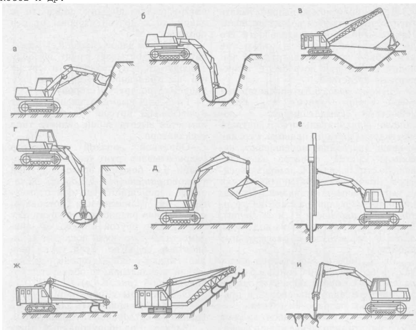
Рис. 1. Одноковшовые экскаваторы с рабочим сменным оборудованием : а - прямая лопата; б - обратная лопата; в - драглайн; г - грейфер; д - кран; е - сваебойный копер; ж - струг; з - планировщик откосов; и - рыхлитель грунта
