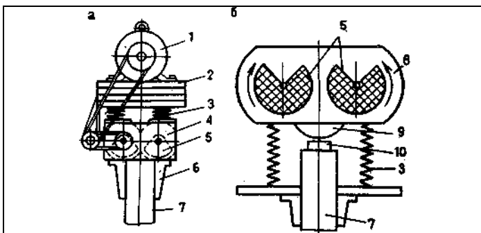
Рис. 4. Схема вибропогружателя (а) и вибромолота (б)
