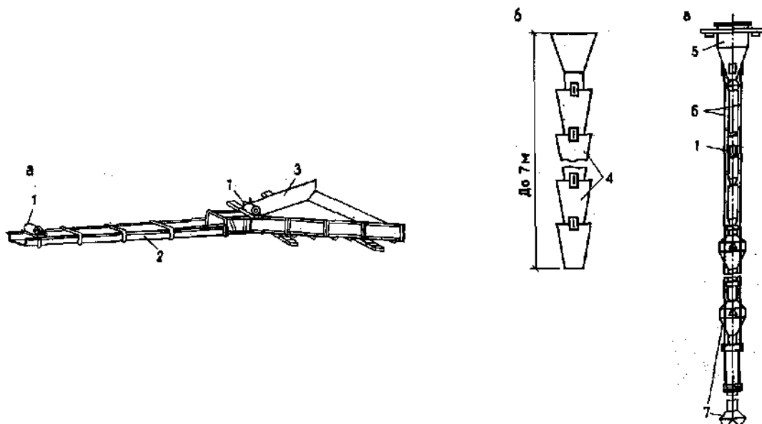
Рис. 1. Средства для подачи бетонной смеси : а - вибропитатель и виброжелоб; б - звеньевой хобот; в - виброхобот; 1 - вибраторы; 2 - виброжелоб; 3 - вибропитатель; 4 - элементы хобота; 5 - воронка; 6 - канаты; 7 - гасители.
