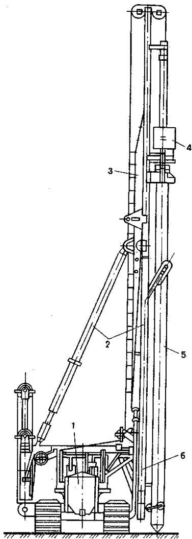
Рис. 2. Сваебойная установка на базе трактора
