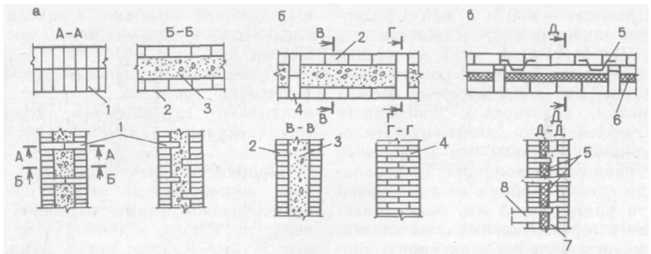
Рис. 3. Виды облегченных кладок : а – кирпично-бетонная; б – колодцевая; в – с термовкладышами конструкции ЦНИИСК им. В.А. Кучеренко; 1 – тычковый ряд; 2 – ложковый ряд; 3 – легкий бетон; 4 – поперечная стенка-перегородка; 5 – скобы; 6 – теплоизоляционные плиты; 7 – воздушная прослойка; 8 – перекрытие.
