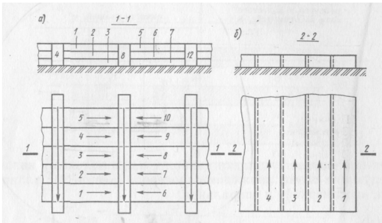
Рис. 5. Схема резания грунта бульдозерами: а - траншейным зарезанием; б - послойная; 1, 2, 3, ... - последовательность резания.
