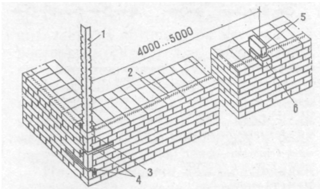
Рис. 4. Установка причалки с помощью порядовок : 1 – инвентарная металлическая порядовка; 2 – причалка; 3 – ползунок для крепления и передвижения причалки; 4 – скобы для крепления порядовки к стене; 5 – прижимной кирпич; 6 – маячный кирпич.
