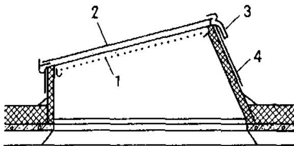
Рис. 1.3 – Конструктивная схема зенитного фонаря точечного типа : 1 – защитная сетка; 2 – светопрозрачное заполнение; 3 – механизм открывания; 4 – опорный стакан.
