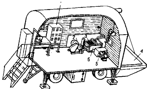
Рис. 2.1 – Штукатурная станция : 1 – пульт управления; 2 – растворонасос; 3 – вибросито; 4 – приёмный бункер; 5 – компрессор; 6 – бункер растворонасоса.
