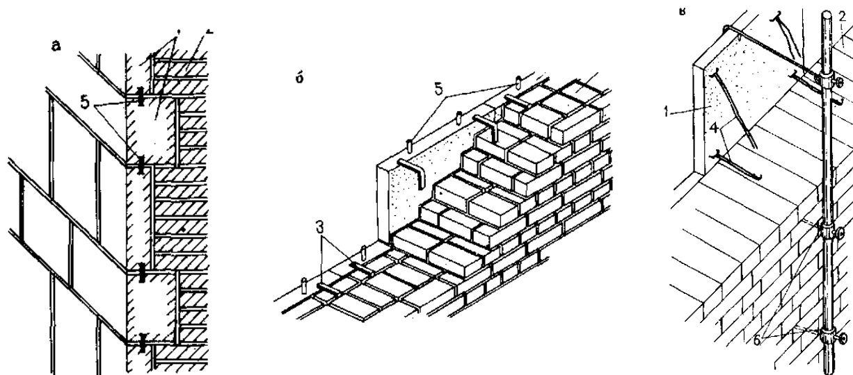
Рис. 2.1 – Устройство облицовки наружных стен одновременно с ведением кладки : а – в перевязку с кладкой; б – с жестким креплением к кладке; в – приспособление для временного закрепления плит; 1 – облицовка; 2 – кладка; 3 – детали жестких креплений для ведения облицовки природным камнем одновременно с кладкой; 4 – то же, искусственными декоративными плитами; 5 – пироны; 6 – приспособление для временного закрепления плит облицовки.
