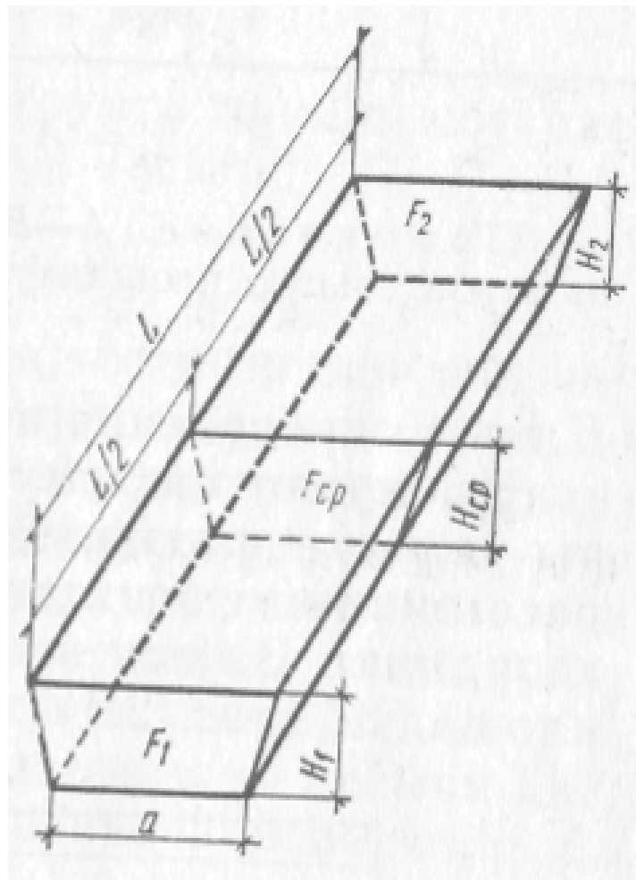
Рис. 2. Вид траншеи и схема для определения её объема.
