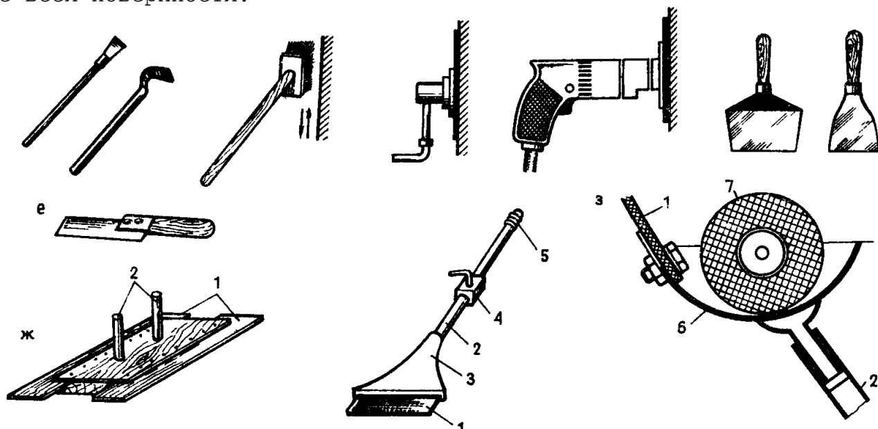
Рис. 1.1. Инструмент для подготовки поверхностей под окраску а — скребки; б — щетка; в — затирочно-шлифовальная машина пневматическая; г — то же, электрическая; д — стальные шпатели; е — малярный нож; ж — шпатель-полутёрка; з — механизированный шпатель плоский и с валиком; 1 — полотно шпателя; 2 — рукоятка; 3 — корпус; 4 — вентиль для включения подачи шпатлёвки; 5 — штуцер; 6 — ванночка; 7 — валик
