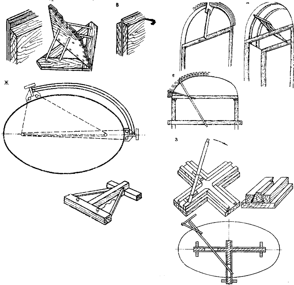
Рис. 2.7 - Оснастка для шаблонов : а - профильная доска с двойной оковкой для тяг с декоративной накрывкой; б - шаблон для прямолинейных тяг с входящими углами; в - профильная доска для прямолинейных тяг с входящими углами; г - шаблон с воробой для вытягивания архивольта; д - шаблон с воробой для вытягивания профилей подпружных арок; е - шаблон с воробой - ножницы для вытягивания двуцентровых тяг; ж - шаблон со шнуром для вытягивания двуцентровых тяг; з - шаблон с воробой и патроном для вытягивания двуцентровых тяг.
