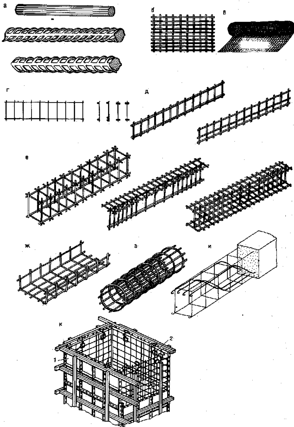
Рис. 1. Виды арматуры : а – арматурные стержни; б – плоская арматурная сетка; в – рулонная арматурная сетка; г – проволочная арматура; д – плоские каркасы; е – пространственные каркасы; ж – гнутый каркас; з – цилиндрический каркас; и – каркас с отогнутыми стержнями, вязанный; к – арматурно-опалубочный блок; 1 – щит опалубки; 2 – арматурный каркас
