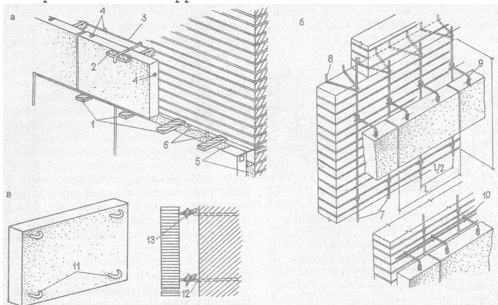
Рис. 2.2 – Устройство облицовки плитами по готовым стенам : а – временное закрепление ряда облицовки с жесткой анкерровкой; б – установка облицовки со скользящей анкерровкой; в – крепление искусственных облицовочных плит; 1 – уравнивательные клинья; 2 – натяжной клин; 3 – временный натяжной анкер; 4 – отверстия для анкеров и пиროнов; 5 – раствор; 6 – пирон; 7 – вертикальные стержни; 8 – анкеры для крепления стержней; 9 – скользящие анкеры; 10 – горизонтальный скользящий анкер; 11 – монтажные петли; 12 – анкерный крюк; 13 – проволочные крепления монтажных петель к анкерам.
