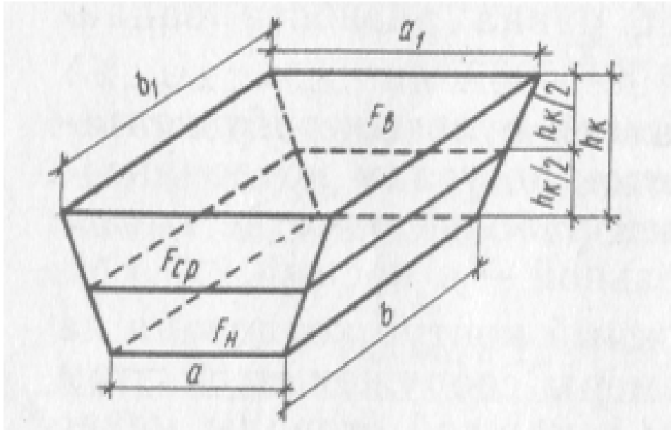
Рис. 1. Вид котлована и схема для определения его объема Траншея - выемка менее 3-х метров и длиной многократно превышающей ширину (рис. 2).
