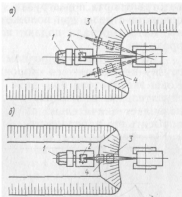
Рис. 9. Способы разработки забоя экскаватором драглайн: а – поперечно-челночный; б, д – продольно-челночный; 1 – автосамосвал; 2 – разгрузка ковша; 3 – окончание набора и подъем ковша; 4 – опускание ковша и набор грунта.
