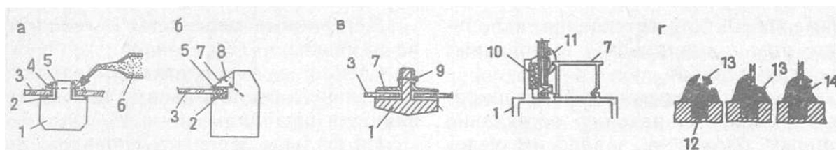
Рис. 1.1 - Остекление переплетов : а - деревянных на замазке; б - деревянных на штапиках; в - металлических на штапиках с уплотнителями; г - со шпунтом для установки фигурных замковых уплотнителей; 1 — переплет; 2 — слой замазки (первый); 3 — стекло; 4 — стальные шпильки; 5 — замазка (второй слой); 6 — шприц для нанесения замазки; 7 — штапики; 8 — шурупы; 9 — болт; 10 — зубчатая прокладка; 11 — лепестковая прокладка; 12 — гребень уплотнителя; 13 — бортик уплотнителя; 14 — замковый профиль уплотнителя.
