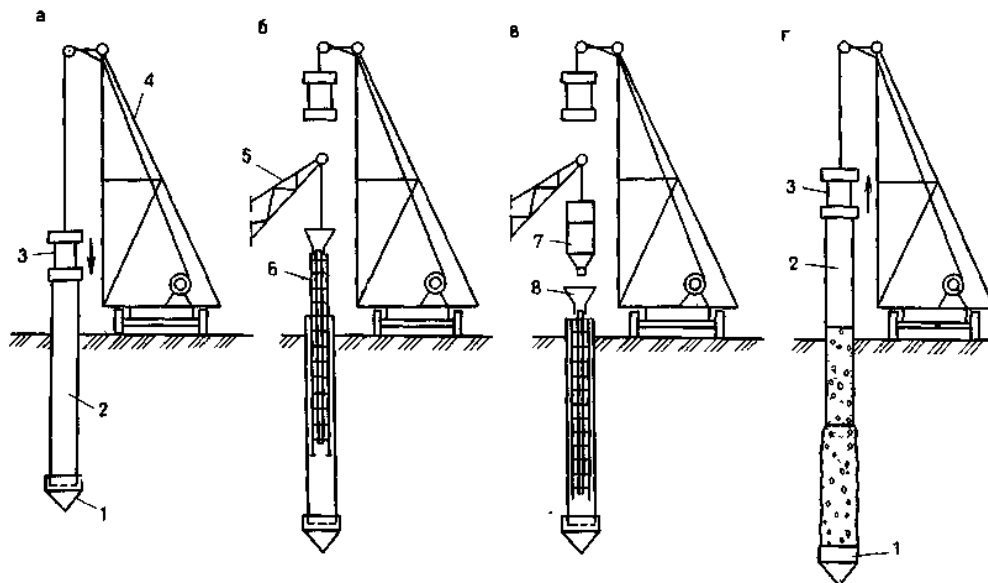
Рис. 5. Технологическая схема устройства частотрамбованных свай : а – погружение обсадной трубы; б – установка арматурного каркаса; в – подача бетонной смеси в полость трубы; г – извлечение обсадной трубы с одновременным уплотнением бетонной смеси; 1 – съемный башмак; 2 – обсадная труба; 3 – молот двойного действия; 4 – копер; 5 – кран; 6 – арматурный каркас; 7 – вибробадья; 8 – приемная воронка.
