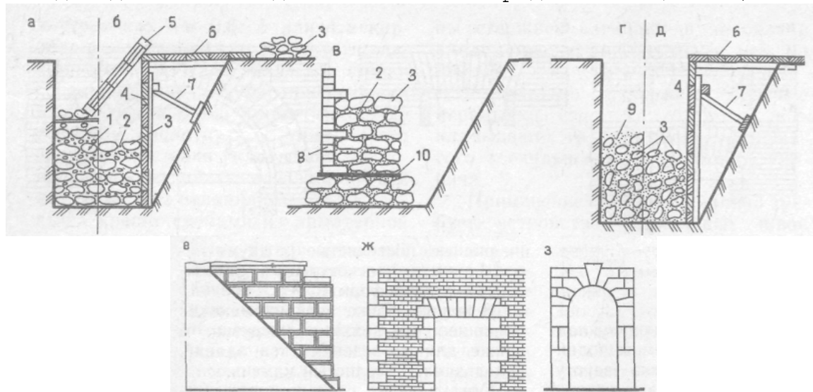
Рис. 8. Кладки из природных камней :
