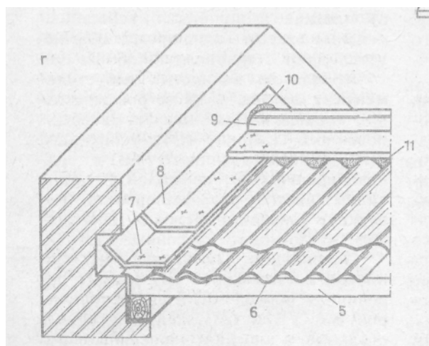
Рис. 1. Устройство кровель из асбестоцементных листов : а – раскладка со смещением листов; б – раскладка без смещения листов; в – покрытие ската листами ВО; г – продольное примыкание ската к стене; 1 и 2 – первый и второй листы первых рядов; 3 – второй лист последующего ряда; 4 – первый лист последующего ряда; 5 – брусок обрешетки; 6 – лист ВО; 7 – гвоздь; 8 – уголковая асбестоцементная деталь; 9 – коньковая асбестоцементная деталь; 10 – заделка раствором; 11 – заполнение мастикой.
