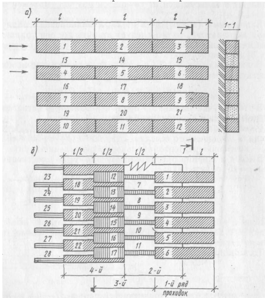
Рис. 3. Схема разработки грунта скреперами при планировке площадок: а – проходка через полосу; б – ребристо-шахматная проходка.
