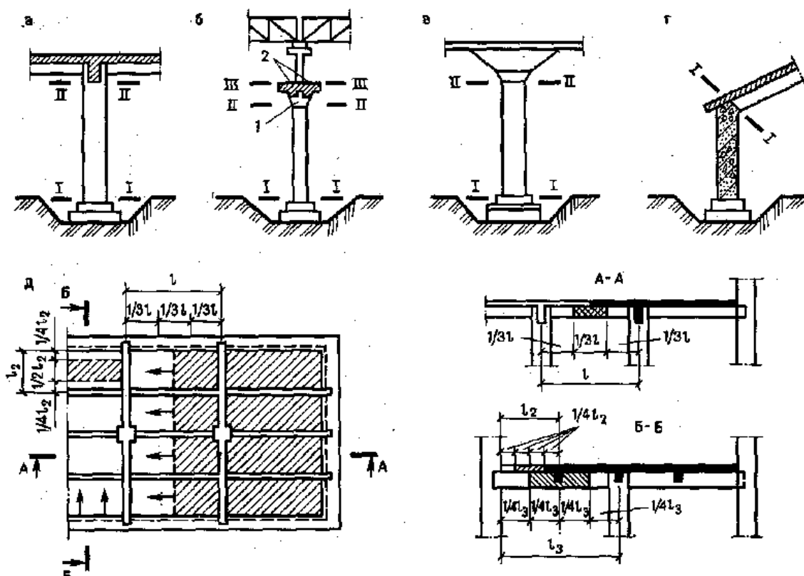
Рис. 1. Расположение рабочих швов при бетонировании : а — колонн и балок ребристого перекрытия; б — колонн с подкрановыми балками; в — колонн с безбалочным перекрытием; г — стойки и ригеля; д — перекрытия в направлении, параллельном второстепенным балкам и в направлении, перпендикулярном второстепенным балкам; I, II, III — положение рабочих швов; 1 — колонна; 2 — подкрановая балка.
