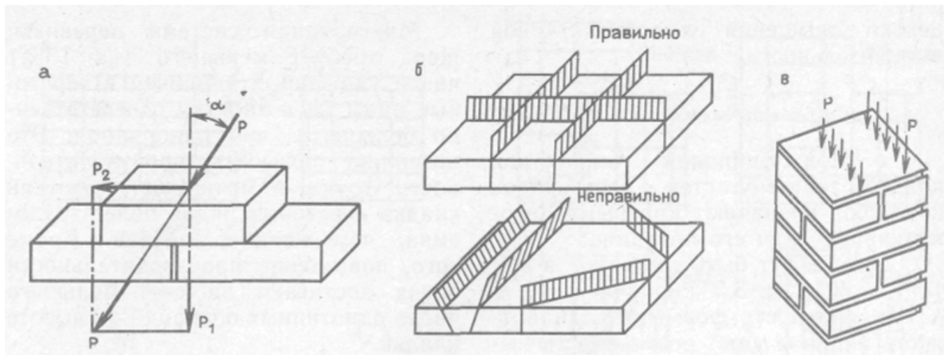
Рис. 2. Правила разрезки каменной кладки :
