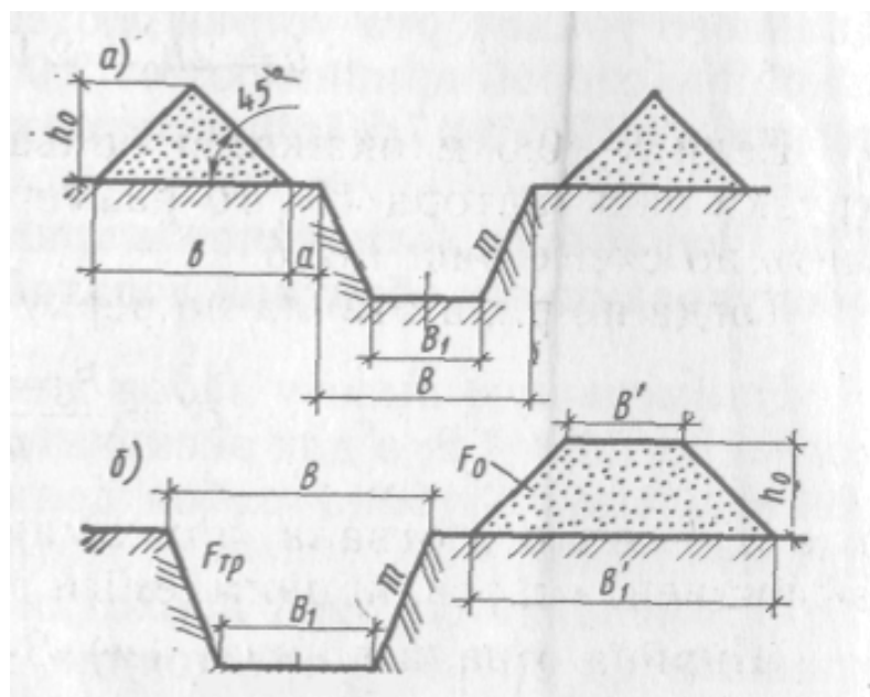
Рис. 3. Выемка и создаваемая при её разработке насыпь: а – при двустороннем отвале; б – при одностороннем.
