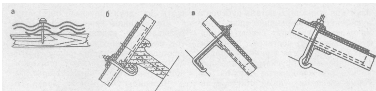
Рис. 2. Крепление асбестоцементных листов : а – к деревянной обрешетке; б – к железобетонным и стальным прогонам швеллерного и уголкового сечения.
