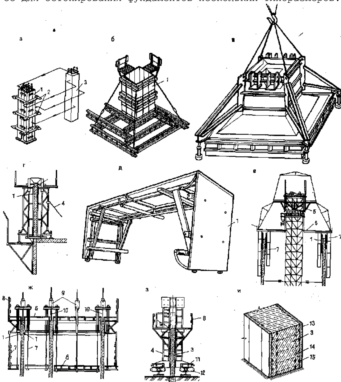
Рис. 1. Виды опалубки :
