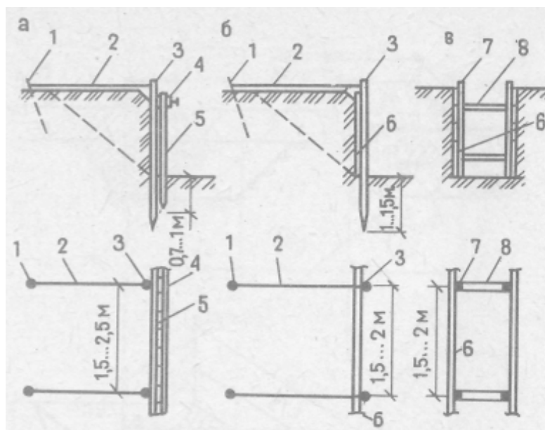
Рис. 5. Крепление стенок шпунтом (а), щитами с опорными стойками (б), щитами с опорными рамами: 1 – анкерная связь; 2 – оттяжка; 3 – опорная стойка; 4 – направляющая; 5 – шпунтовое ограждение; 6 – щиты; 7 – стойка распорной рамы; 8 – распорка.
