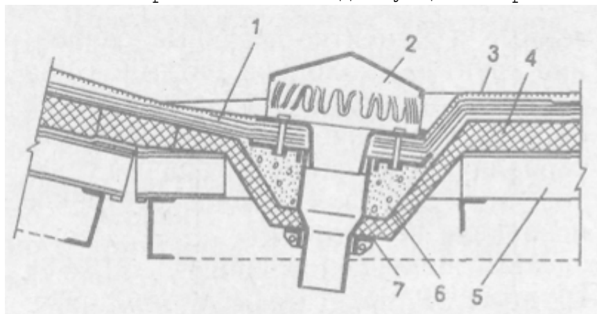
Рис. 2. Примыкание к воронкам внутренних водостоков : 1 – дополнительные слои кровельного материал; 2 – водоприемный колпак; 3 – защитный гидроизоляционный слой; 4 – теплоизоляционный материал; 5 – панель покрытия; 6 – цементно-песчаный раствор; 7 – стальной оцинкованный поддон.
