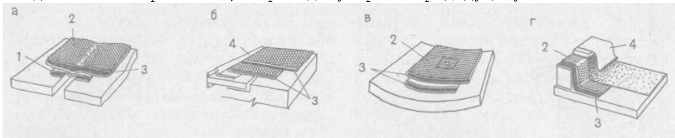
Рис. 5. Устройство мастичных кровель : а- над швами в стыках; б – на карнизах; в – в ендовах; г – в местах примыканий; 1 – компенсатор из пленки ПВХ; 2 – прокладки из стеклоткани; 3 – слой мастики; 4 – фартук из оцинкованной стали.
