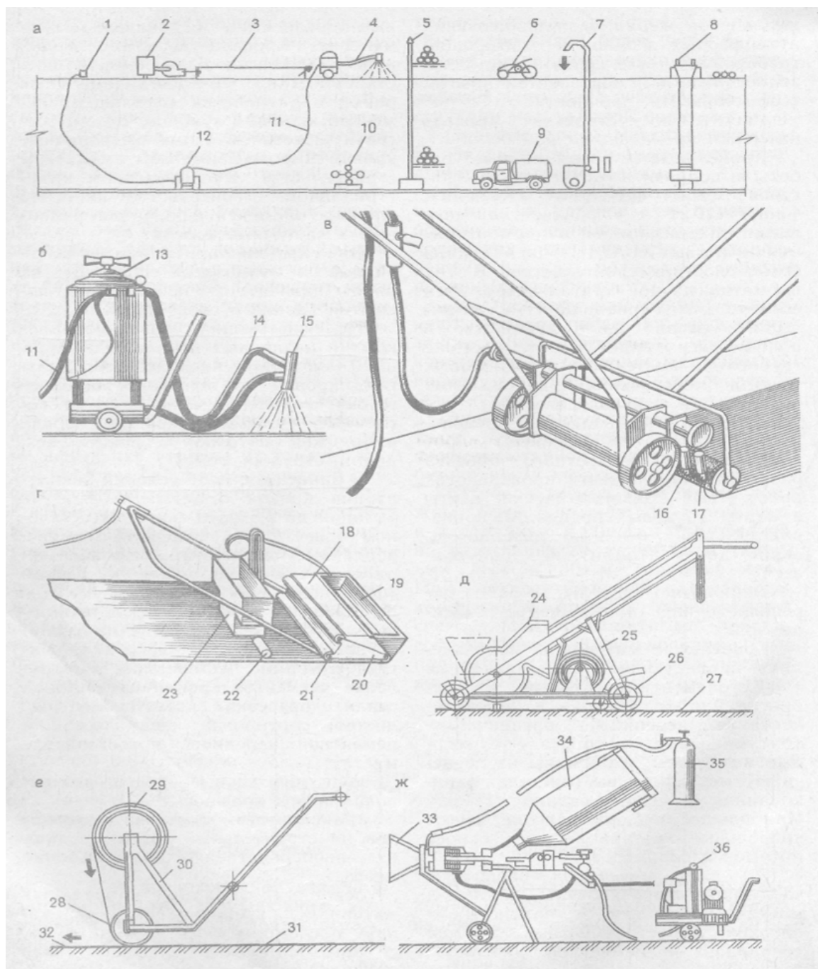
Рис. 1. Комплексная механизация при устройстве рулонных кровель : а — схема комплексной механизации; б — установка для нанесения грунтовки на основание; в — машина для наклеивания ковра из наплавляемого рубероида; г — машина, наносщая мастику на укладываемый рулон; д — машина, наносщая мастику на основание; е — каток-раскатчик; ж — газопламенная установка; 1 — чистка и обеспыливание поверхности основания сжатым воздухом; 2 — передвижной калорифер для просушки основания горячим воздухом; 3 — короб для продувки горячего воздуха; 4 — пистолет-распылитель для нанесения грунтовки на основание; 5 — подъемник; 6 — машина для наклейки рулона; 7 — стальной трубопровод для подачи мастики; 8 — элеватор для подачи гравия защитного слоя; 9 — автогудронатор; 10 — станок для очистки и перемотки рулонов; 11 — рукава для подачи воздуха; 12 — компрессор; 13 — нагнетательный бачок; 14 — рукав для подачи мастики; 15 — пистолет-распылитель; 16 — газовые горелки; 17 — рулон наплавляемого рубероида; 18 — полотнище рулонного материала; 19 — бачок со щелевым отверстием для прохода полотнища; 20 — валик с панцирной сеткой; 21 — вал для насадки рулона; 22 — колеса; 23 — бак для мастик; 24 — бак с мастикой; 25 — вал для насадки рулона; 26 — каток с резиновой обкладкой; 27 — накатанное полотнище; 28 — прижимной каток; 29 — полотнище, 32 — нанесенная мастика; 33 — загрузочный бачок; 35 — баллон со сжиженным газом; 36 — компрессор.
