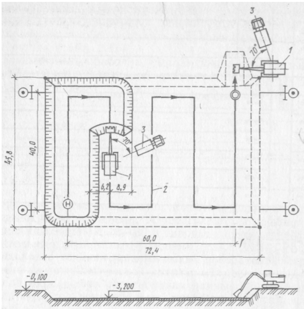
Рис. 8. Схема отрывки котлована одноковшовым экскаватором: 1 – экскаватор, оборудованный обратной лопатой, с объёмом ковша 0,5 \text{ м}^3 ; 2 – направление движения экскаватора; 3 – автосамосвал.
