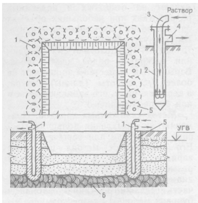
Рис. 6. Схема закрепления грунтов методом замораживания : 1 - колонка; 2 - наружная труба; 3 - питающая труба; 4 - патрубок для подсоединения к холодильной установке; 5 - замороженный грунт; 6 - водонепроницаемый грунт.
