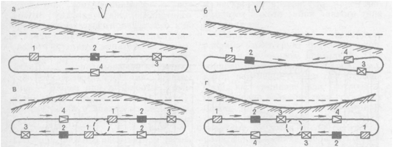
Рис. 2. Схема разработки грунта скреперами :
