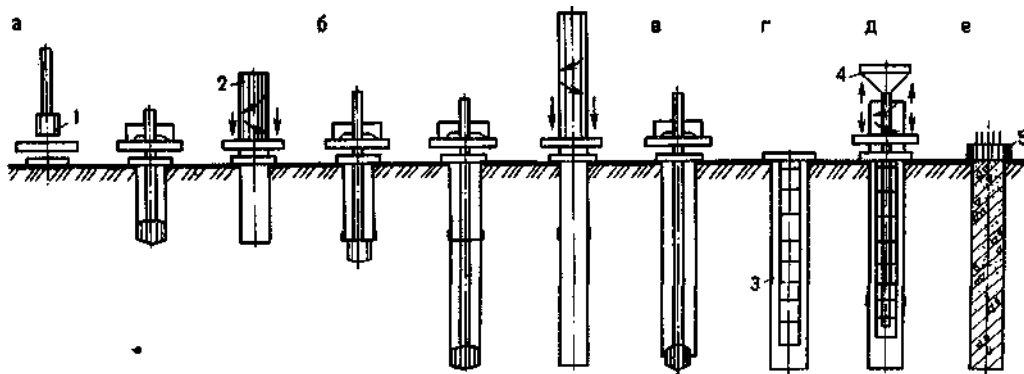
Рис. 2. Технологическая схема устройства буронабивных свай с применением обсадных труб : а — монтаж ротора и забуривание скважин с одновременным погружением обсадной трубы, б — проходка скважины, в — зачистка забоя скважины, г — установка арматурного каркаса, д — заполнение скважины бетонной смесью, извлечение обсадной трубы, е — формирование головы сваи в инвентарном кондукторе, 1 — роторная бурильная установка, 2 — обсадная труба, 3 — арматурный каркас, 4 — бетонолитная труба с приемным бункером, 5 — кондуктор
