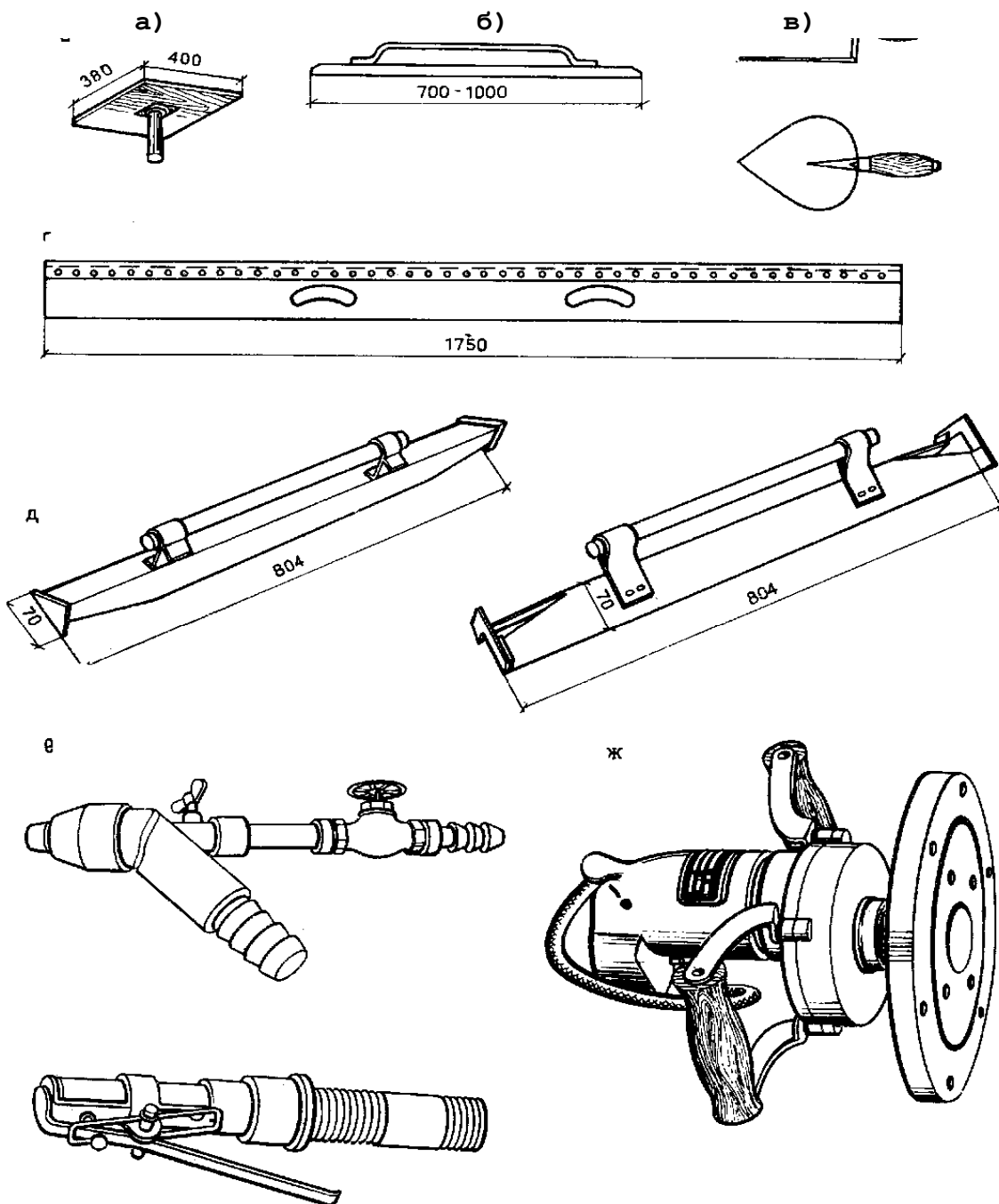
Рис. 2.2 - Основной инструмент и ручные машины для выполнения обычных штукатурок : а - сокол; б - полутёрка; в - мастерок; г - правило; д - лузговое и усеночное правило; е - форсунки пневматического и бескомпрессорного распыления; ж - затирочная ручная машина
