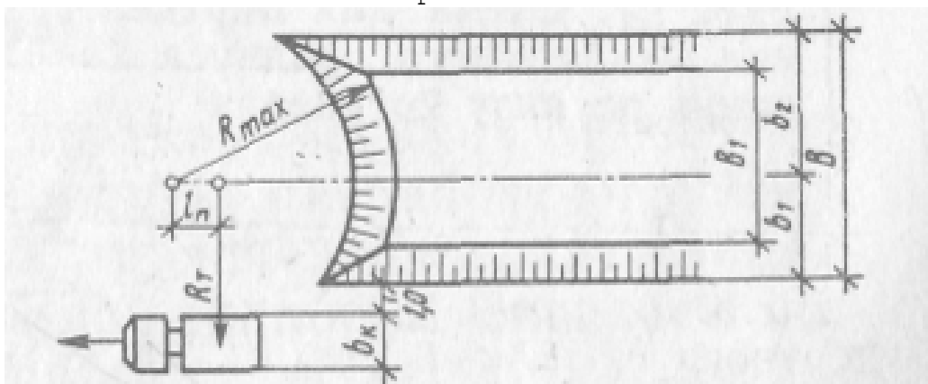
Рис. 7. Схема разработки грунта экскаватором обратная лопата при торцевой проходке
