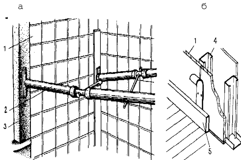
Рис. 2.4 – Устройство облицовки из листовых материалов: а – временное закрепление приклеиваемых листов или плит винтовыми упорами; б – схема установки облицовочных листов по металлическому каркасу перегородки; 1 – облицовочный лист; 2 – винтовой упор; 3 – прижимной брусок; 4 – стойка металлического каркаса; 5 – плинтус.
