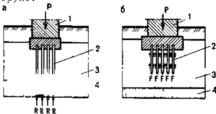
Рис. 1. Характер работы в грунте свай-стоек (а) и висячих свай (б): R - сила реакции от воздействия фундамента на грунт, F - сила трения поверхности свай о грунт; P - нагрузка; 1 - фундамент сооружения; 2 - свая; 3 - слабый грунт; 4 - прочный грунт
