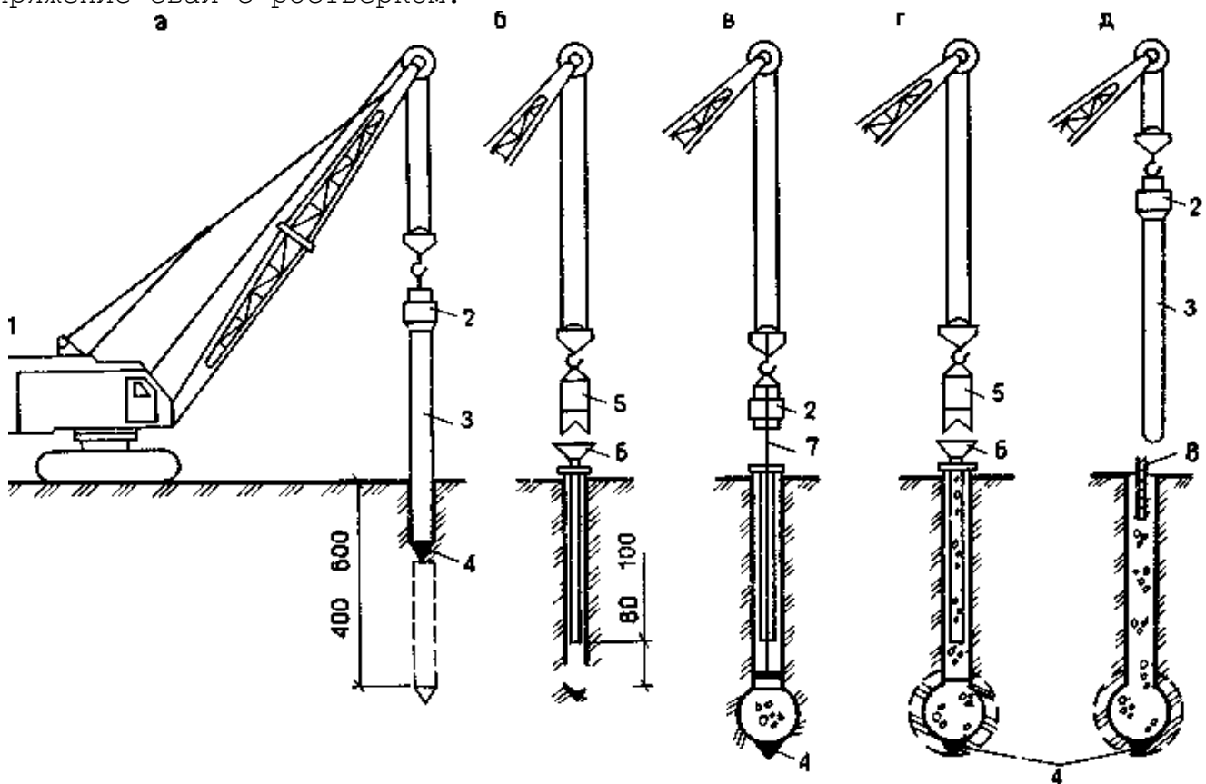
Рис. 4. Технологическая схема устройства вибротрамбованных свай : а - образование скважины; б - укладка первой порции бетонной смеси; в - уплотнение бетонной смеси трамбующей штангой, жестко соединенной с вибропогружателем; г - укладка и уплотнение последующих слоев бетонной смеси; д - извлечение обсадной трубы и установка арматурного каркаса в голове сваи; 1 - кран; 2 - вибропогружатель; 3 - обсадная труба; 4 - съемный башмак; 5 - загрузочный бункер; 6 - бетонолитная труба с приемной воронкой; 7 - трамбующая штанга; 8 - арматурный каркас
