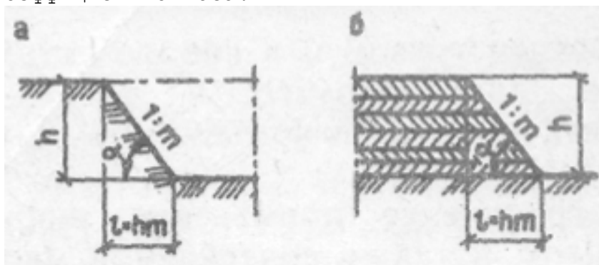
Рис. 4. Элементы откосов: а - выемки; б - насыпи.
