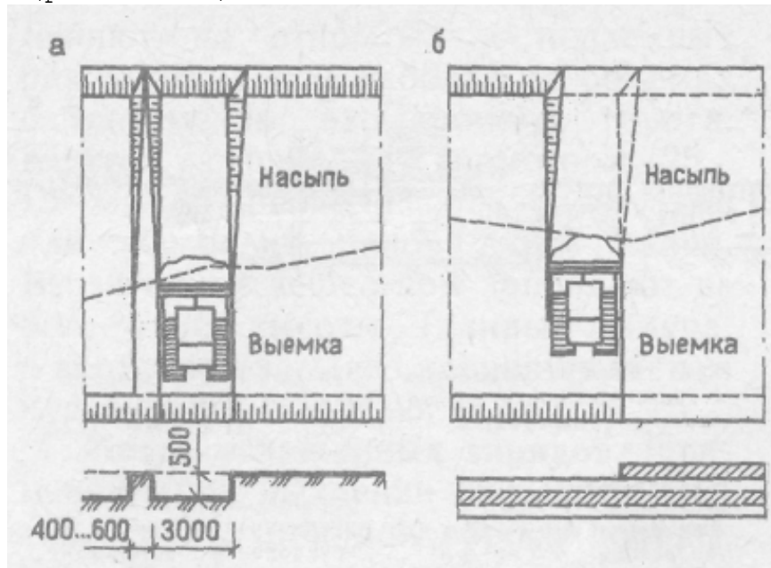
Рис. 4. Схемы разработки грунта бульдозерами : а - траншейным способом; б - послойным способом.
