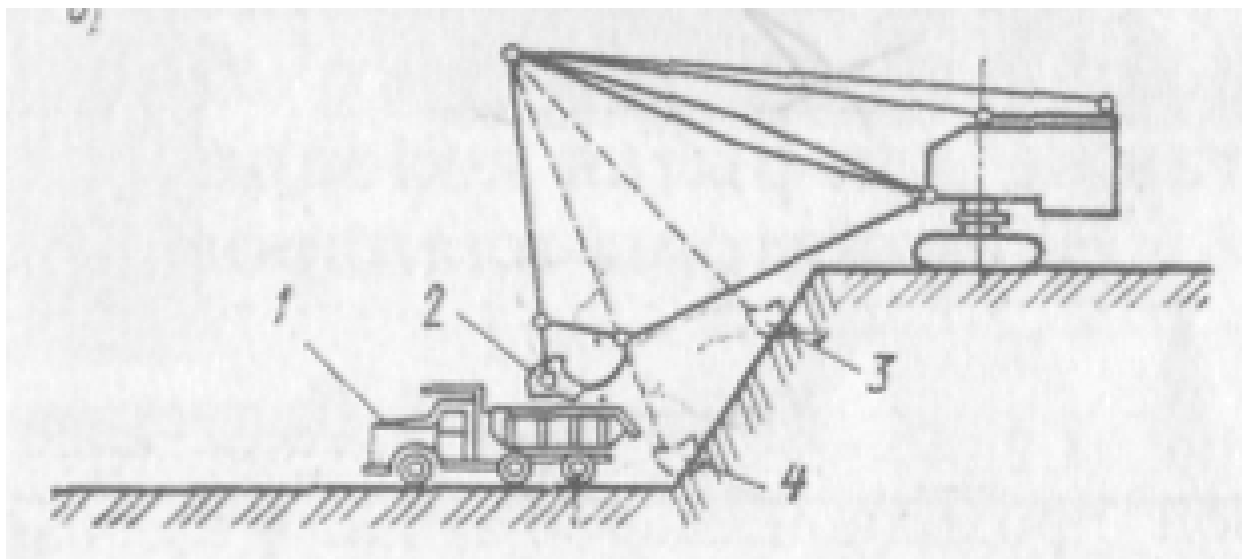
Рис. 10. Схема разработки и погрузки грунта экскаватором драглайн: 1 – автосамосвал; 2 – разгрузка ковша; 3 – окончание набора и подъем ковша; 4 – опускание ковша и набор грунта.
