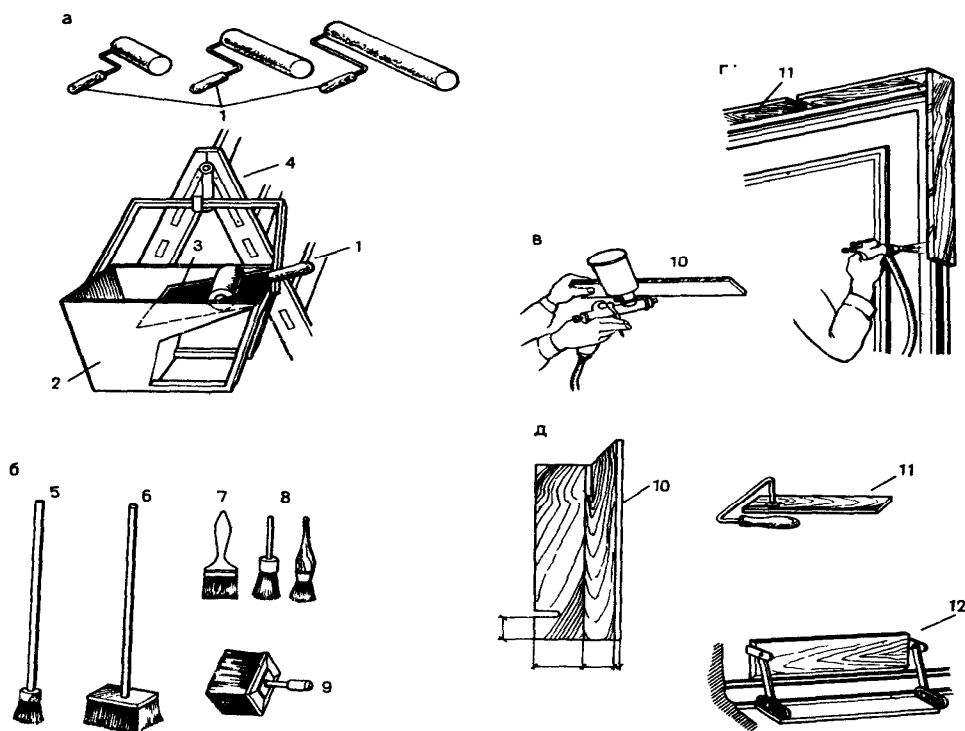
Рис. 1.4. Инструмент и приспособления для окрашивания поверхностей вручную
