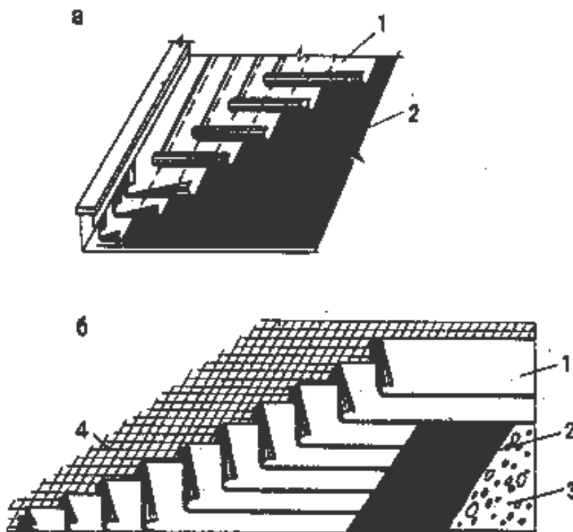
Рис. 3. Наклеивание полотнищ рулонного ковра послойно (а) и одновременно (б): 1 – полотнище; 2 – мастика; 3 – подсыпка из гравия; 4 – огрунтованное основание.
