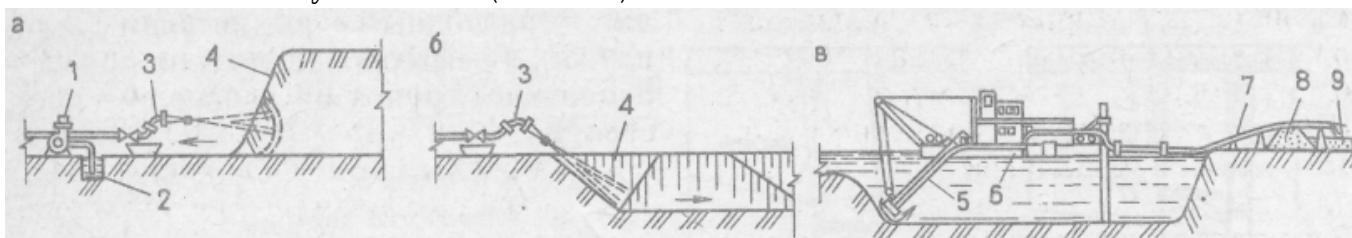
Рис. 1. Схемы разработки грунта гидромеханическим способом :
