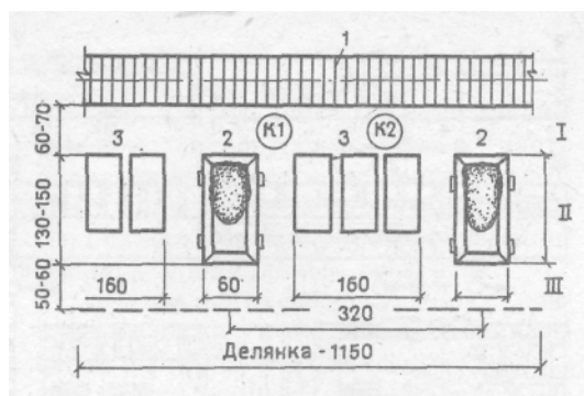
Рис. 2. Схема организации рабочего места звена каменщиков : I – рабочая зона; II – зона материалов, III – вспомогательная зона; 1 – выкладываемая стена; 2 – ящики с раствором; 3 – пакеты кирпича; К1, К2 – размещение каменщиков.
