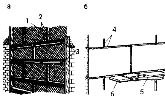
Рис. 2.9 - Расшивка рустов : а - рейками; б - наградкой; 1 - грунт; 2 - спаренные рейки; 3 - распорки; 4 - шов, выбранный наградкой; 5 - наградка; 6 - правило.
