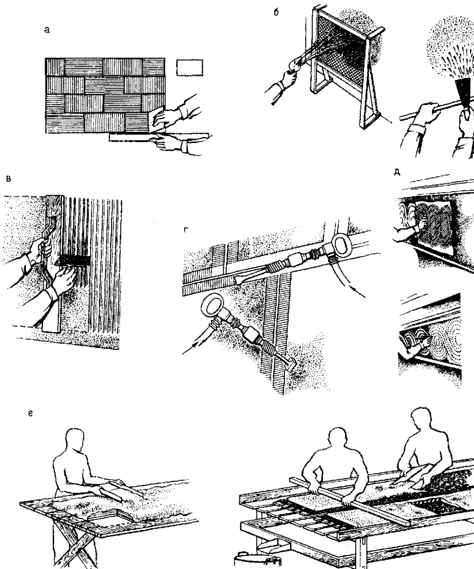
Рис. 2.5 - Создание фактуры и текстуры декоративных штукатурок : а - обработка циклей; б - набрызг с метелки через сетку; в - накатка фигурным валиком; г - обработка руста бучардой и борозд скампелью; д - перенос контура рисунка через перфорированный трафарет и проработка рисунка резцом при выполнении сграффито; е - подготовка декоративного слоя полированного искусственного мрамора.
