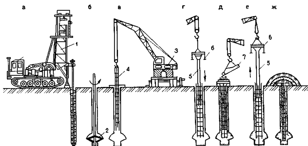
Рис. 1. Технологическая схема устройства буронабивных свай сухим способом : а – бурение скважины; б – устройство уширенной полости; в – установка арматурного каркаса; г – установка бетонолитной трубы с вибробункером; д – заполнение вибробункера бетонной смесью; е – бетонирование скважины методом вертикального перемещения трубы; ж – утепление оголовка сваи, в зимних условиях; 1 – шнековая буровая установка; 2 – расширитель; 3 – кран грузоподъемностью 10... 12 т; 4 – арматурный каркас; 5 – бетонолитная труба; 6 – вибробункер; 7 – загрузочный бункер
