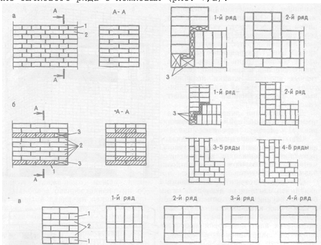
Рис. 3. Системы перевязки швов кладки : а – однорядная; б – многорядная; в – трёхрядная; 1 – тычковый ряд; 2 – ложковый ряд; 3 – неполные кирпичи.
