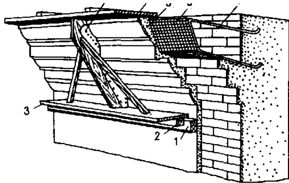
Рис. 2.6 - Вытягивание карниза : 1 - направляющие бруски; 2 - ползок; 3 - салазки; 4 - профильная доска; 5 - штукатурный намет; 6 - металлическая сетка; 7 - металлический каркас
