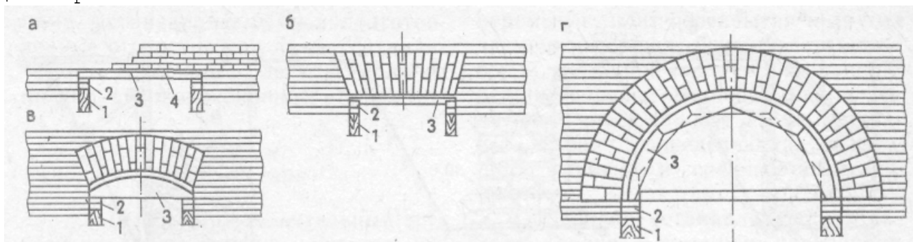
Рис. 7. Кладка перемычек из кирпича : а - рядовых; б - клинчатых; в - лучковых; г - арочных; 1 - стойка; 2 - клинья; 3 - опалубка; 4 - арматура.
