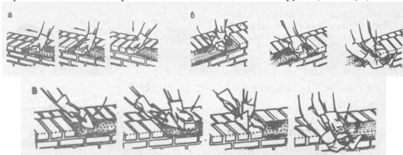
Рис. 5. Укладка тычкового ряда наружной версты «вприсык» (а), «вприсык с подрезкой» (б) и «вприжим» (в).
