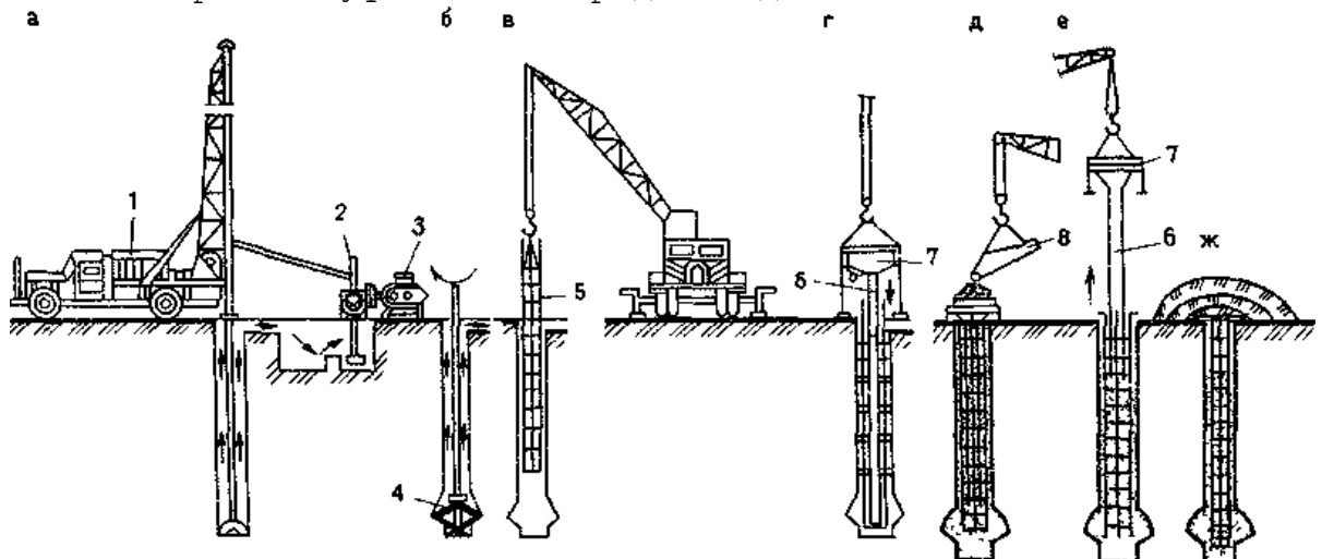
Рис. 3. Технологическая схема устройства буронабивных свай под глинистым раствором : а — бурение скважины; б — устройство уширенной полости; в — установка арматурного каркаса; г — установка бетонолитной трубы с вибробункером; д — заполнение вибробункера бетонной смесью; е — бетонирование методом ВПТ; ж — утепление оголовка сваи в зимних условиях; 7 — буровая установка; 2 — глиносмеситель; 3 — насос; 4 — расширитель, 5 — арматурный каркас; 6 — бетонолитная труба; 7 — приемный бункер; 8 — загрузочный бункер
