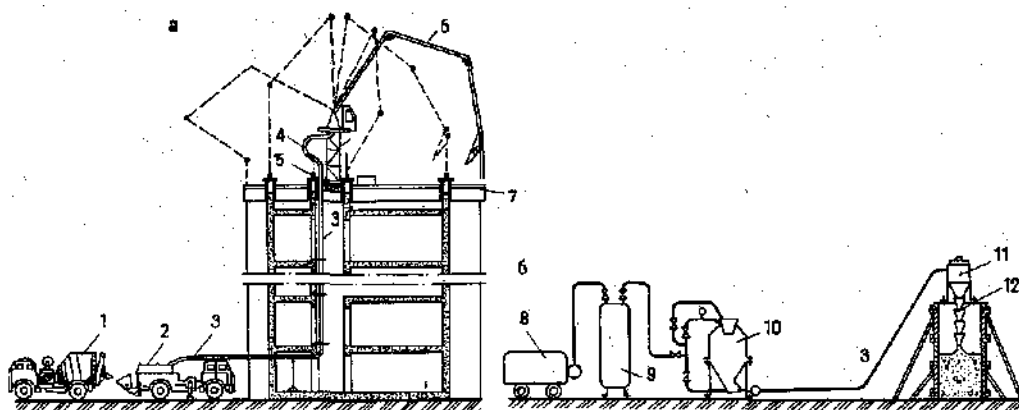
Рис. 2. Схема подачи бетонной смеси с помощью автобетононасоса (а) и пневматического нагнетателя (б) : 1 – автобетоносмеситель; 2 – автобетононасос; 3 – бетоновод; 4 – рукав (компенсатор длины бетоновода); 5 – постамент с полноповоротной платформой; 6 – распределительная стрела; 7 – скользящая опалубка; 8 – компрессор; 9 – ресивер; 10 – пневмонагнетатель; 11 – гаситель; 12 – хобот; (пунктиром даны положения стрелы).
