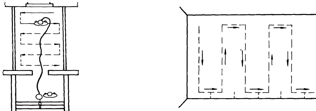
Рис. 1.3. Схема перемещения краскораспылителя при окрашивании поверхности с помощью пневматической и гидродинамической установок высокого давления
