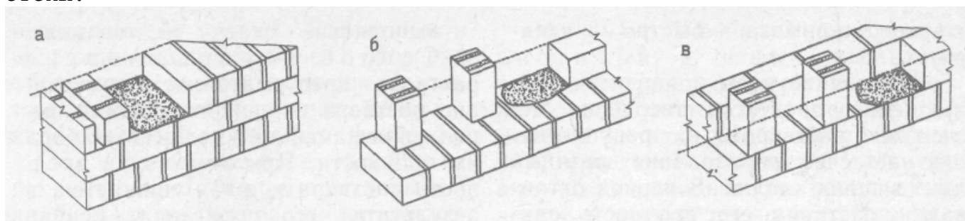
Рис. 6. Выполнение кладки из мелких блоков : а — тычкового ряда; б — ложкового ряда наружной версты; в — то же, внутренней версты.
