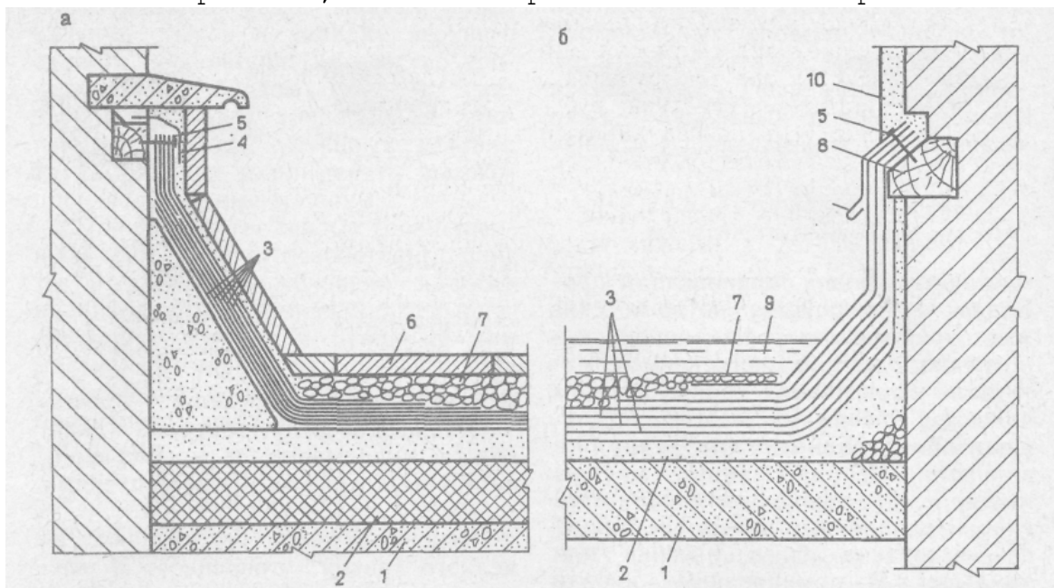
Рис. 4. Устройство плоских эксплуатируемых (а) и водонаполненных (б) кровель : 1 - железобетонная плита; 2 - стяжка; 3 - кровельный ковер; 4 - фартук из стали; 5 - кровельный гвоздь; 6 - бетонные плиты; 7 - дренарующий слой из гравия; 8 - закладная рейка; 9 - слой воды; 10 - заделка раствором.
