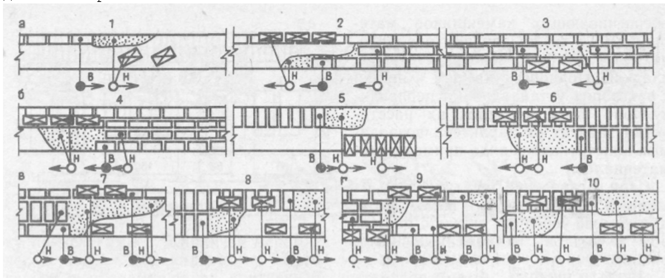
Рис. 1. Схема работы звеньев каменщиков :
