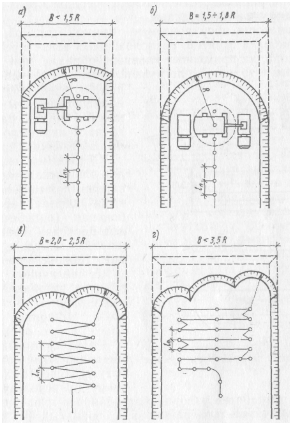
Рис. 2. Разработка грунта экскаватором прямой лопата: а – лобовая проходка с односторонней погрузкой грунта в автосамосвалы; б – то же, с двусторонней погрузкой; в – то же, с перемещением экскаватора по зигзагу; г – уширенная проходка с перемещением экскаватора поперек котлована
