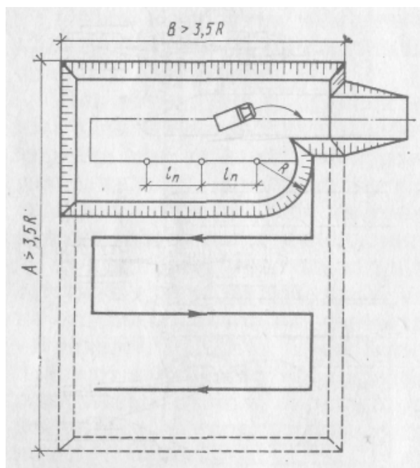
Рис. 3. Разработка котлована боковой проходкой экскаватором прямая лопата
