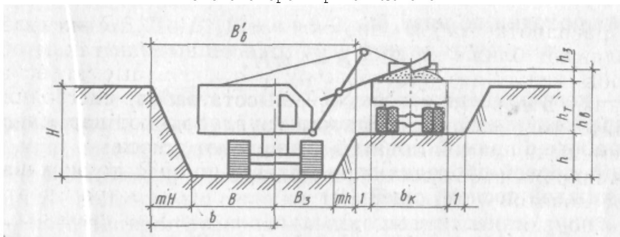
Рис. 4. Разработка котлована экскаватором прямая лопата параллельными боковыми проходками.
