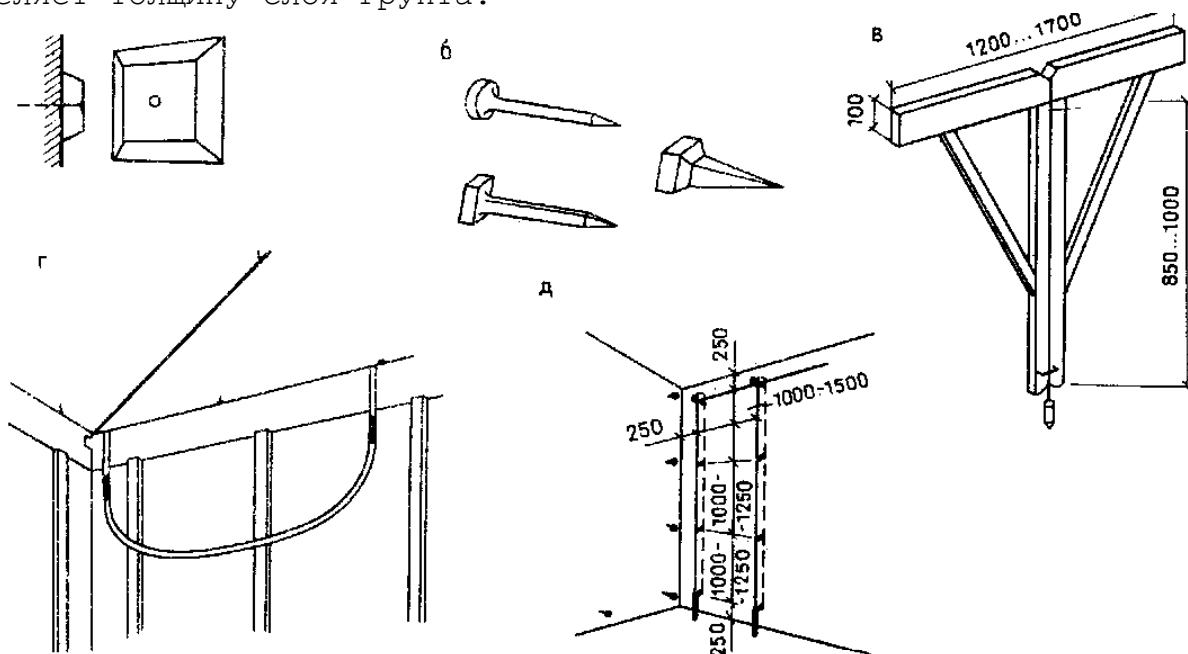
Рис. 2.3 - Марки и приспособления для их установки : а - марка из раствора; б - инвентарные марки; в - ватерпас для установки и проверки положения марок на потолках; г - водяной уровень для установки и проверки положения марок на потолках; д - схема установки марок на стенах
