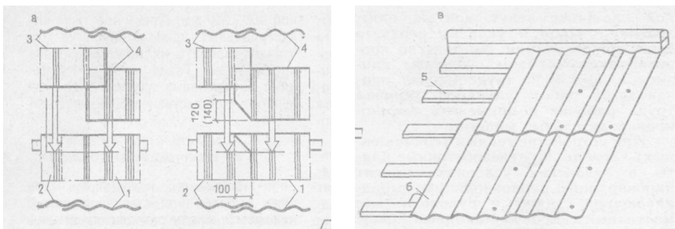
Рис. 1. Устройство кровель из асбестоцементных листов : а – раскладка со смещением листов; б – раскладка без смещения листов; в – покрытие ската листами ВО; г – продольное примыкание ската к стене; 1 и 2 – первый и второй листы первых рядов; 3 – второй лист последующего ряда; 4 – первый лист последующего ряда; 5 – брусок обрешетки; 6 – лист ВО; 7 – гвоздь; 8 – уголковая асбестоцементная деталь; 9 – коньковая асбестоцементная деталь; 10 – заделка раствором; 11 – заполнение мастикой.
