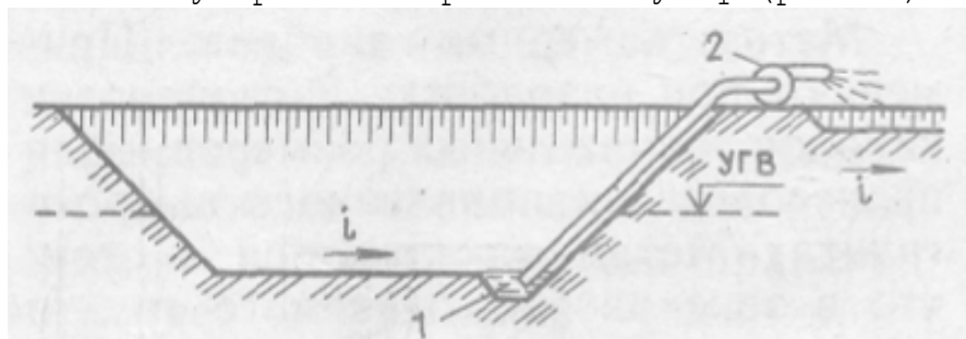
Рис. 7. Схема открытого водоотлива из котлована : 1 - зумпф; 2 - центробежный насос.
