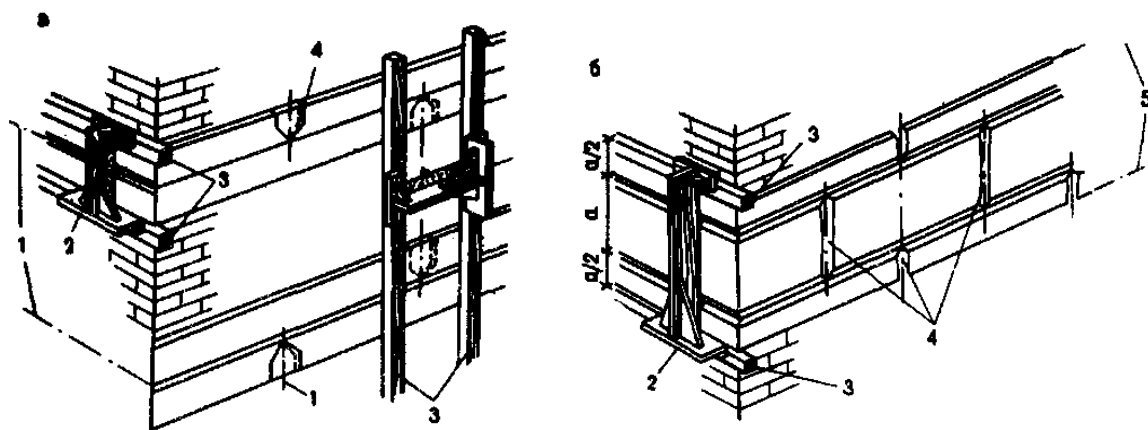
Рис. 2.8 – Вытягивание контура рустов :
